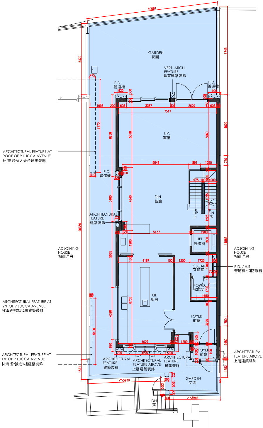
G/F FLOOR PLAN 地下樓面平面圖
