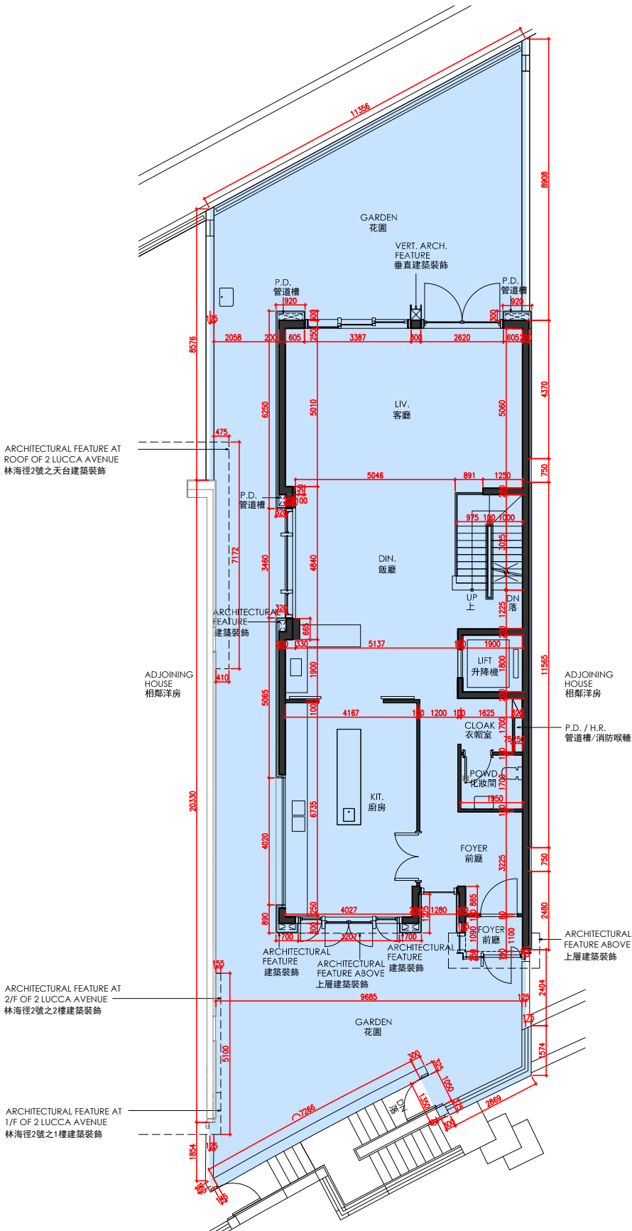
G/F FLOOR PLAN 地下樓面平面圖
