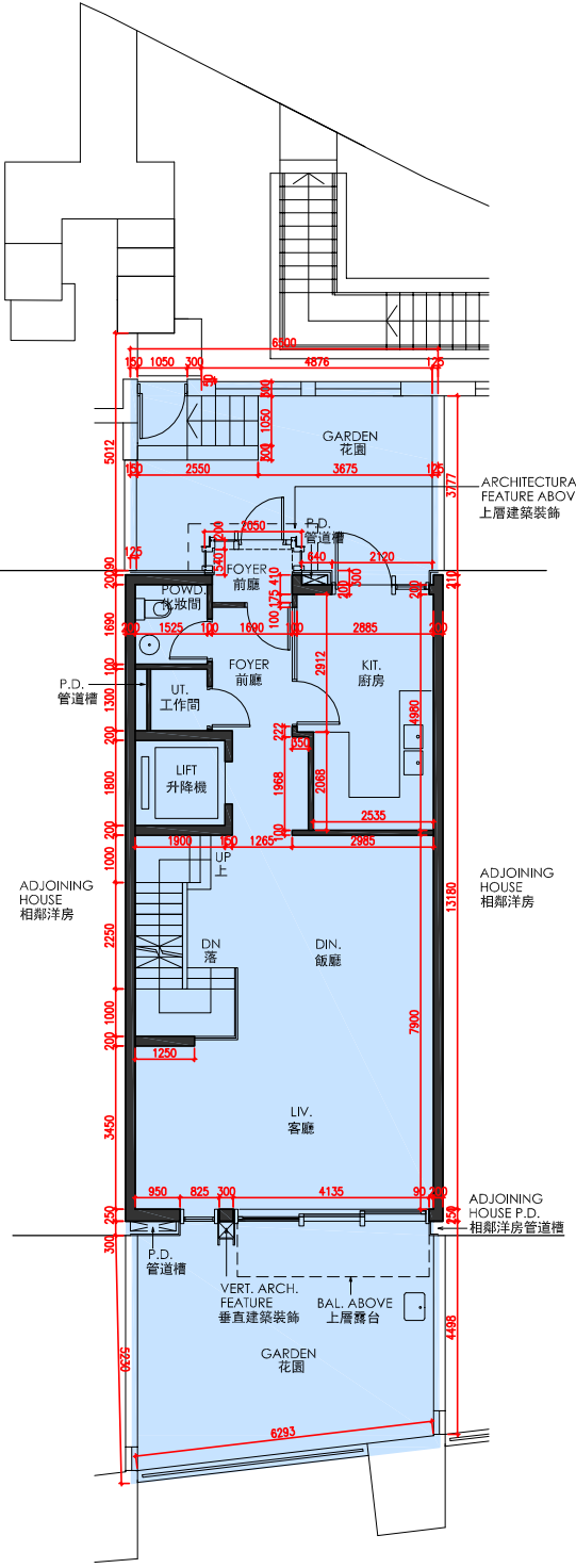
G/F FLOOR PLAN 地下樓面平面圖
