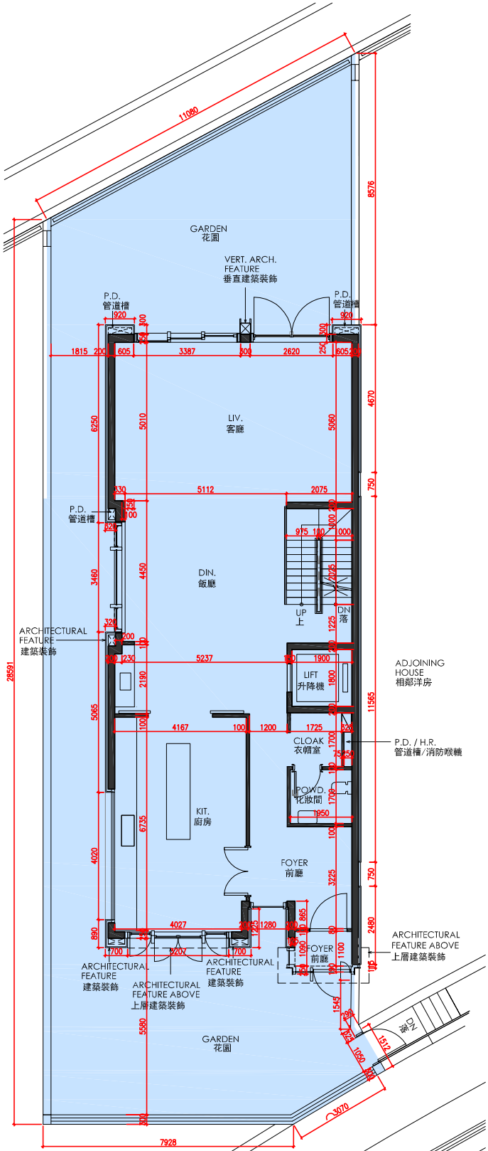
G/F FLOOR PLAN 地下樓面平面圖
