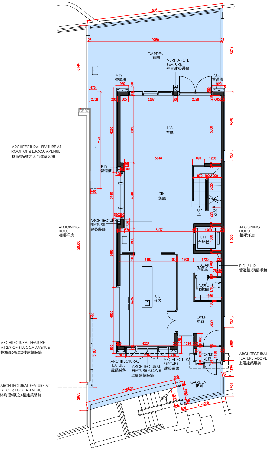
G/F FLOOR PLAN 地下樓面平面圖
