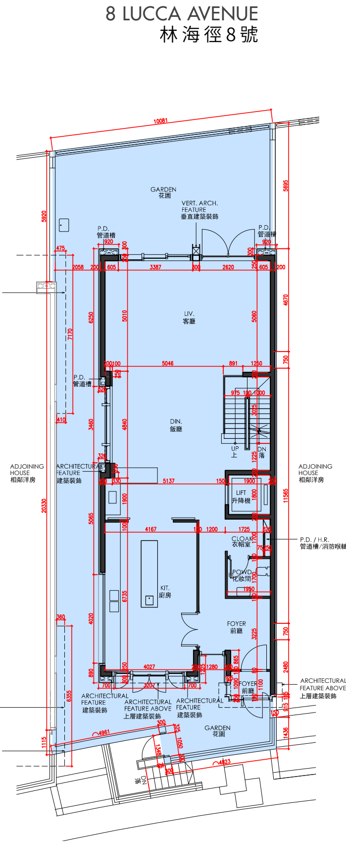
G/F FLOOR PLAN 地下樓面平面圖
