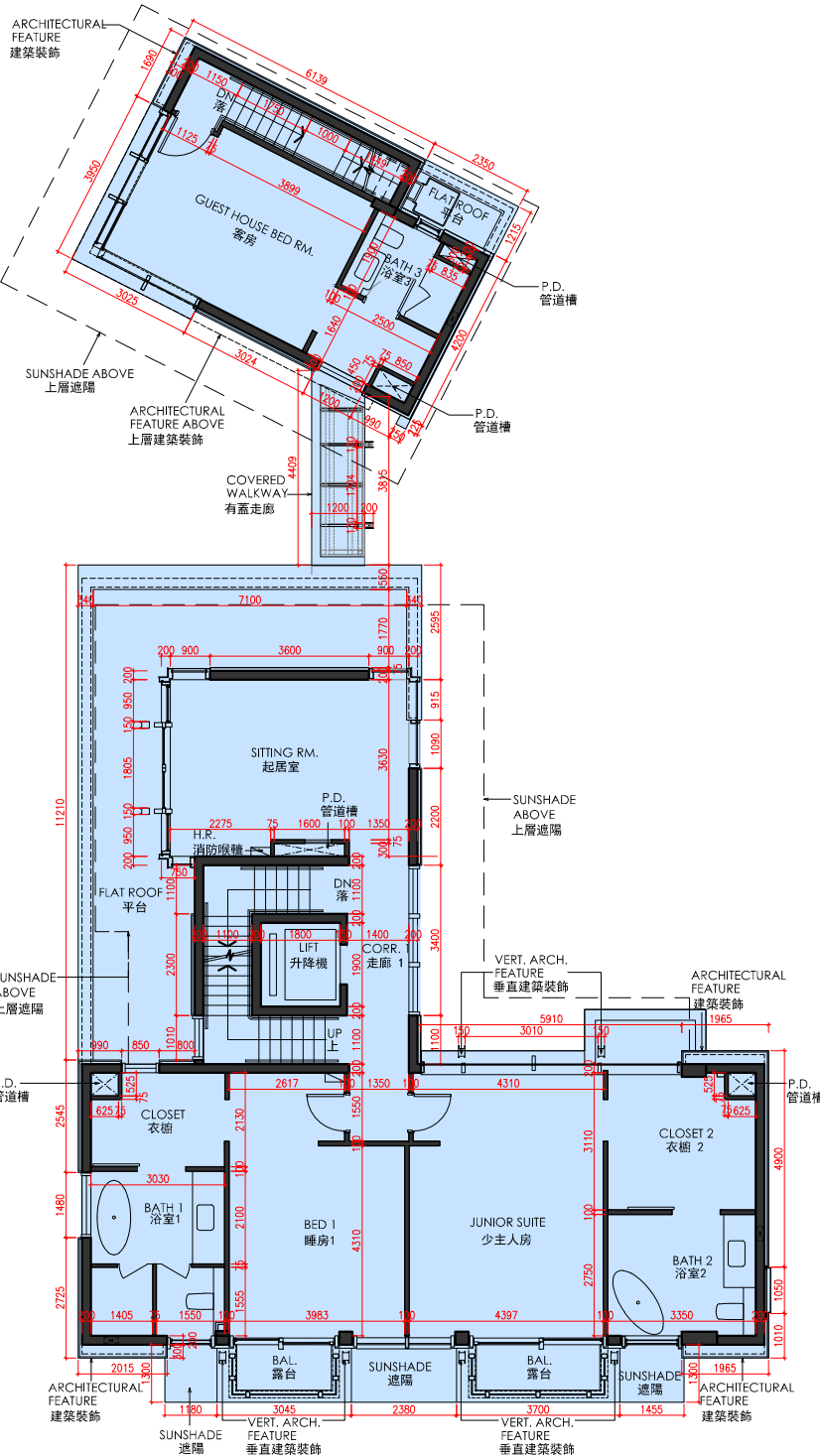
1/F FLOOR PLAN 1樓樓面平面圖
