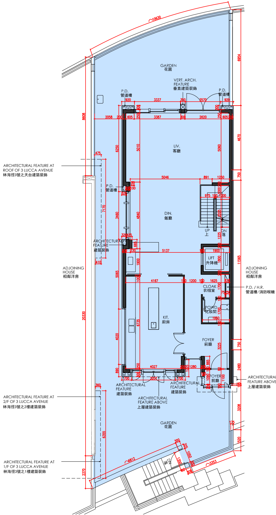
G/F FLOOR PLAN 地下樓面平面圖
