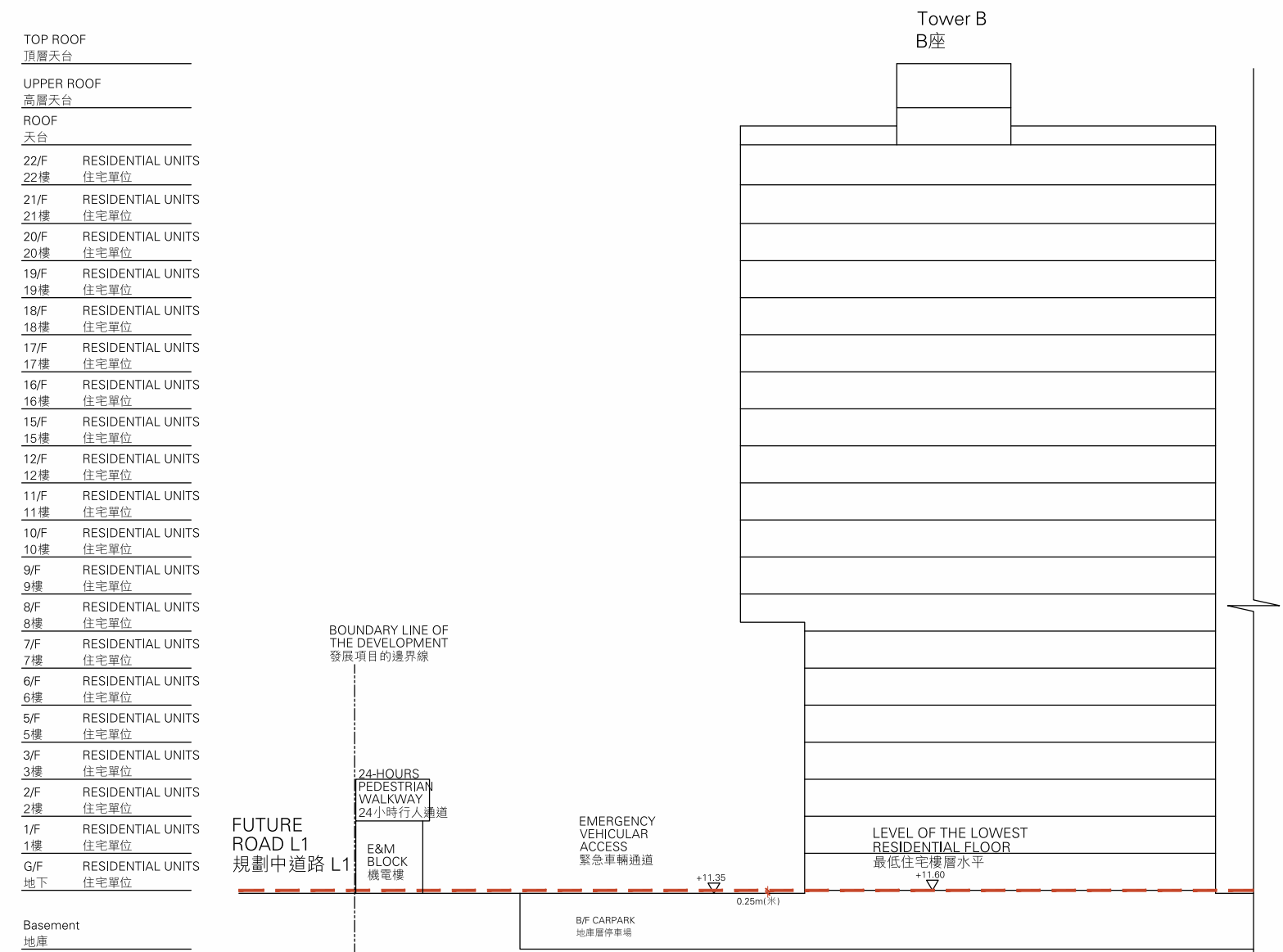
橫截面圖 C-C CROSS-SECTION PLAN C-C
