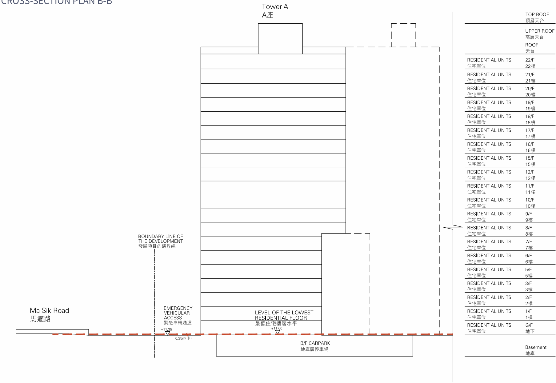
橫截面圖 B-B CROSS-SECTION PLAN B-B
