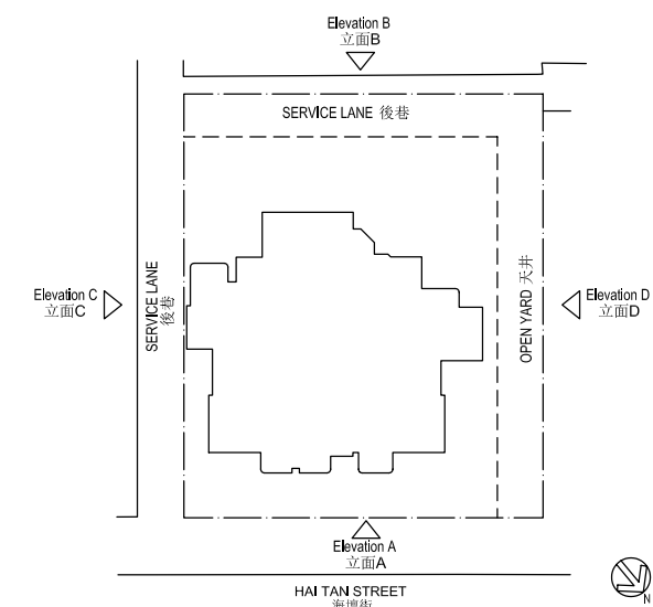
BLOCK PLAN 座向圖
