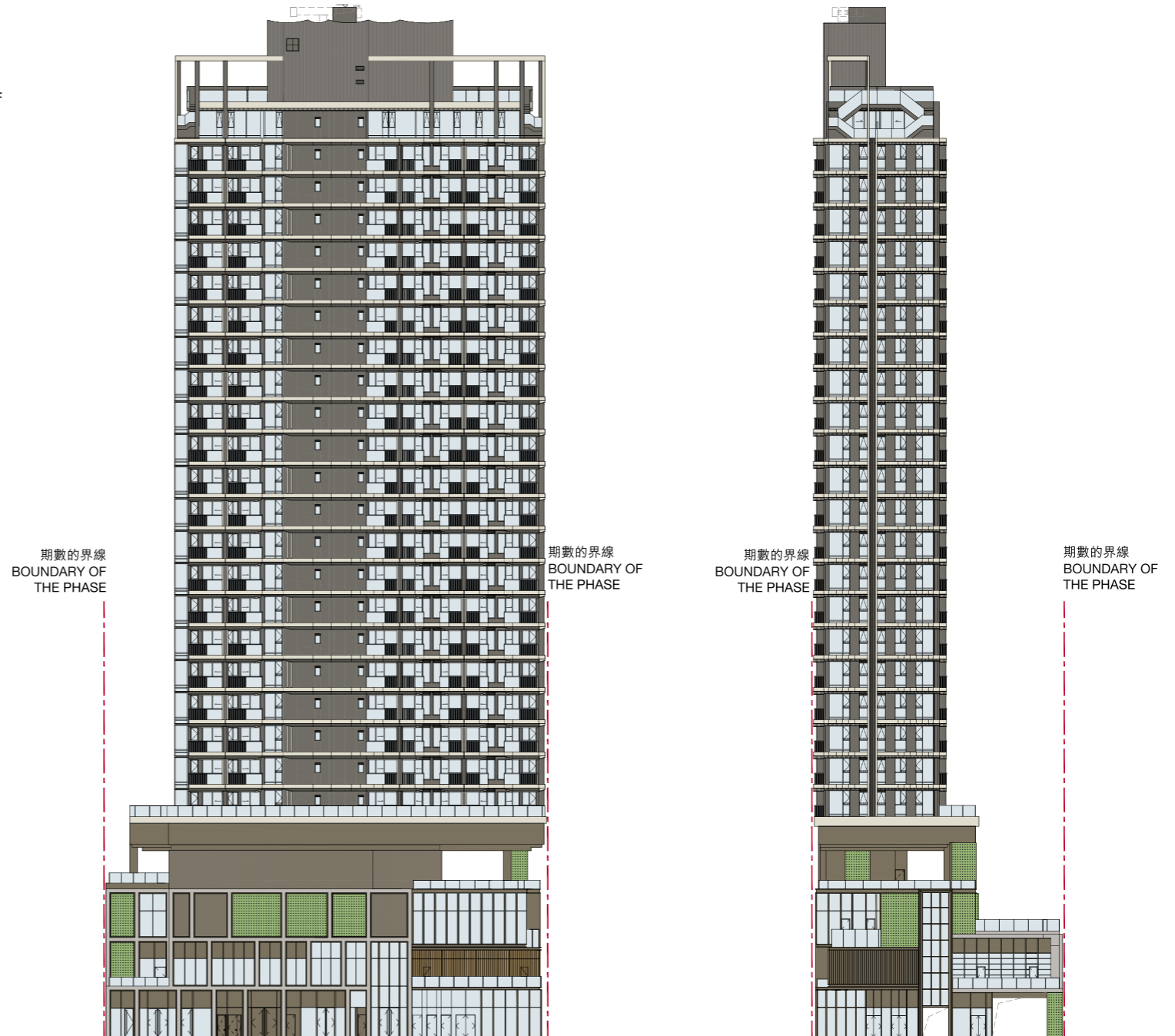
立面圖 C ELEVATION PLAN C
