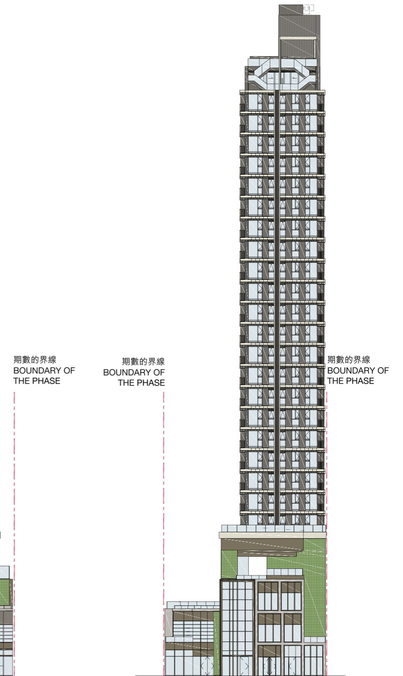
立面圖 B ELEVATION PLAN B
