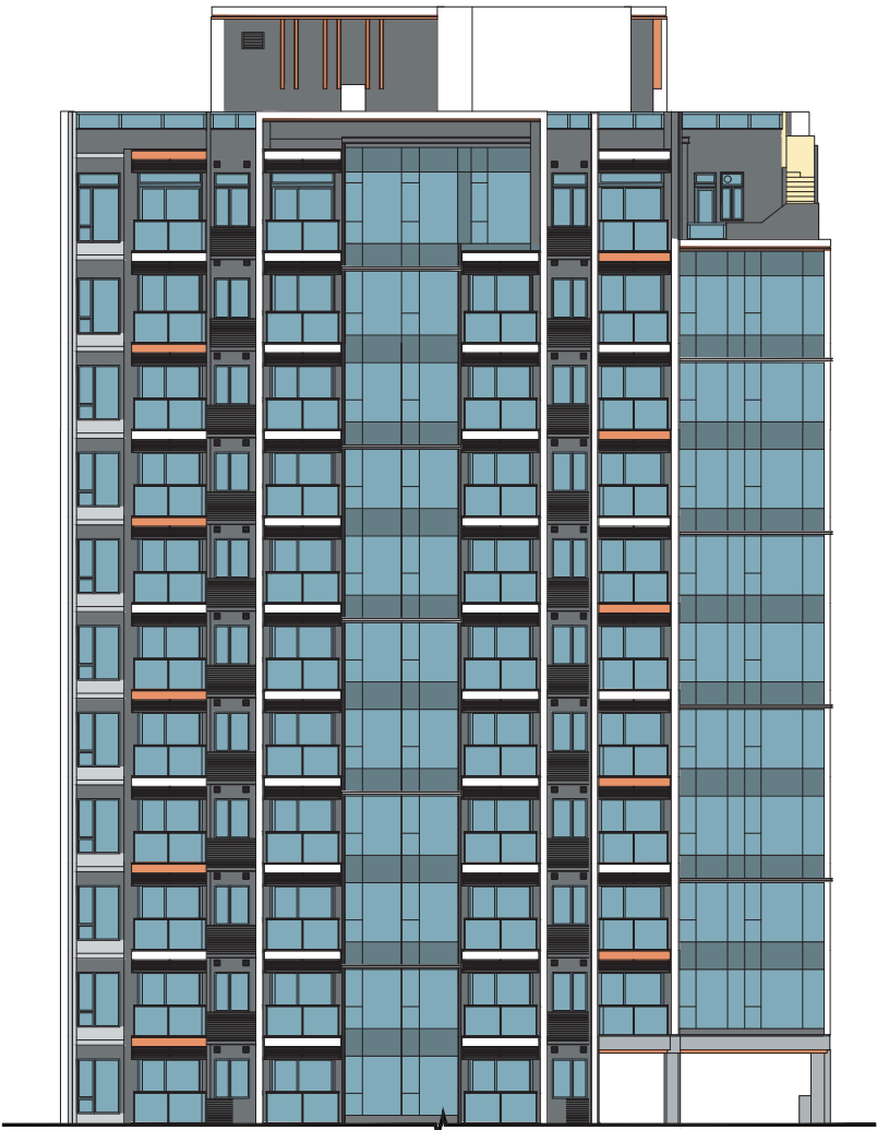
ELEVATION 4 立面 4
