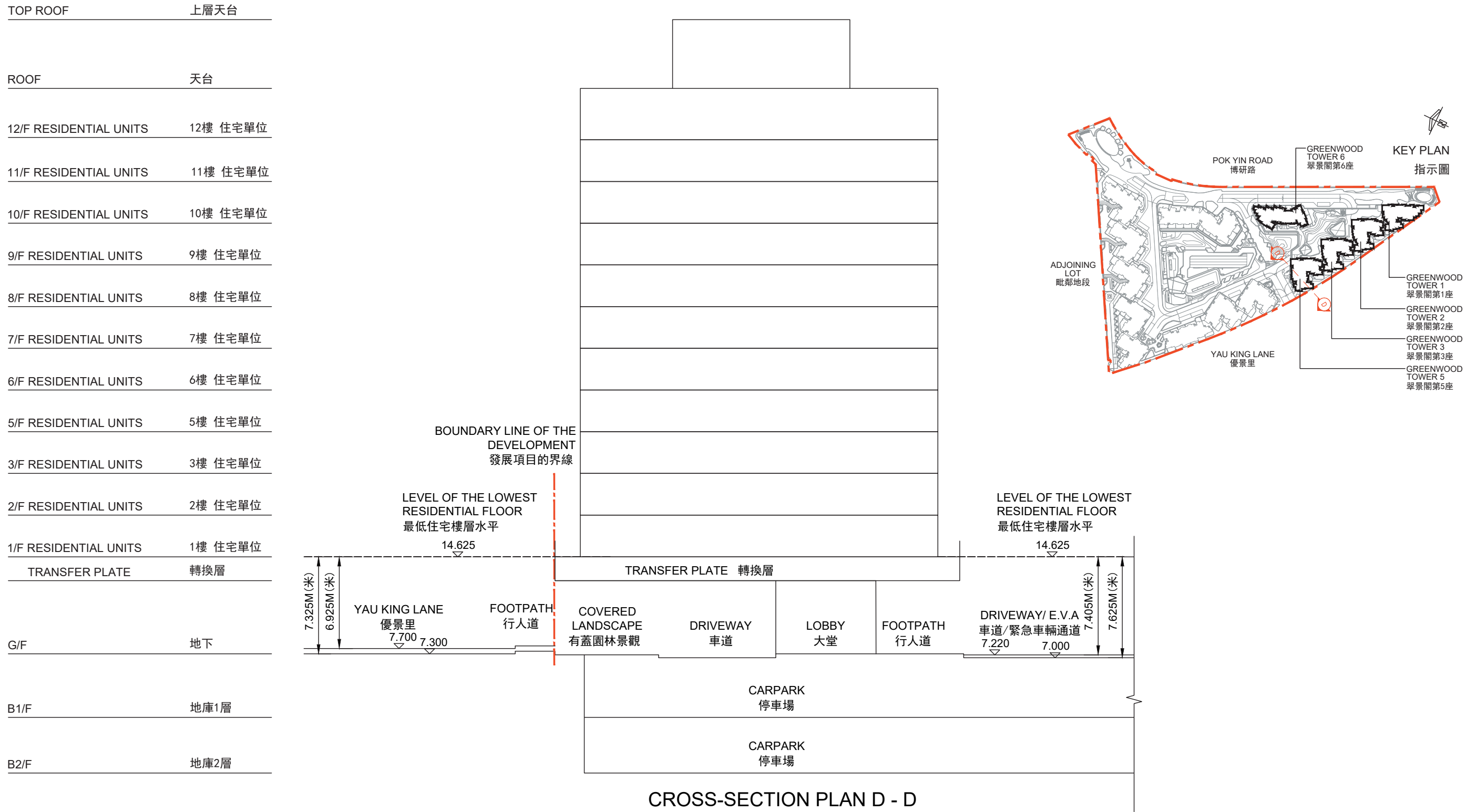
GREENWOOD TOWER 5 翠景閣第5座
