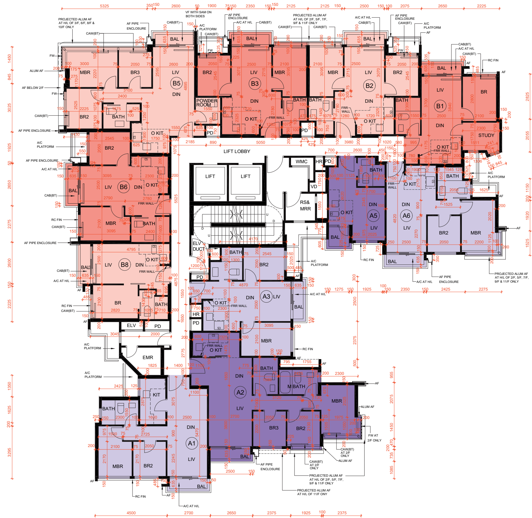
GREENWOOD TOWER 2 2/F-3/F AND 5/F-11/F FLOOR PLAN 翠景閣第2座 2樓至3樓 及 5樓至11樓平面圖
