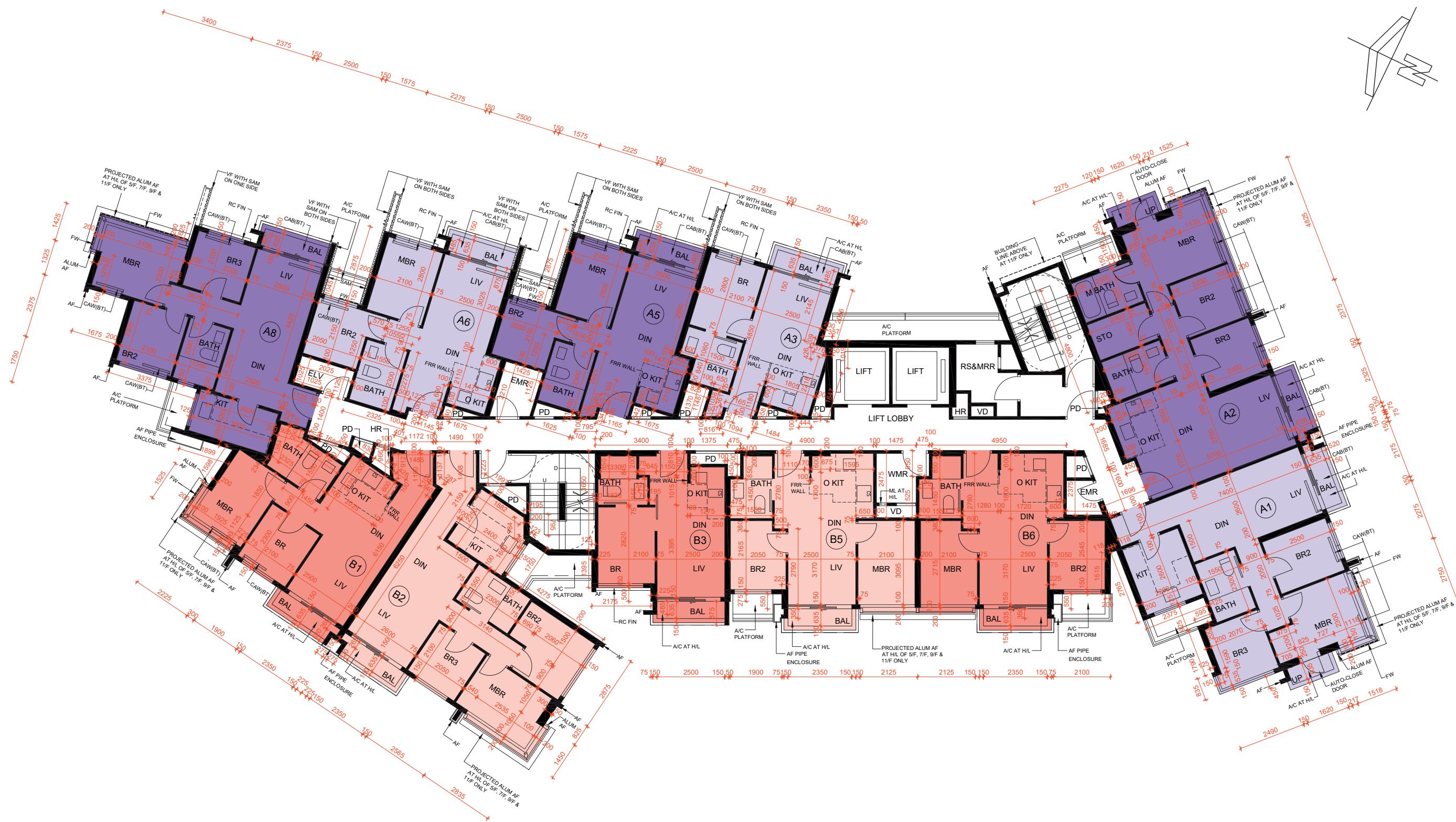
GREENWOOD TOWER 6 3/F AND 5/F-11/F FLOOR PLAN 翠景閣第6座 3樓 及 5樓至11樓平面圖
