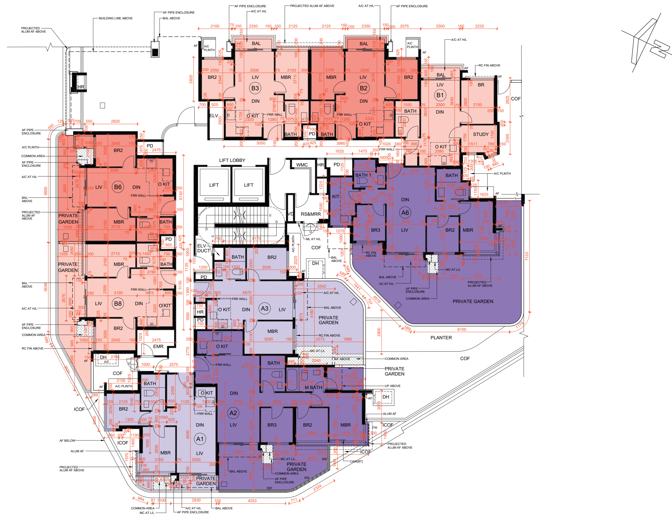
GREENWOOD TOWER 5 1/F FLOOR PLAN 翠景閣第5座 1樓平面圖
