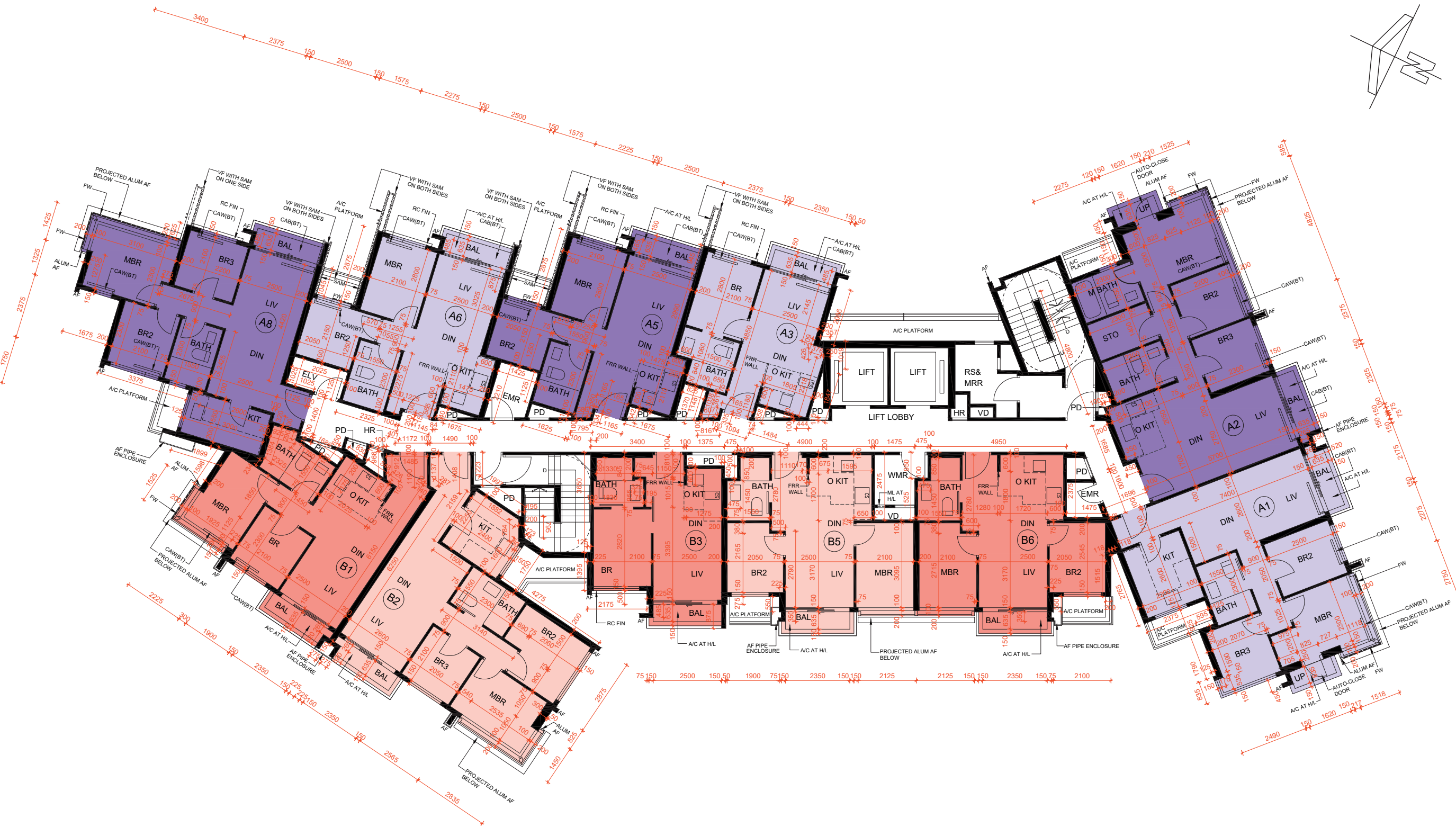
GREENWOOD TOWER 6 12/F FLOOR PLAN 翠景閣第6座 12樓平面圖
