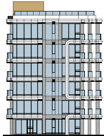
Elevation 2 立面圖2
