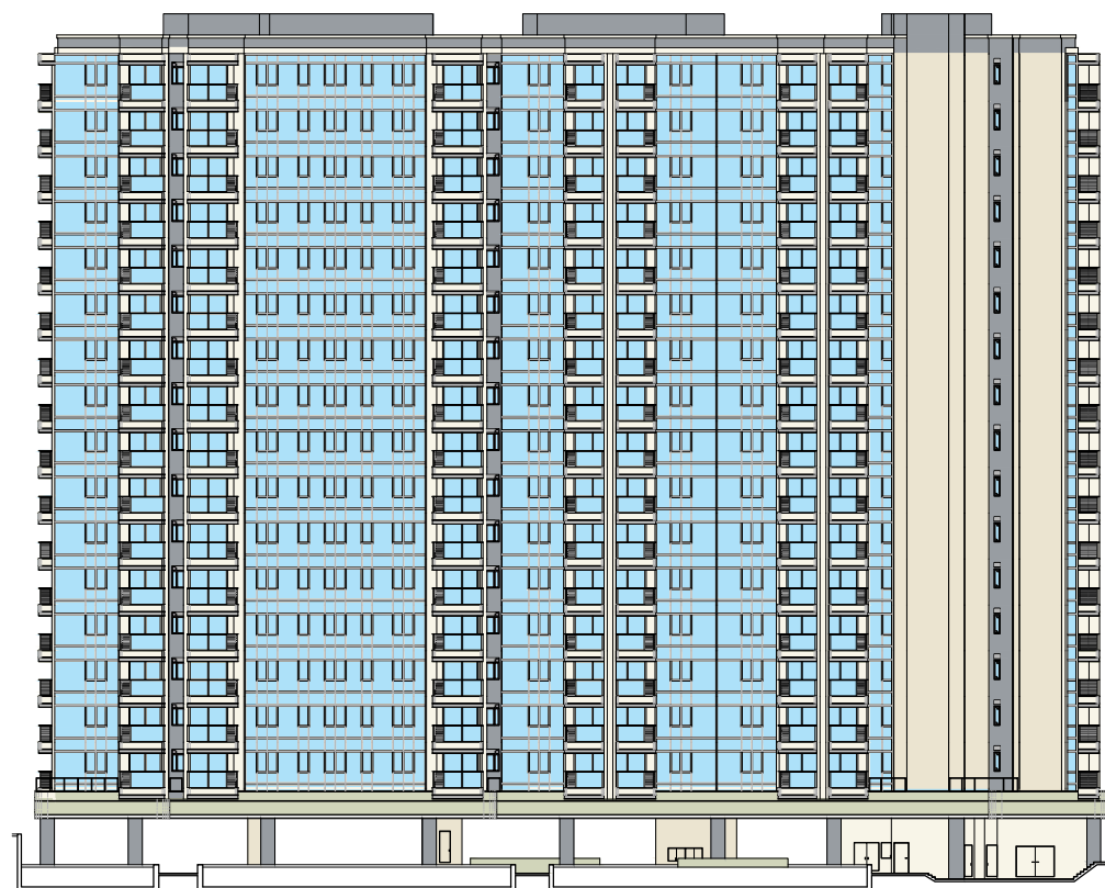
Elevation C 立面圖 C
