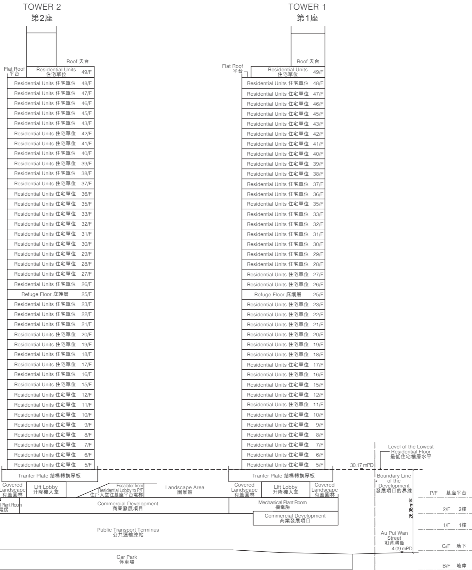
CROSS-SECTION A-A 橫截面圖 A-A
