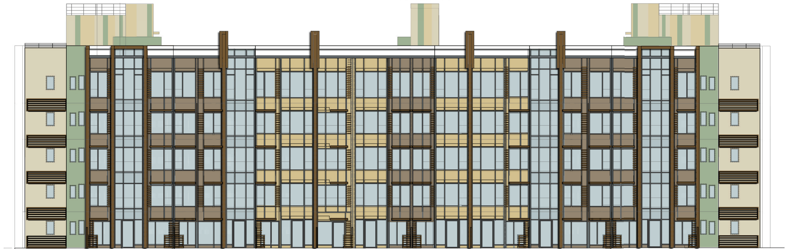
大樓1B座北立面圖 TOWER 1B NORTH ELEVATION
