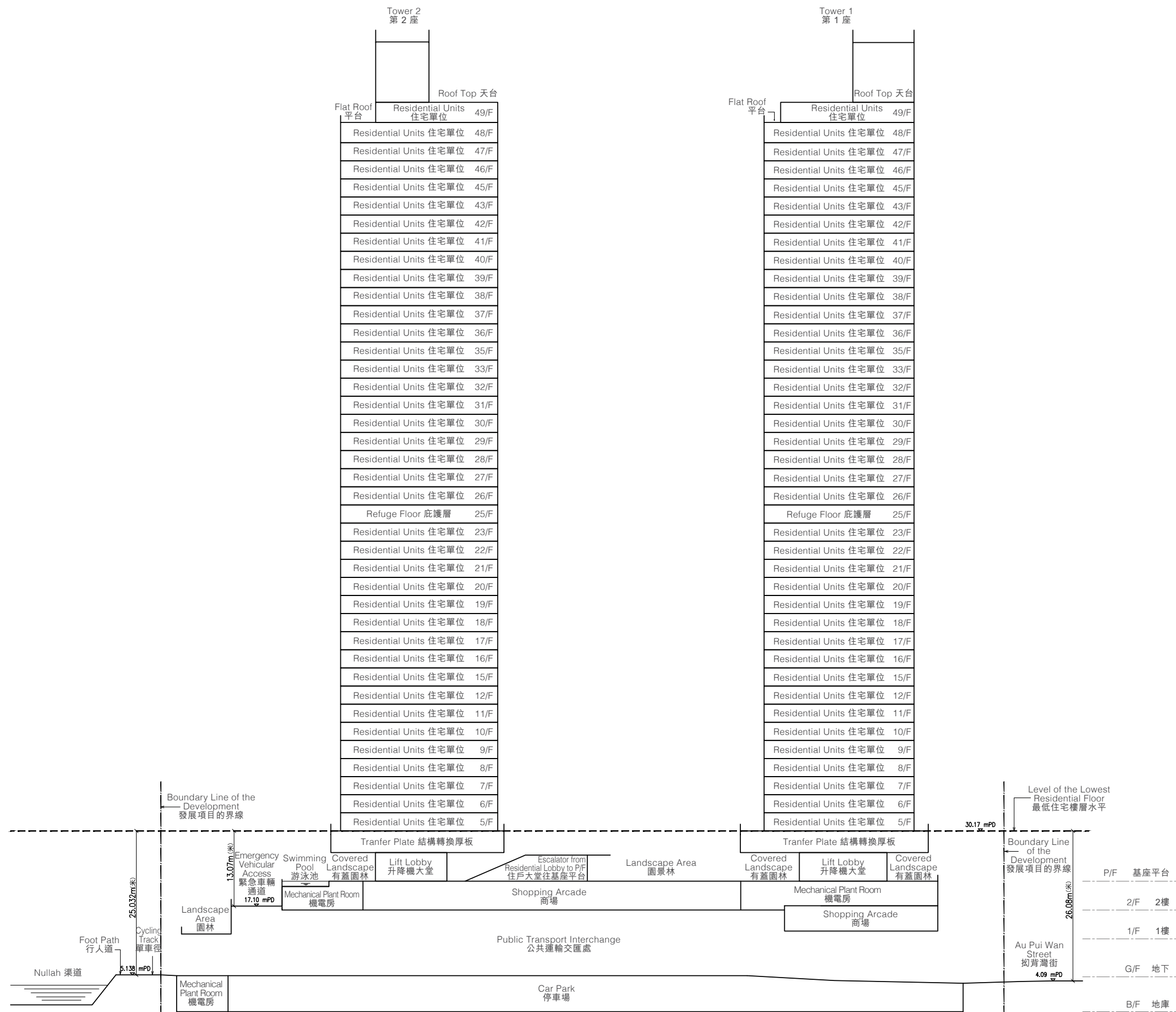
CROSS-SECTION A-A 橫截面圖 A-A
