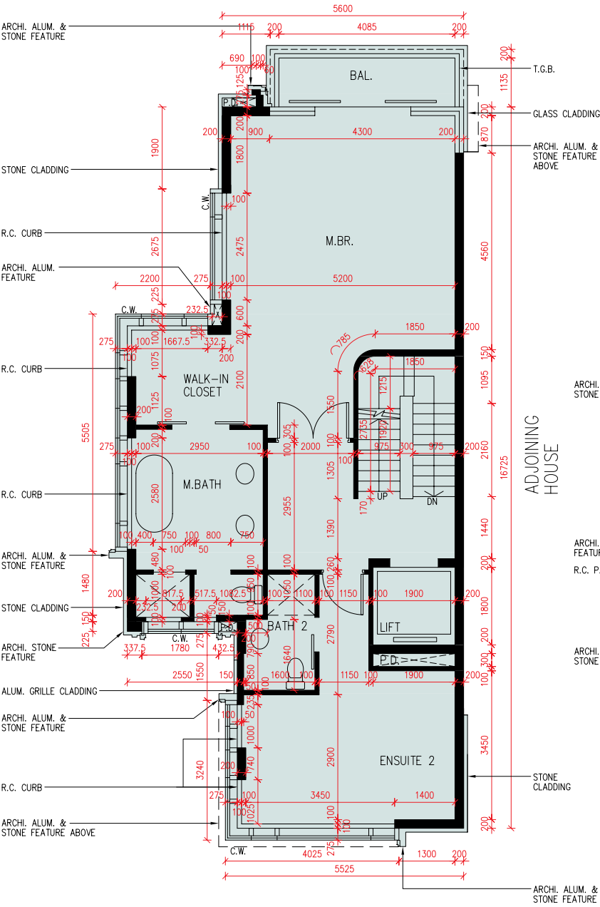
2/F Plan 2樓平面圖
