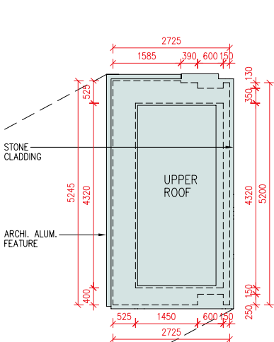
Upper Roof Plan 上層天台平面圖
