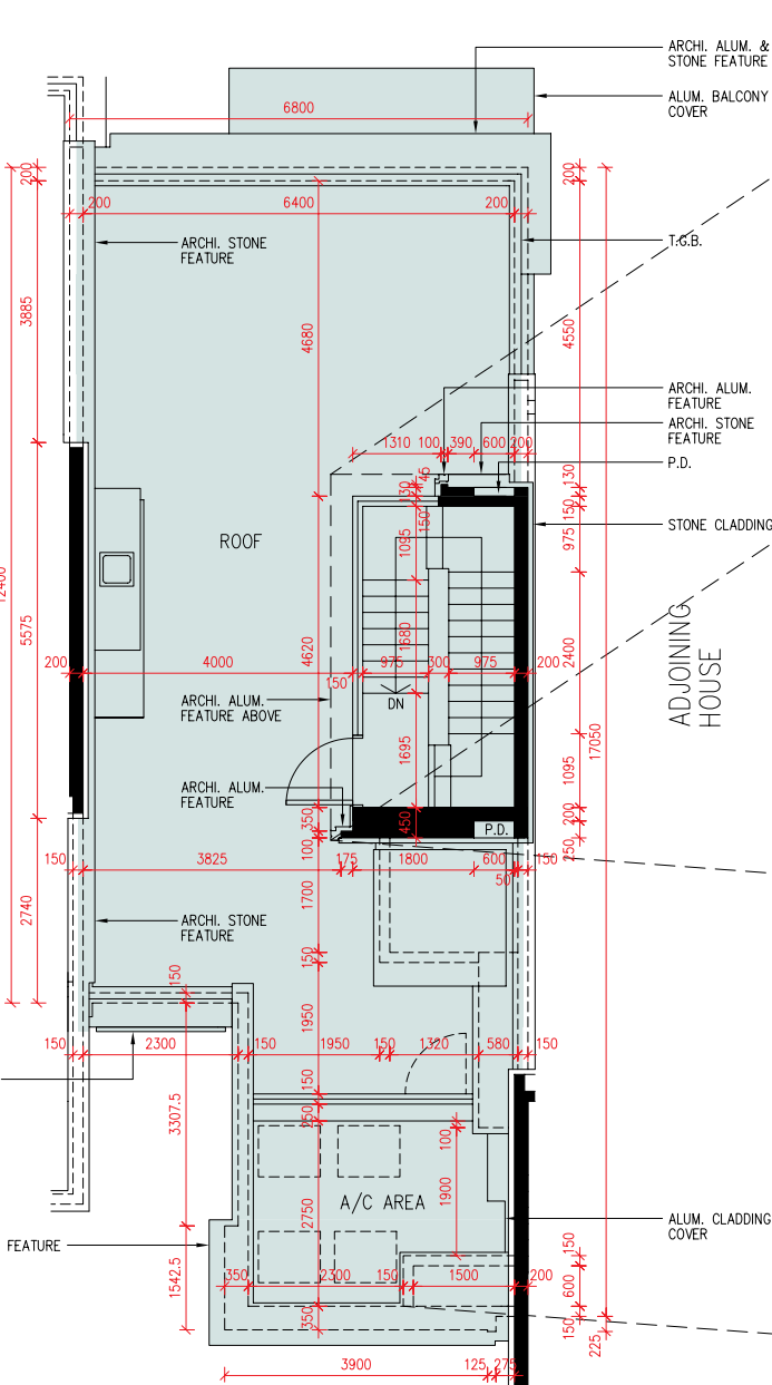
Roof Plan 天台平面圖
