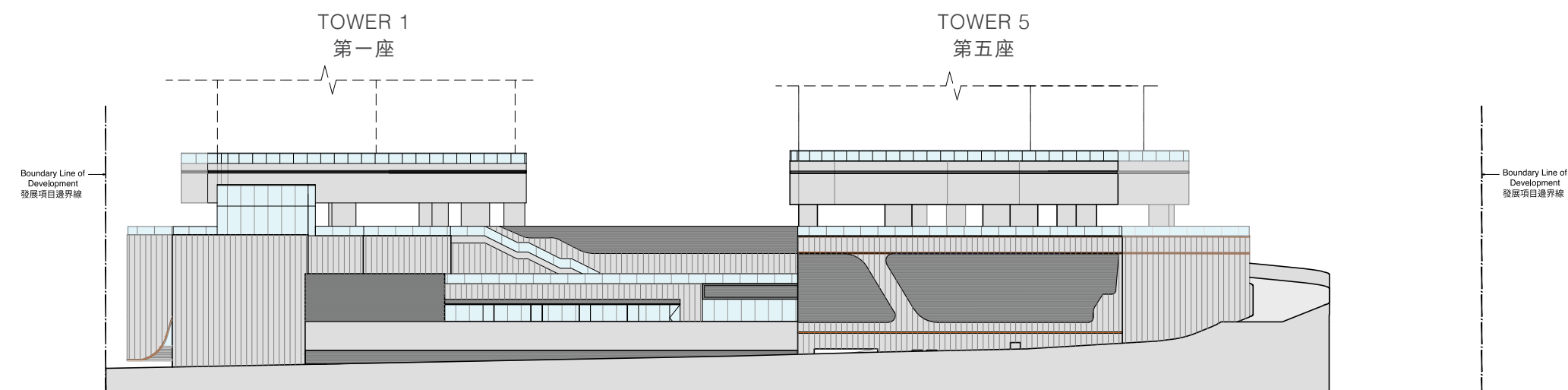
ELEVATION PLAN 3 立面圖 3
