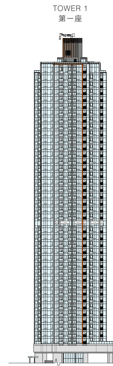
ELEVATION PLAN 4 立面圖 4
