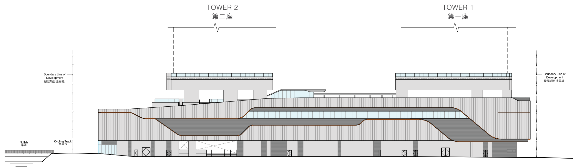
ELEVATION PLAN 1 立面圖 1
