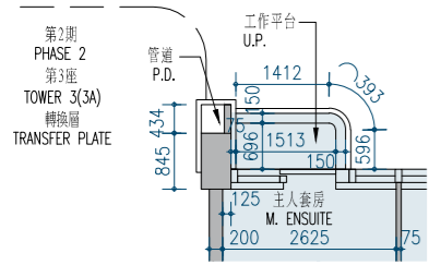
2/F Unit C Part Plan 2樓C單位之部分平面圖
