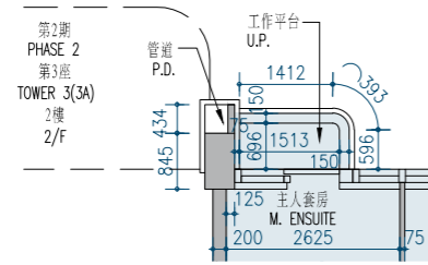
3/F Unit C Part Plan 3樓C單位之部分平面圖
