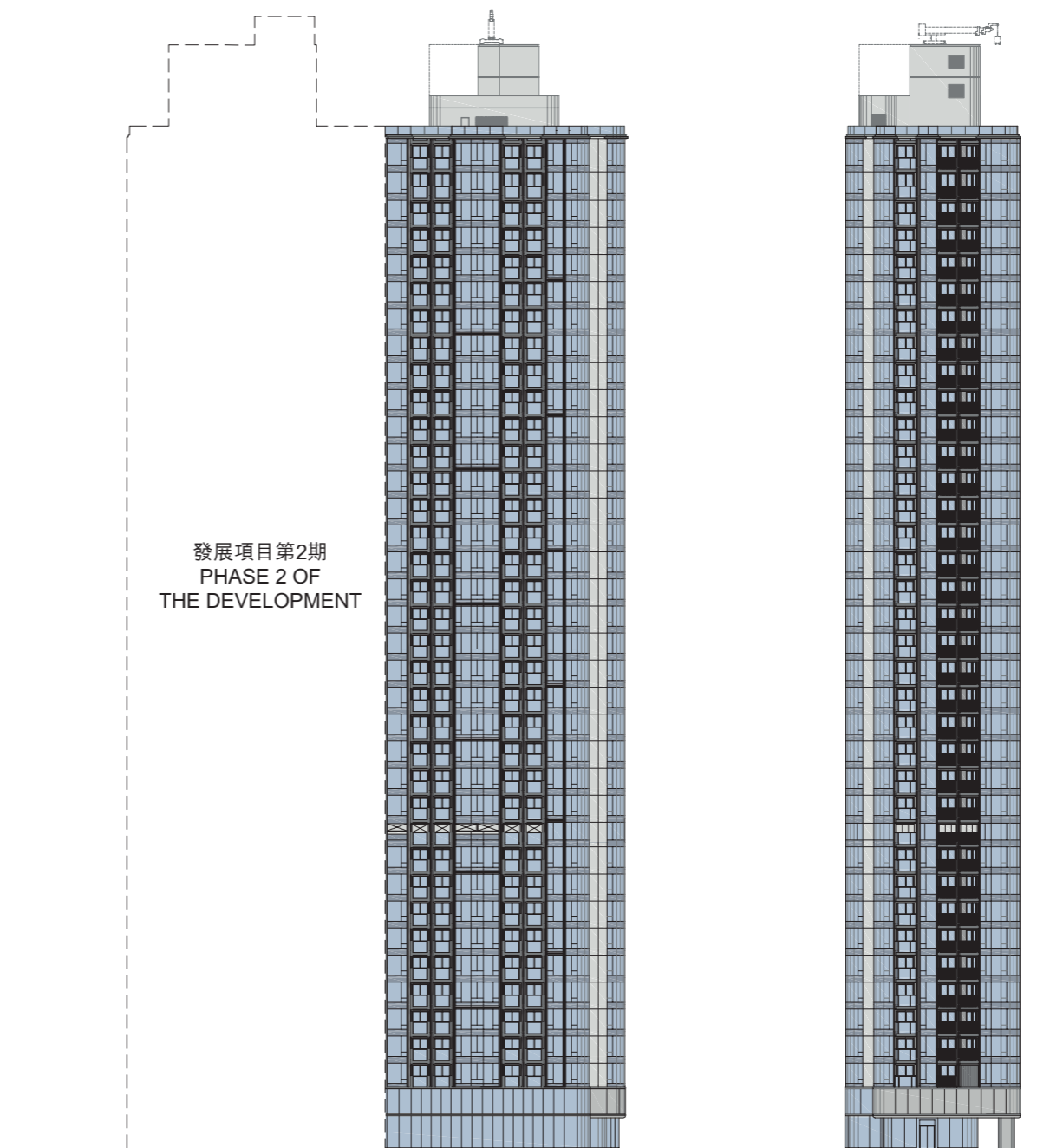
立面圖 B ELEVATION PLAN B
