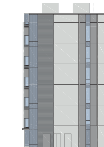
立面圖 B ELEVATION PLAN B
