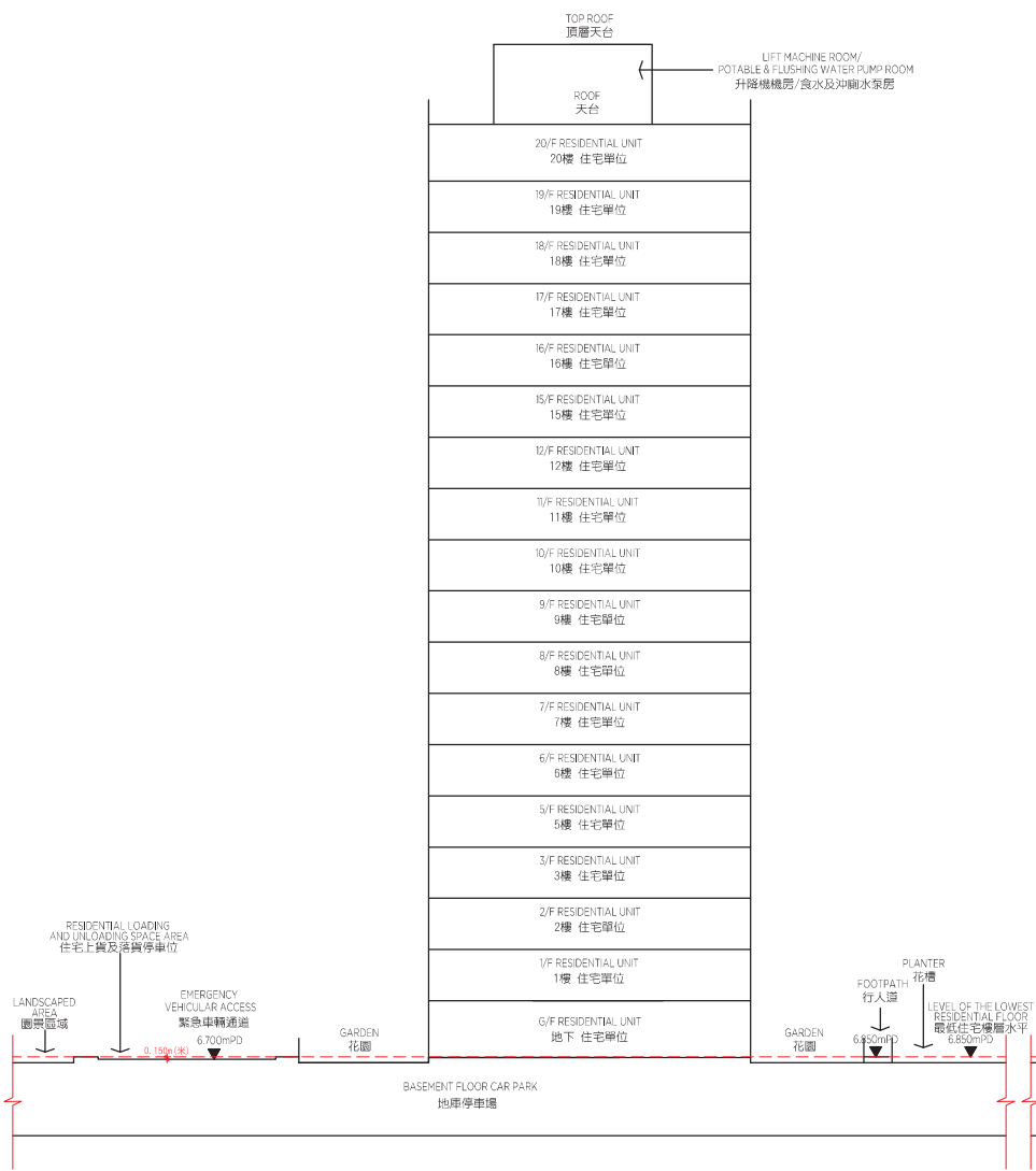
CROSS-SECTION PLAN D 橫截面圖 D TOWER 5 第5座
