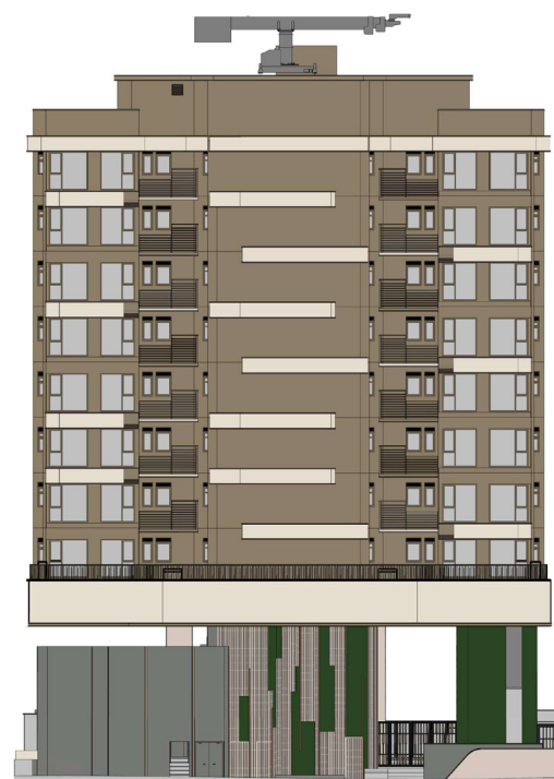
SOUTHEAST ELEVATION 東南面立面圖
