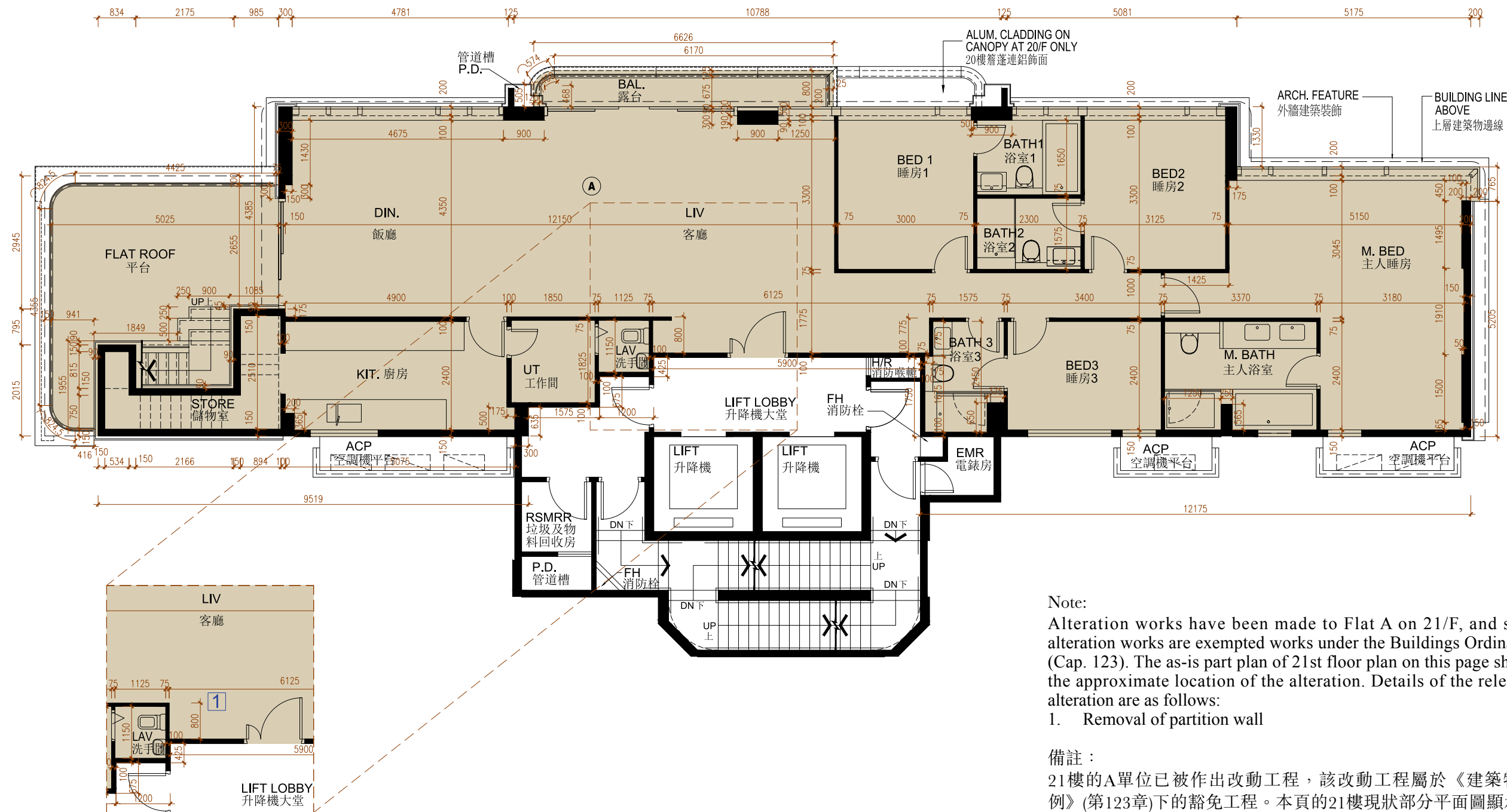
AS-IS PART PLAN OF 21/F 21樓現狀部分平面圖
