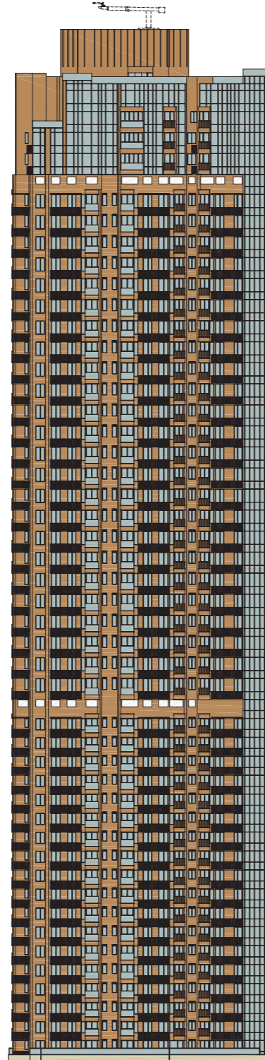
ELEVATION 2 立面圖 2
