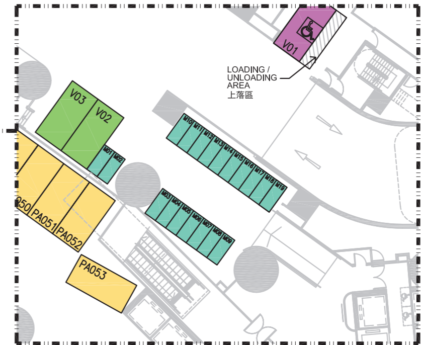
PART PLAN OF MOTOR CYCLE PARKING SPACE 電單車停車位部分平面圖
