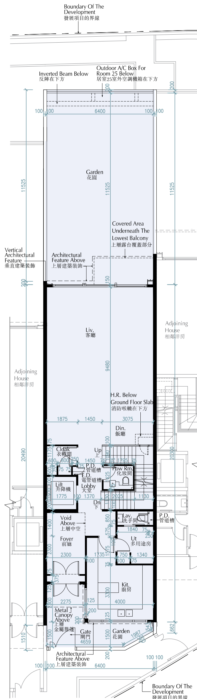
G/F Plan 地下平面圖
