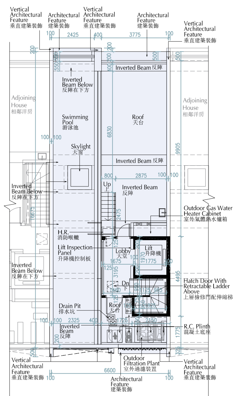
天台平面圖
