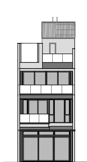
Elevation 1 立面1
