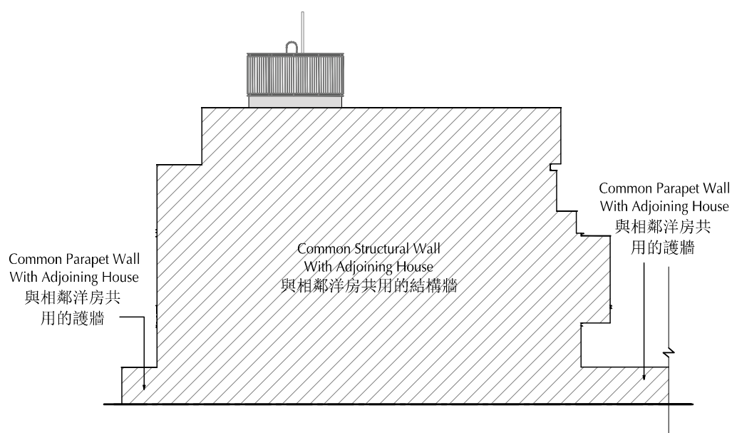
Elevation 2 立面2
