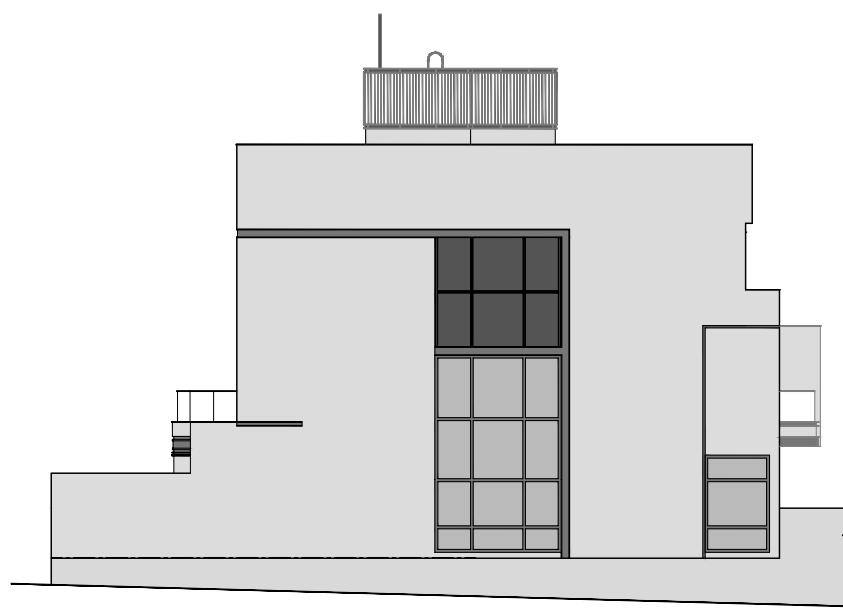
Elevation 2 立面2
