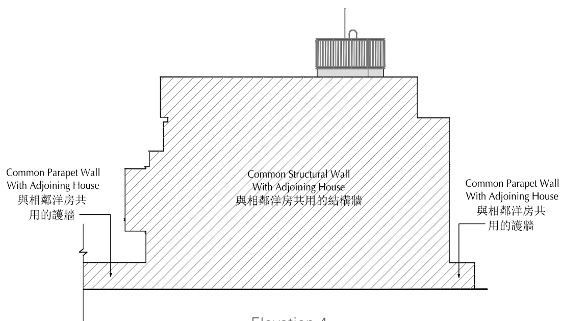
Elevation 4 立面4
