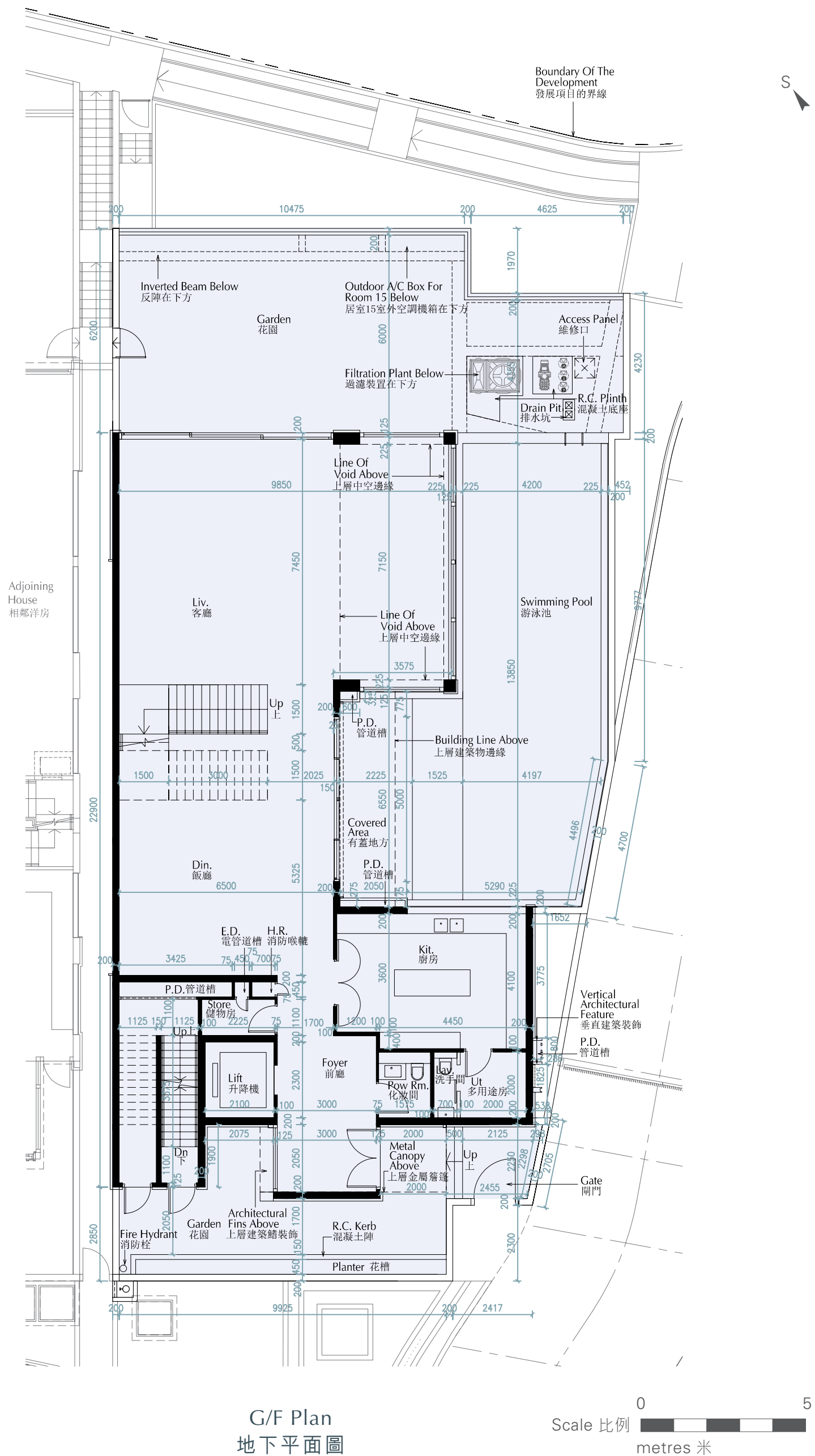
HOUSE 15 Floor Plan 15號洋房樓面平面圖
