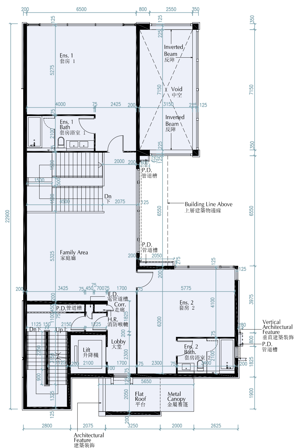
1/F Plan 1樓平面圖
