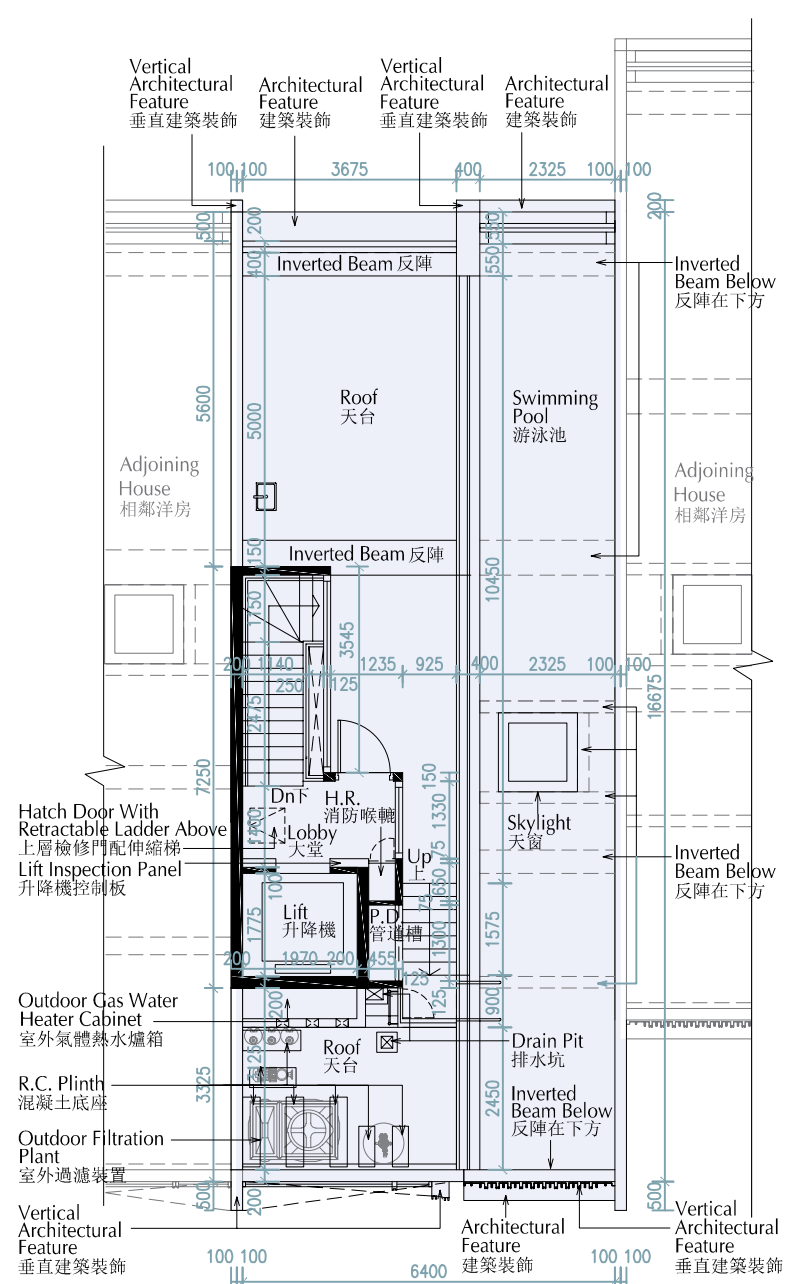
Roof Plan 天台平面圖
