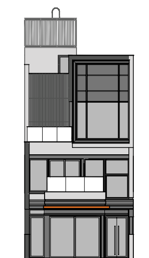
Elevation 3 立面3
