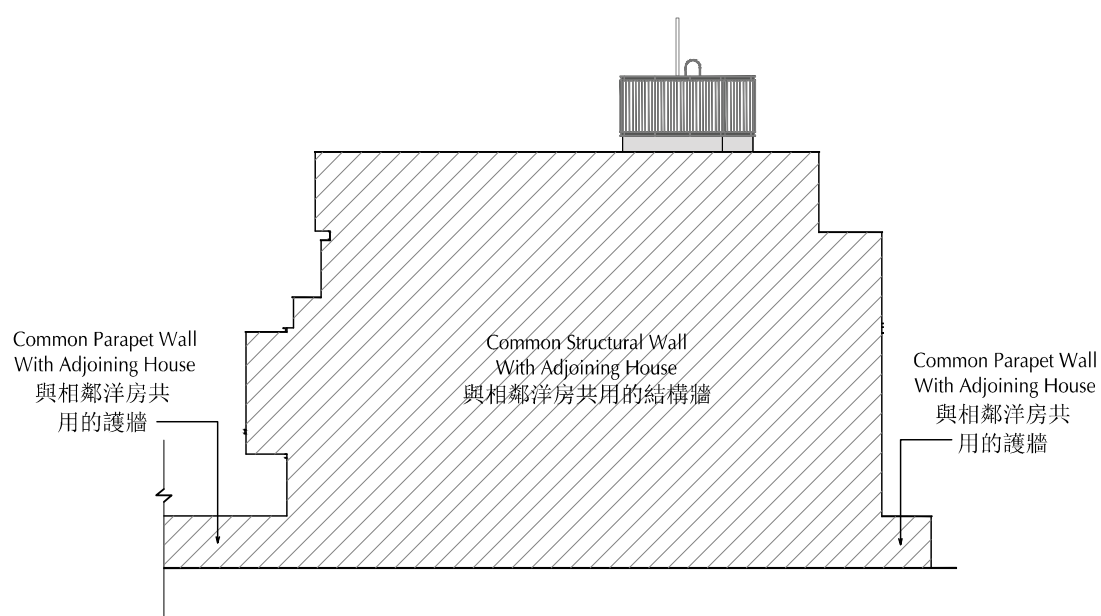
Elevation 4 立面4
