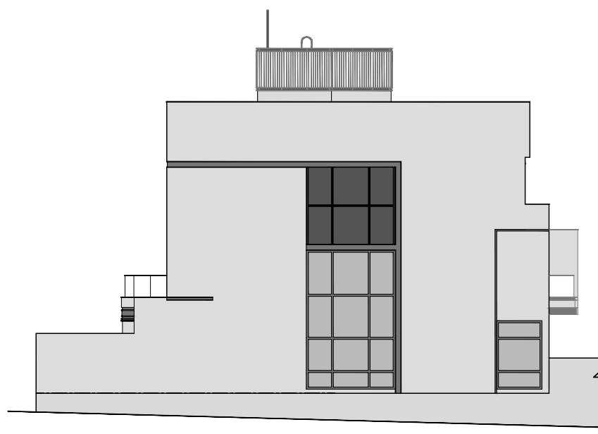
Elevation 2 立面2
