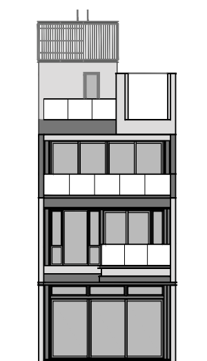
Elevation 1 立面1
