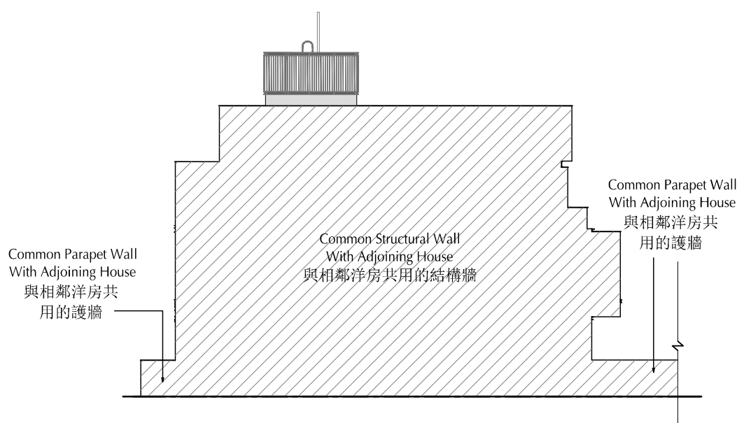
Elevation 2 立面2
