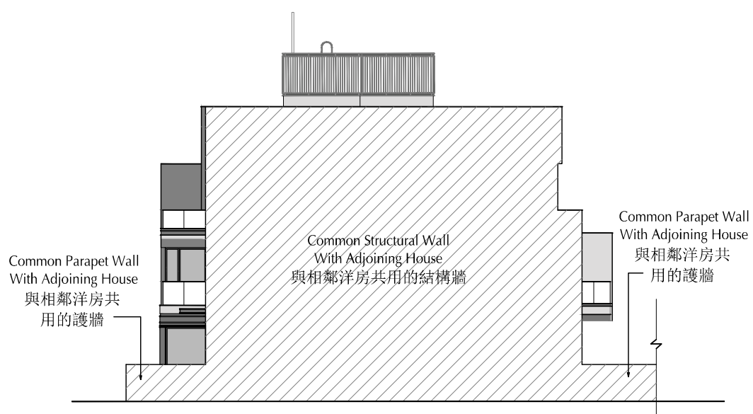
Elevation 2 立面2
