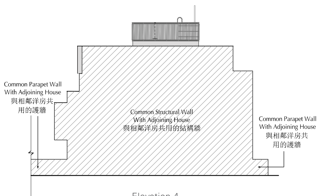
Elevation 4 立面4
