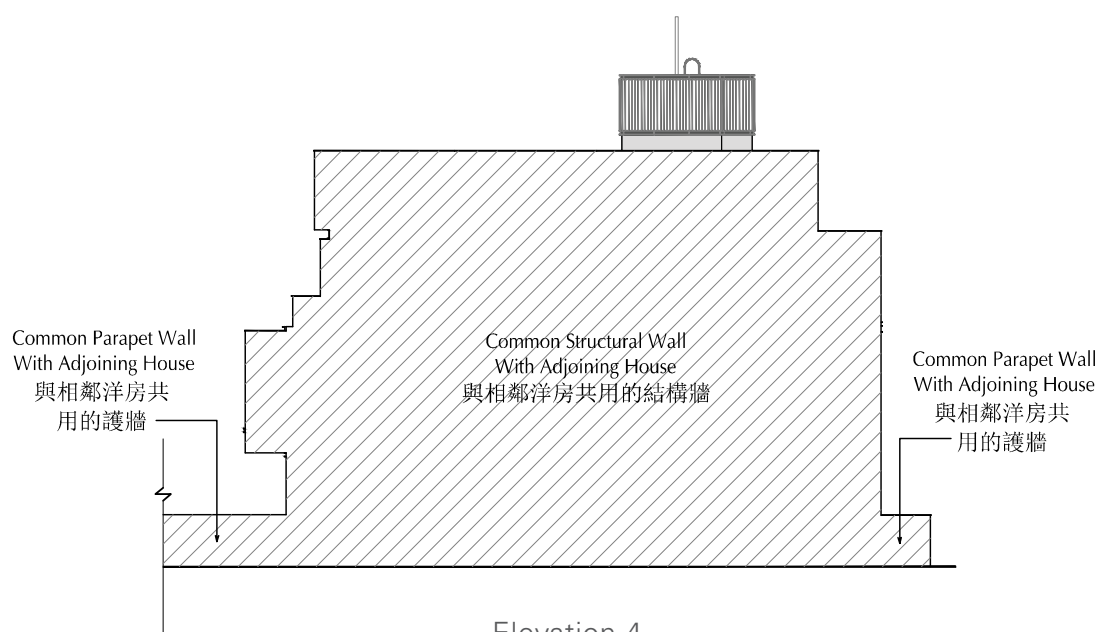
Elevation 4 立面4
