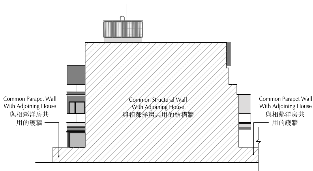
Elevation 2 立面2
