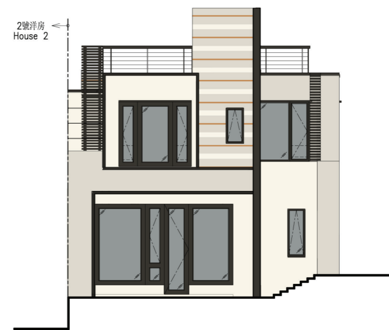
1號洋房立面圖 2 HOUSE 1 ELEVATION 2
