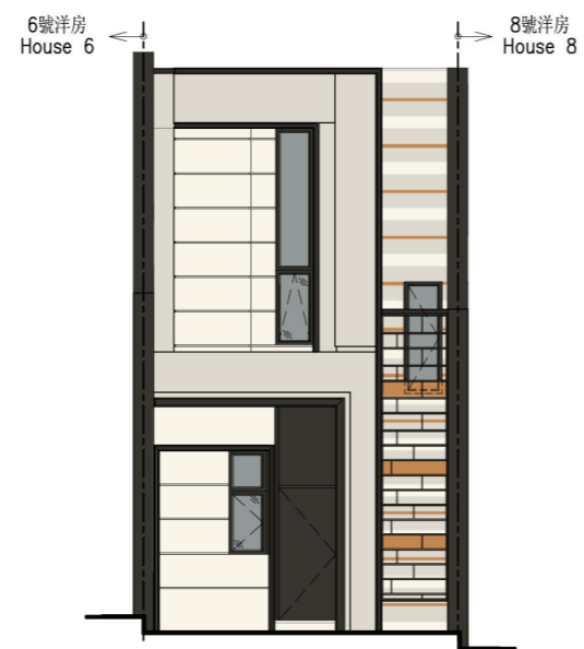
7號洋房立面圖 1 HOUSE 7 ELEVATION 1
