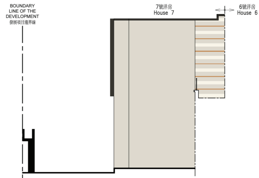
7號洋房立面圖 2 HOUSE 7 ELEVATION 2
