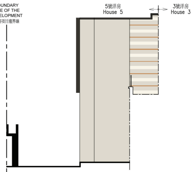
5號洋房立面圖 2 HOUSE 5 ELEVATION 2
