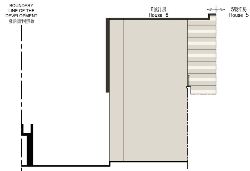
6號洋房立面圖 2 HOUSE 6 ELEVATION 2
