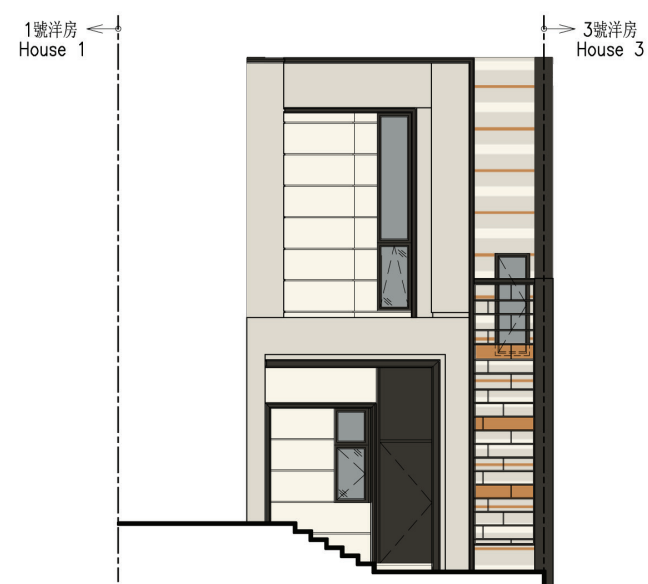
2號洋房立面圖 1 HOUSE 2 ELEVATION 1
