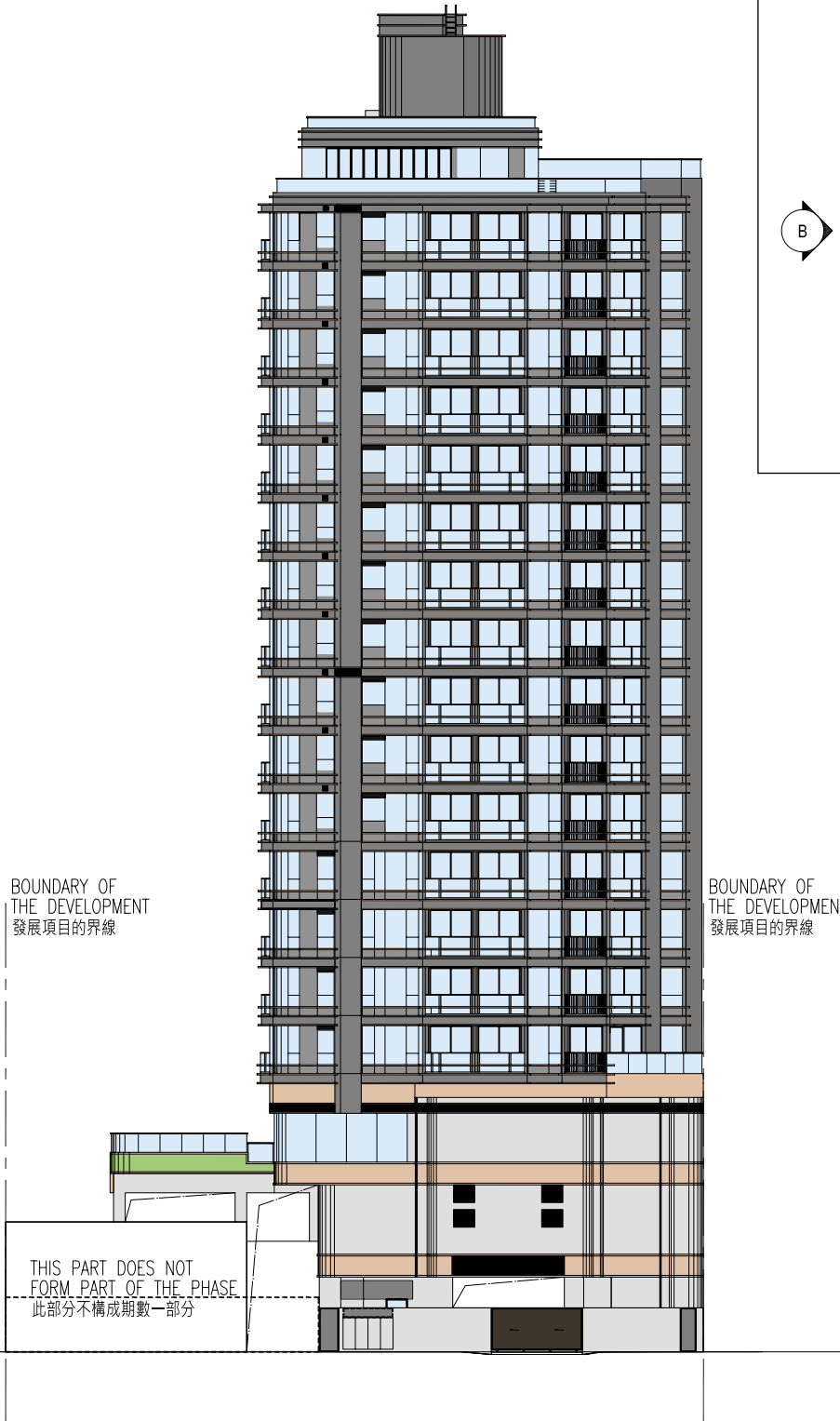
Elevation B 立面圖 B
