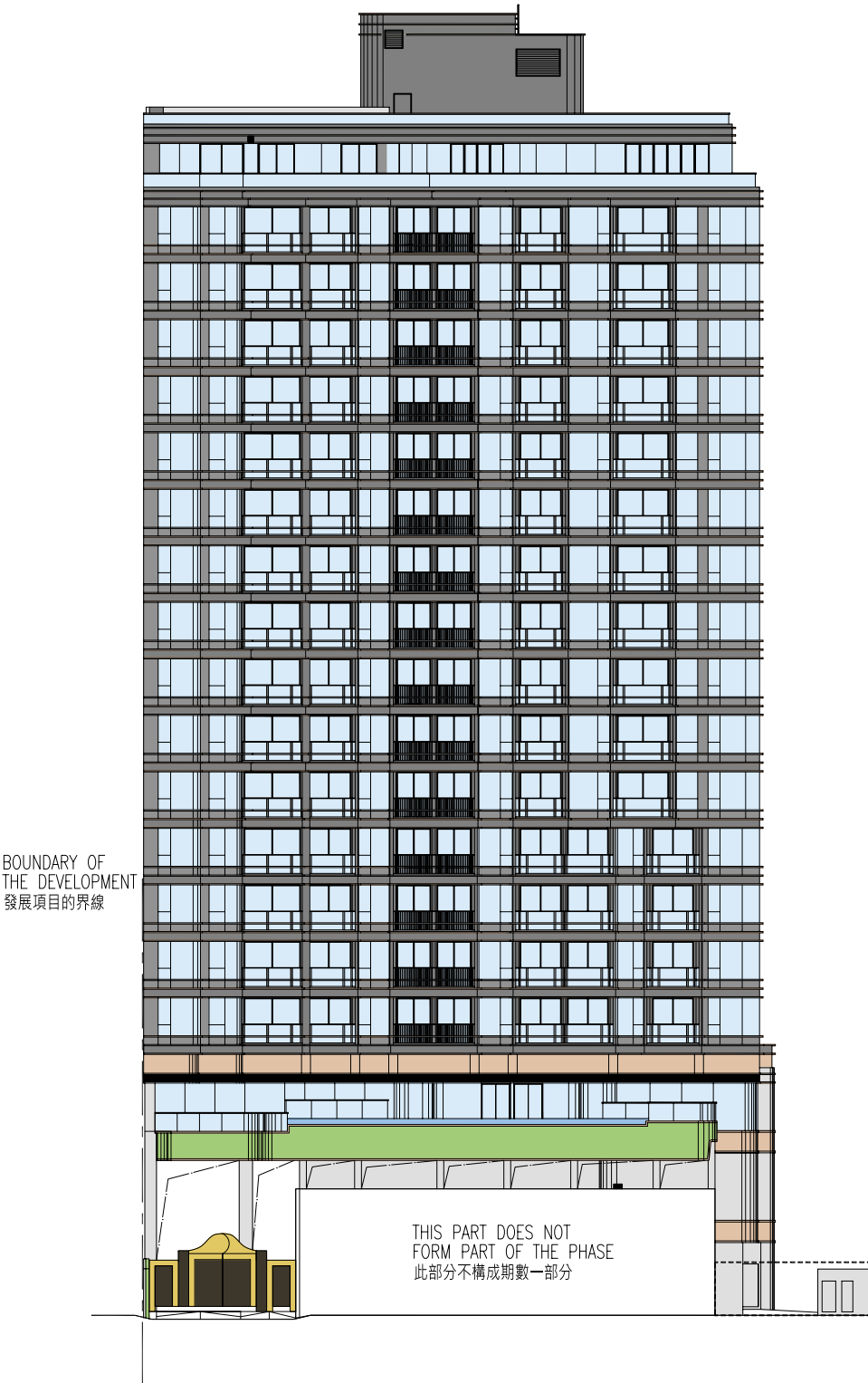
Elevation A 立面圖 A
