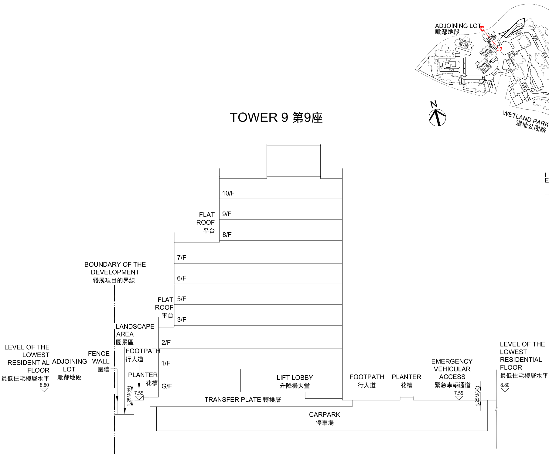
CROSS-SECTION PLAN D1 橫截面圖D1
