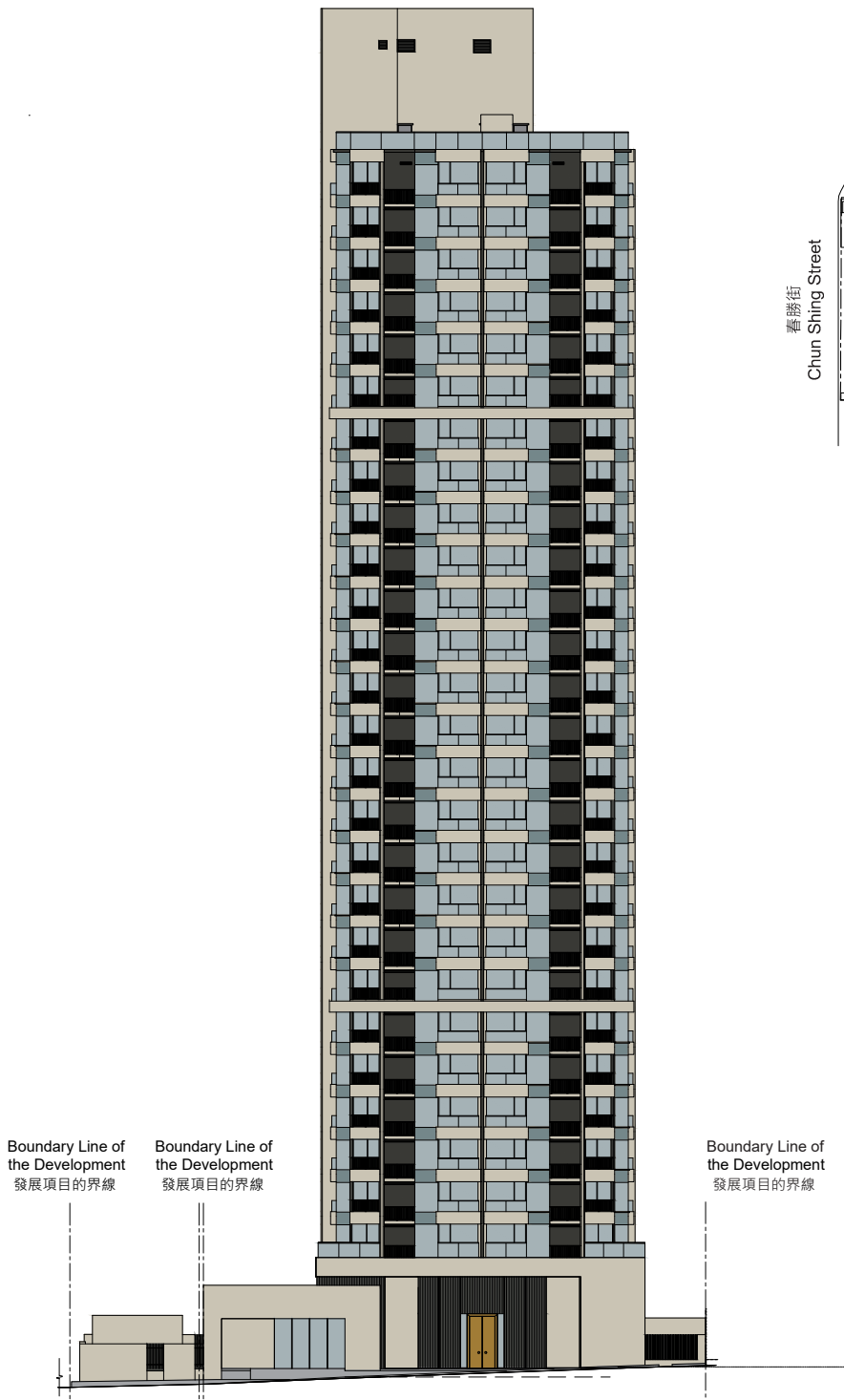
Elevation Plan A 立面圖 A
