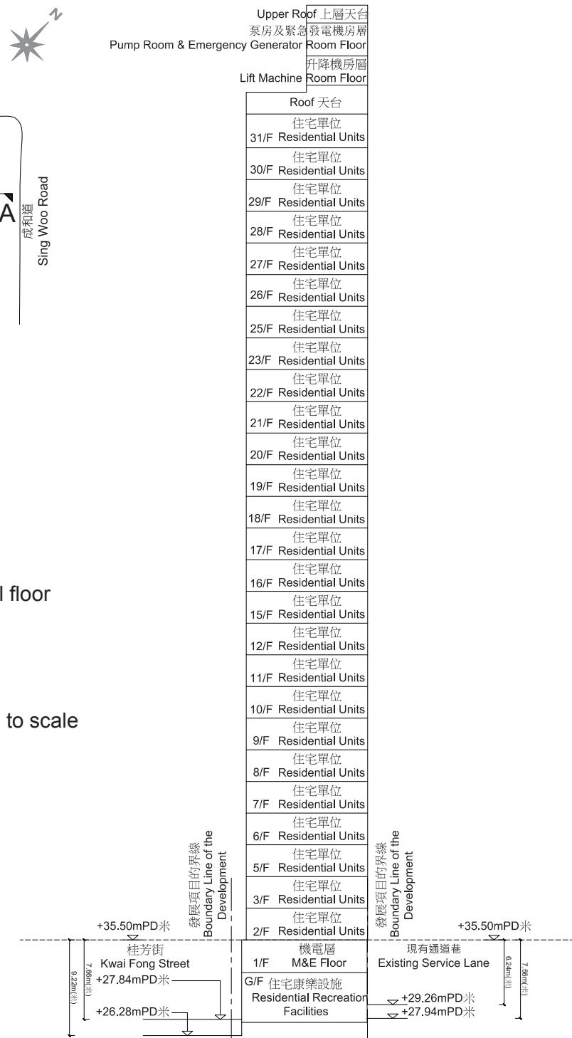
Cross-Section Plan B - B 橫截面圖 B - B
