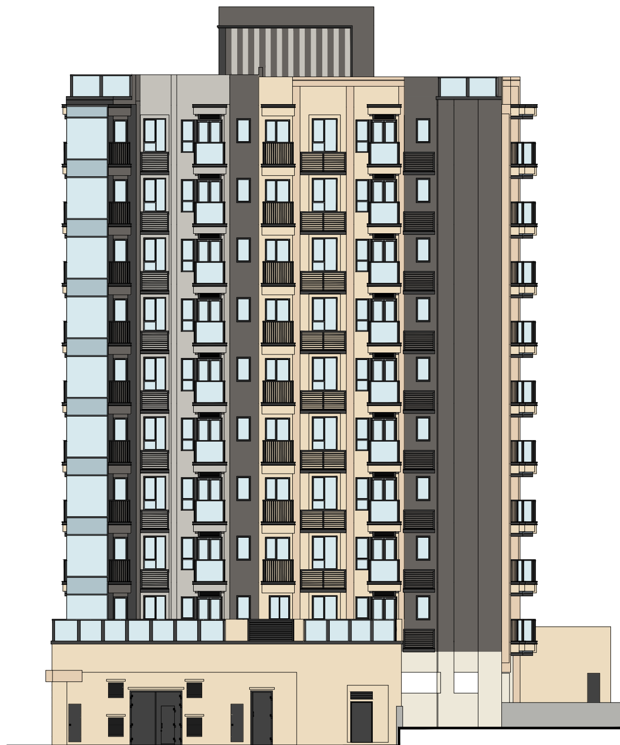
Elevation Plan B1 立面圖 B1
