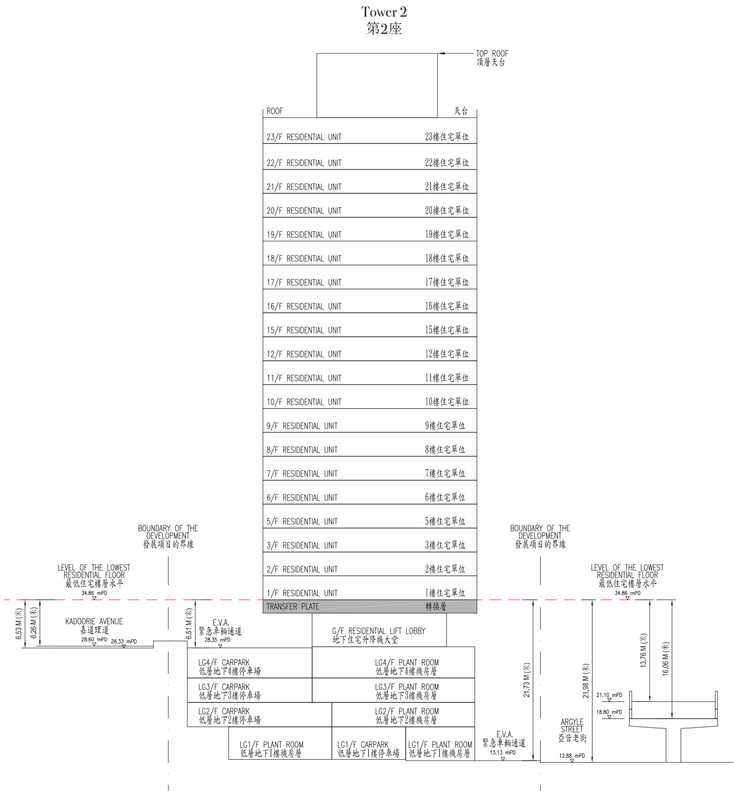
Cross-section Plan 2 橫截面圖 2
