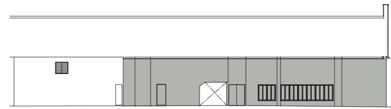
大廈平台立面圖21 PODIUM ELEVATION 21
