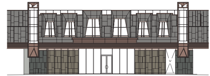
大廈平台立面圖4 PODIUM ELEVATION 4
