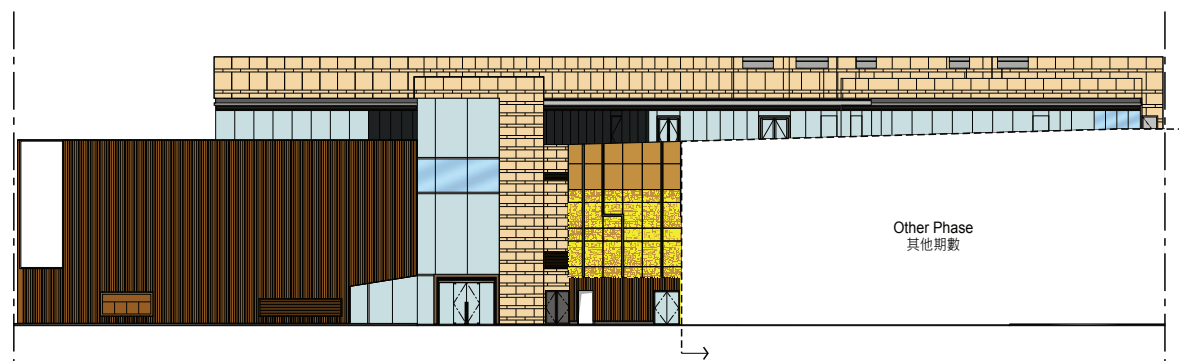
Podium Elevation 3 平台立面圖 3
