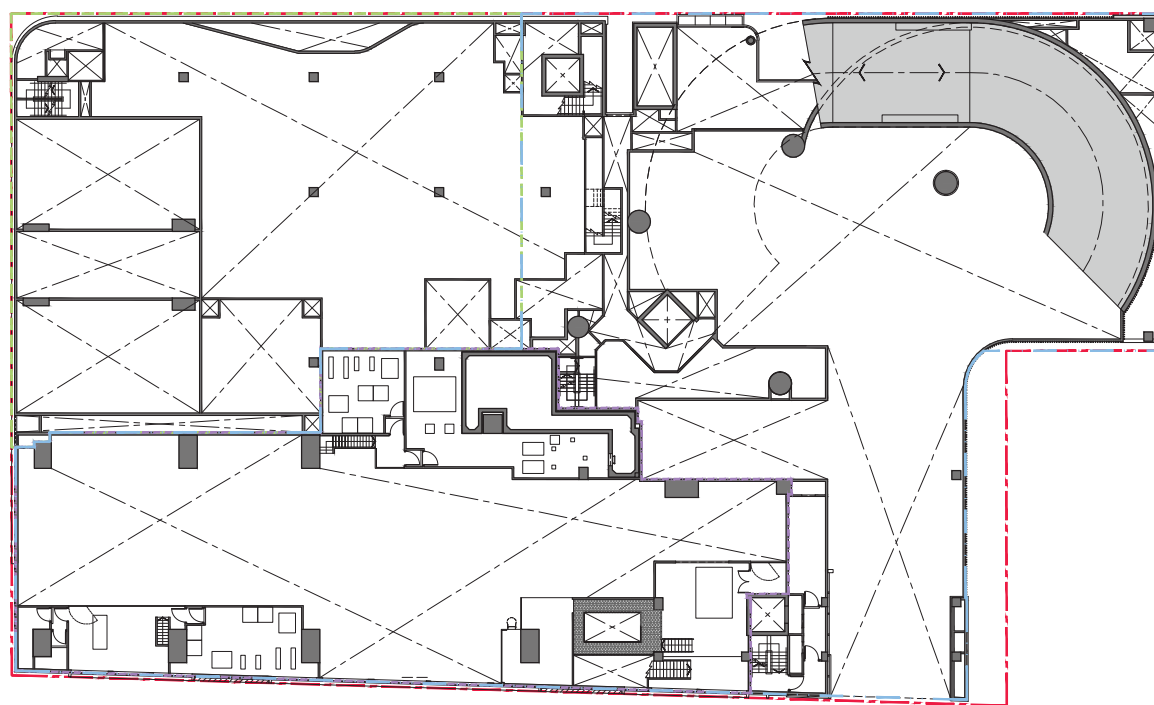
UPPER GROUND FLOOR PLAN 地下高層平面圖
