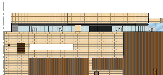
Podium Elevation 1 平台立面圖 1
