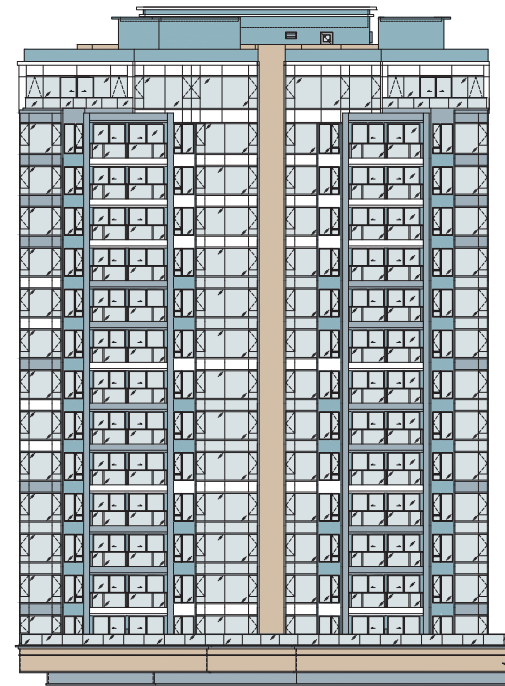
Elevation 4 立面 4
