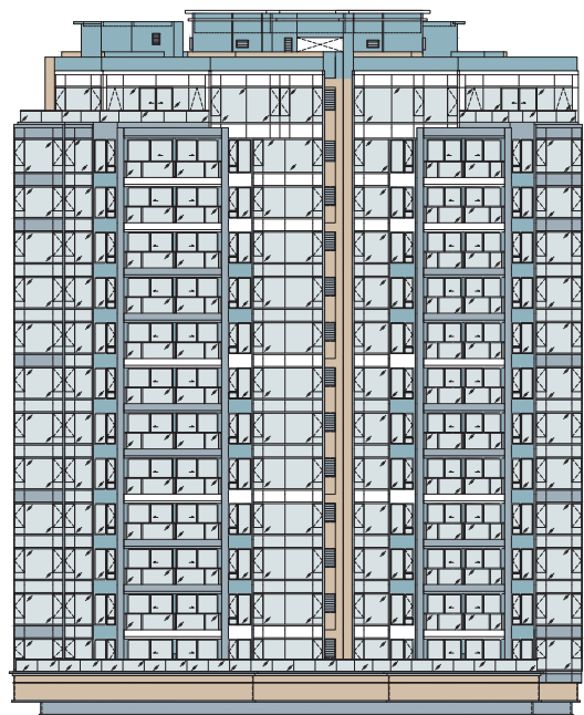
Elevation 2 立面 2
