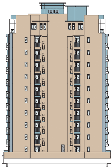
Elevation 2 立面 2
