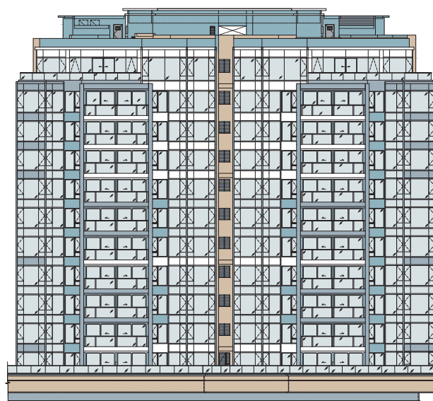
Elevation 2 立面 2
