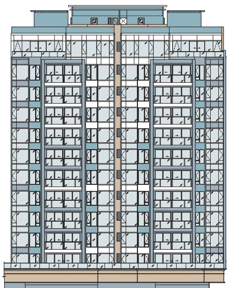
Elevation 3 立面 3
