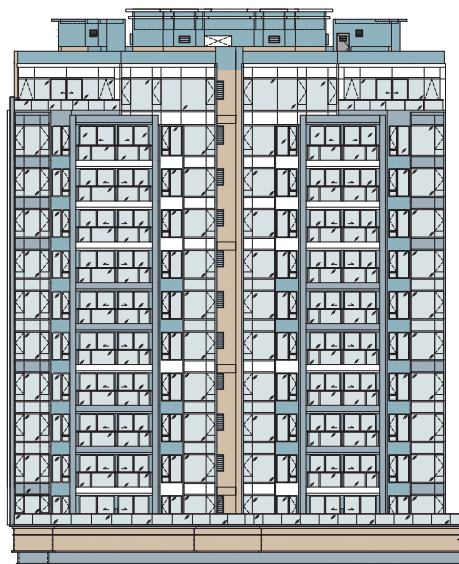
Elevation 1 立面 1
