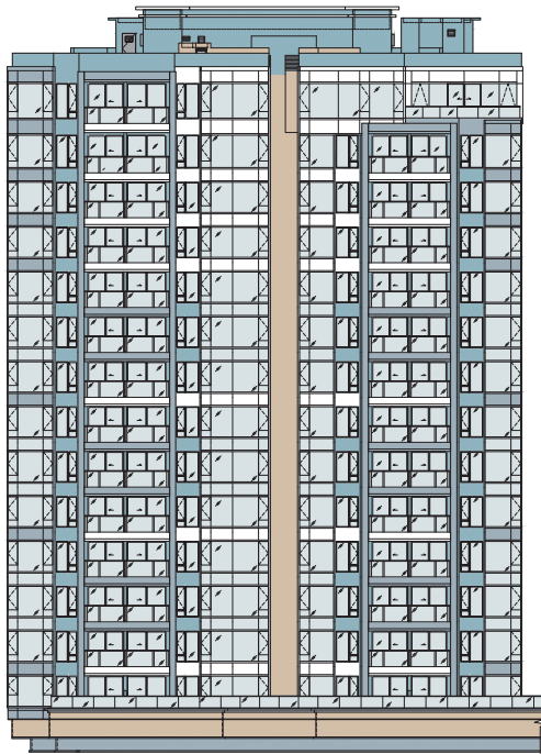
Elevation 2 立面 2
