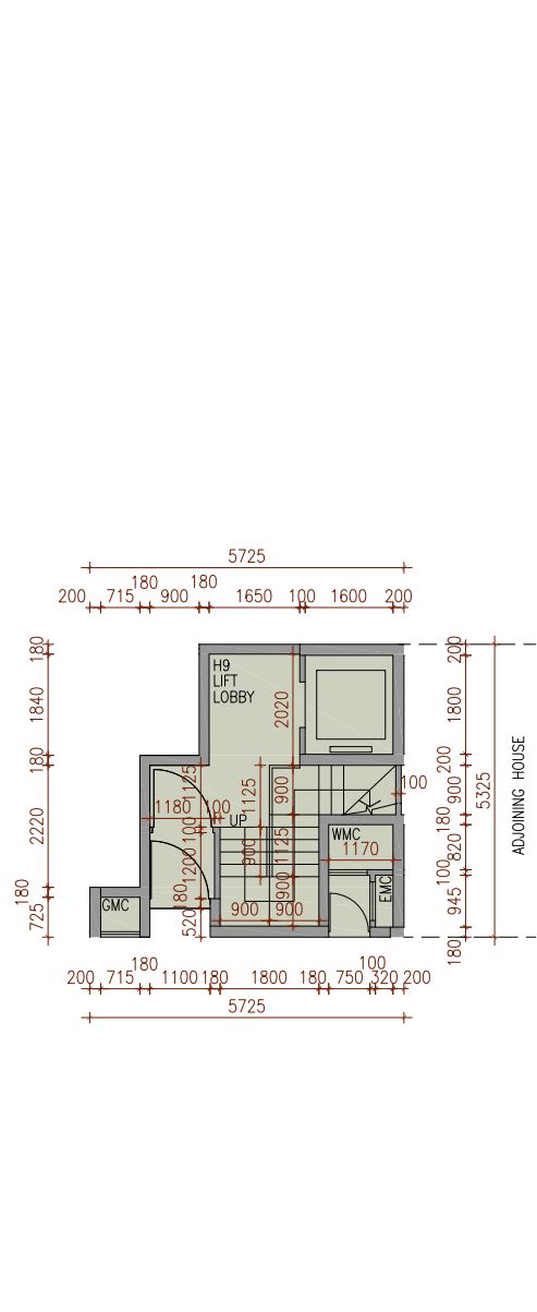
BASEMENT FLOOR PLAN 地庫層平面圖
