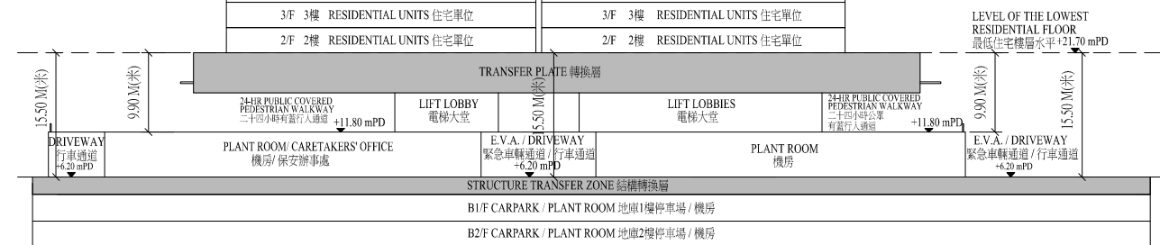
CROSS - SECTION PLAN C 橫截面圖 C
