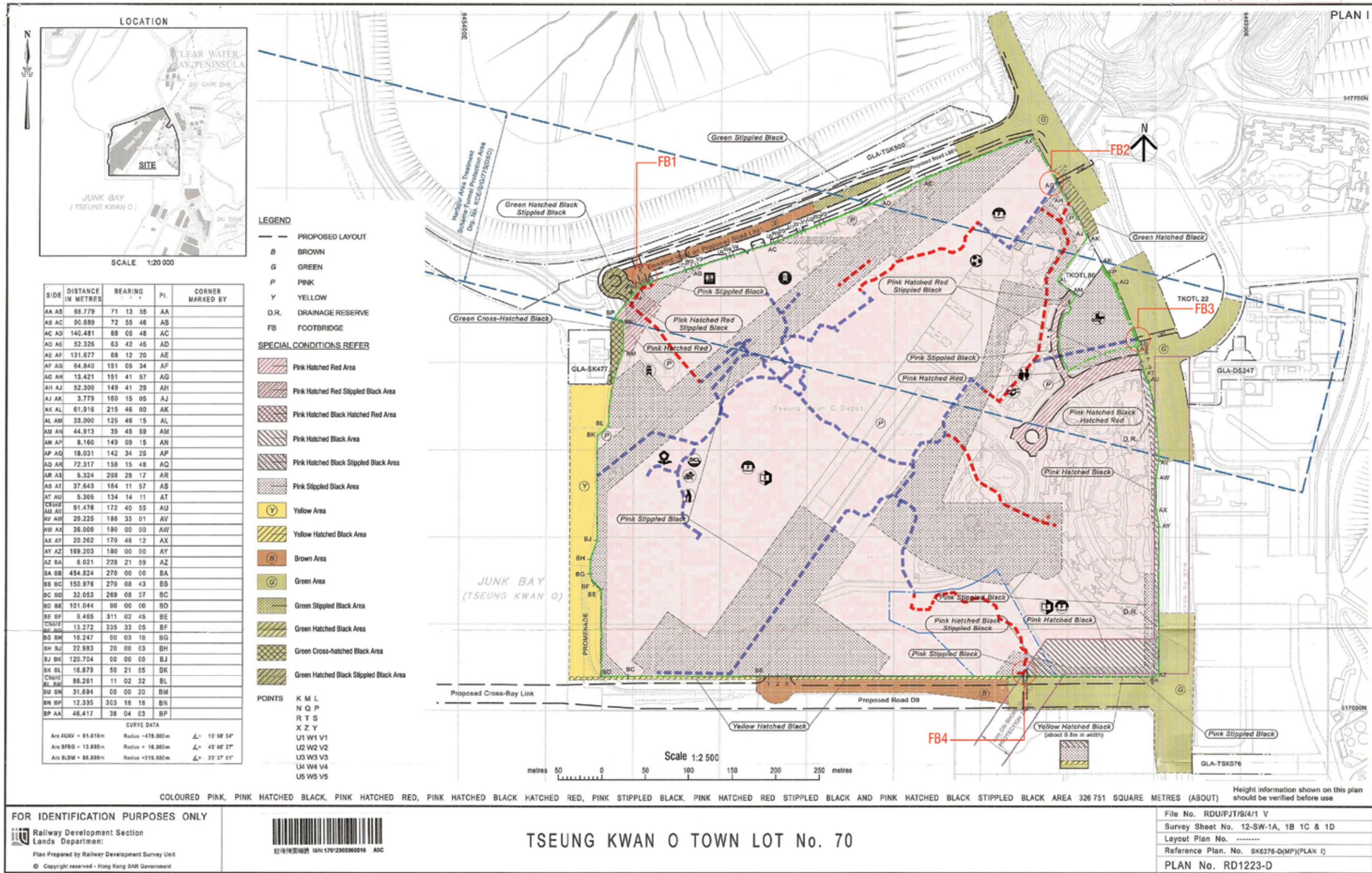
圖一 Plan 1
