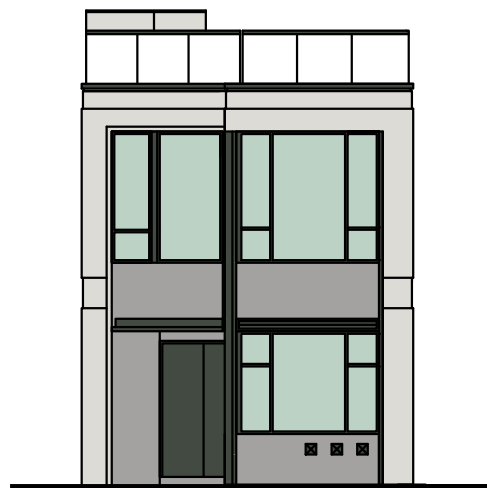
Elevation C (For Villa 2 to Villa 3, Villa 6 to Villa 12, Villa 15 to 16) 立面圖C(適用於2號洋房至3號洋房、 6號洋房至12號洋房、15號洋房至16號洋房)
