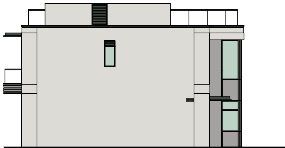
Elevation D (For Villa 2 to Villa 3, Villa 6 to Villa 12, Villa 15 to 16) 立面圖D(適用於2號洋房至3號洋房、 6號洋房至12號洋房、15號洋房至16號洋房)
