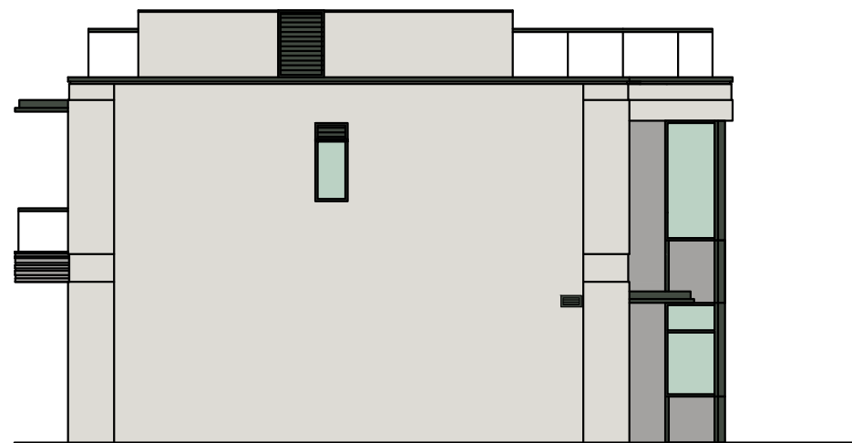
Elevation D (For Villa 1) 立面圖D(適用於1號洋房)
