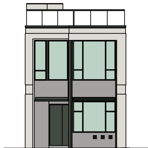
Elevation C (For Villa 1) 立面圖C(適用於1號洋房)
