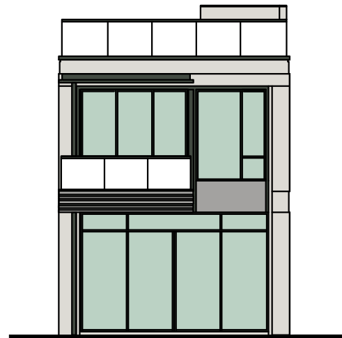
Elevation A (For Villa 17) 立面圖A(適用於17號洋房)
