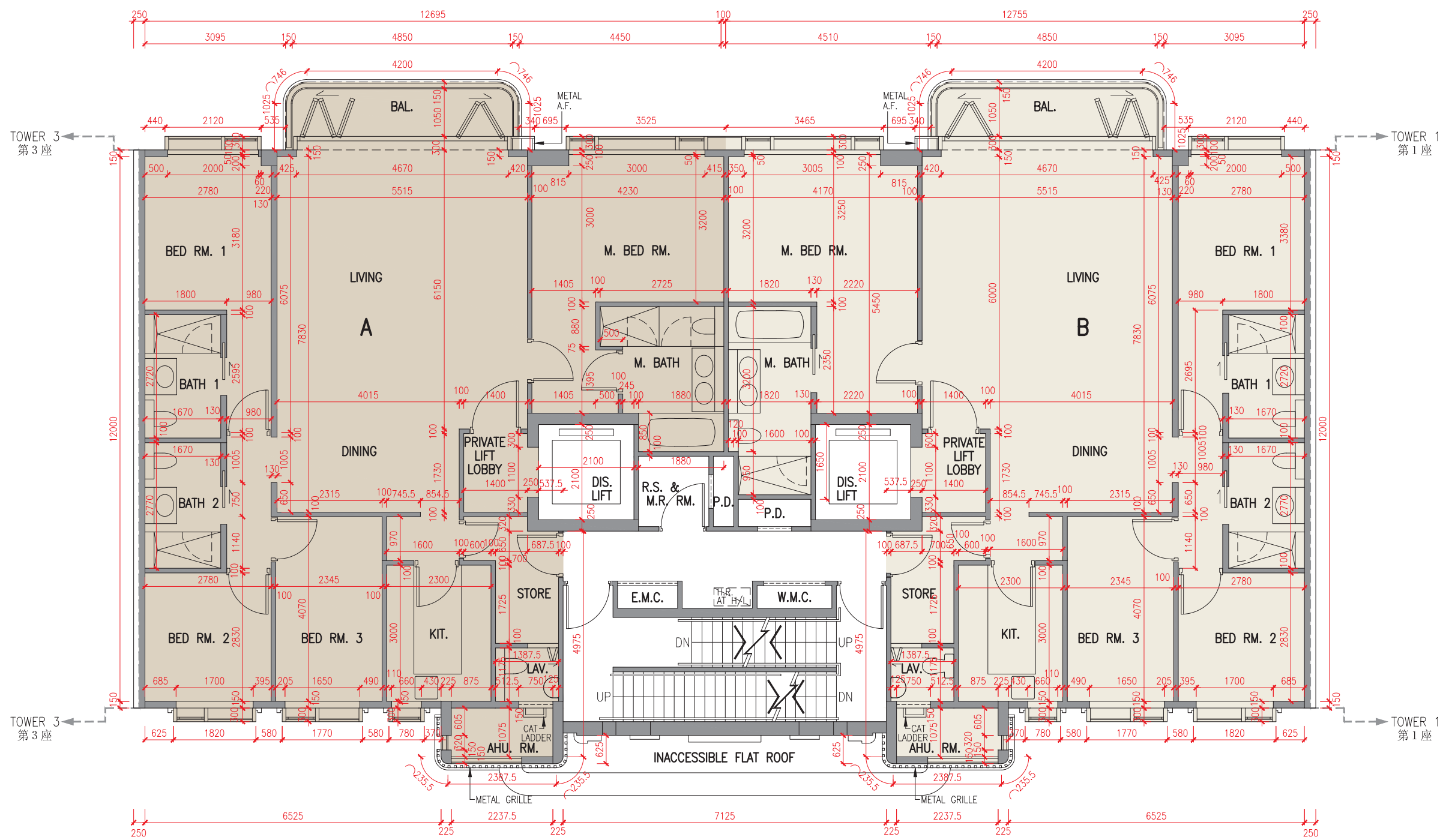
2樓平面圖 2/F Plan
