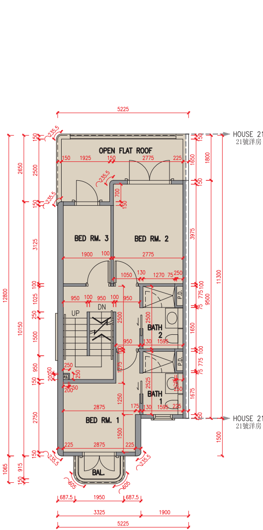
1樓平面圖 1/F Plan
