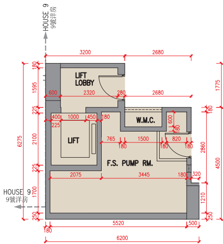
地庫平面圖 B/F Plan
