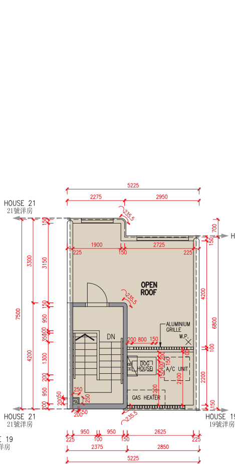
天台平面圖 Roof Plan
