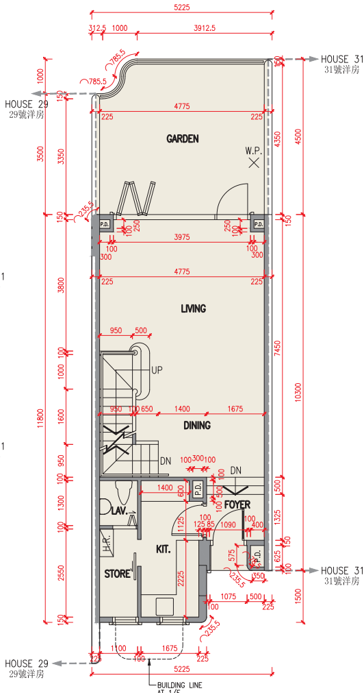
地下平面圖 G/F Plan
