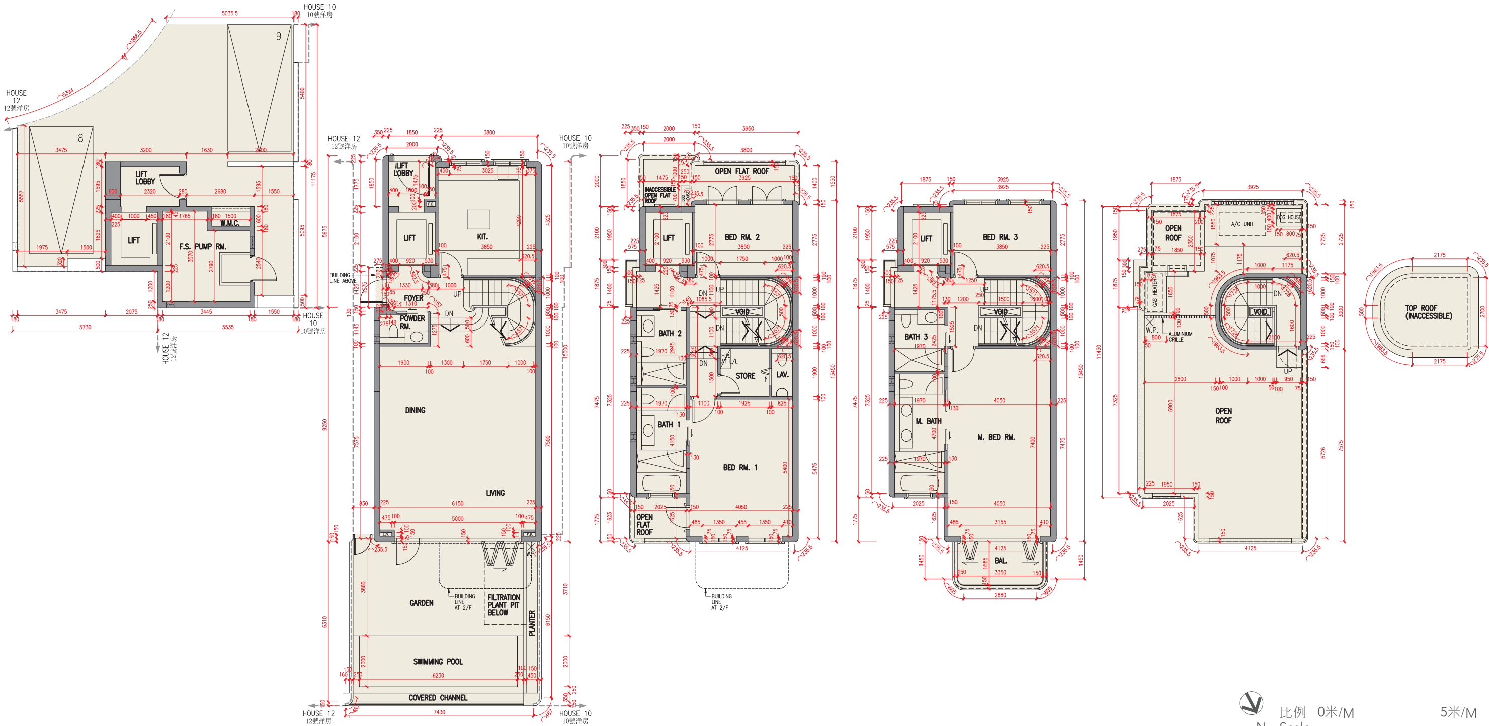
地庫平面圖 B/F Plan
