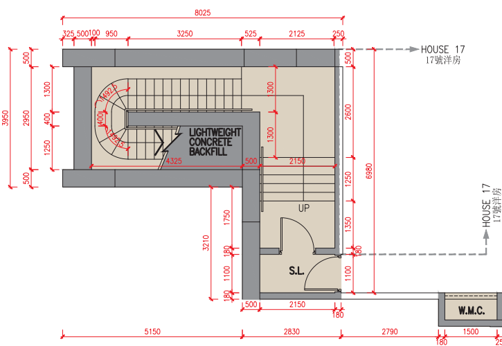
地庫平面圖 B/F Plan
