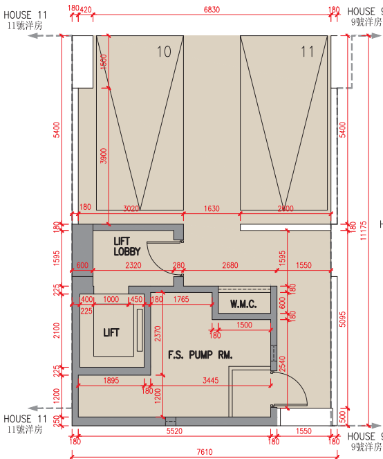
地庫平面圖 B/F Plan
