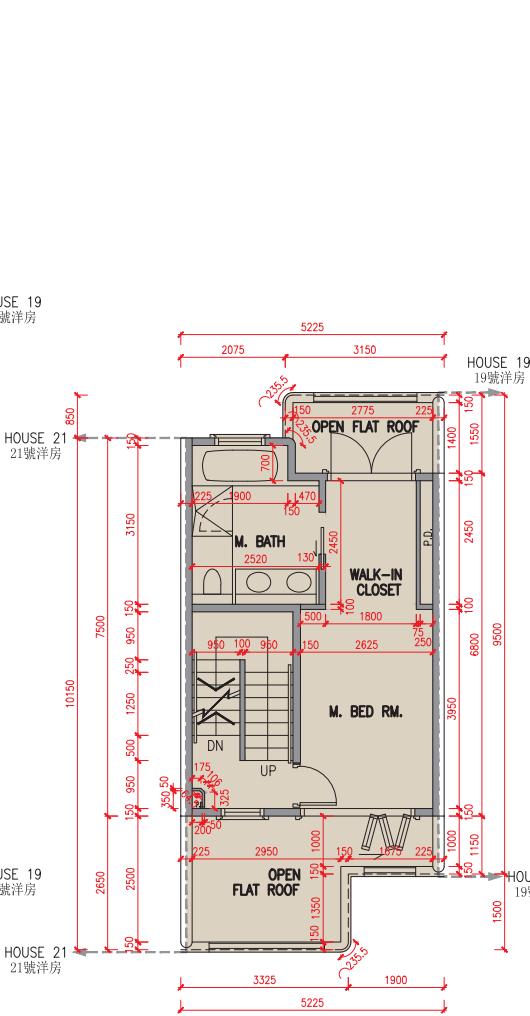
2樓平面圖 2/F Plan
