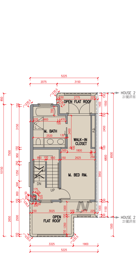
2樓平面圖 2/F Plan
