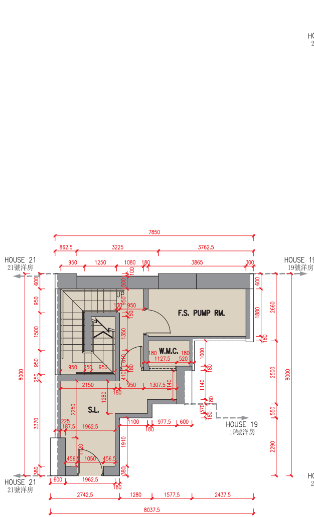
地庫平面圖 B/F Plan
