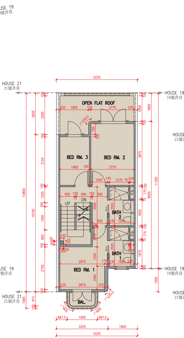
1樓平面圖 1/F Plan
