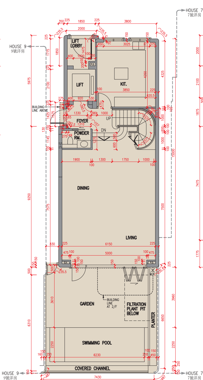
地下平面圖 G/F Plan
