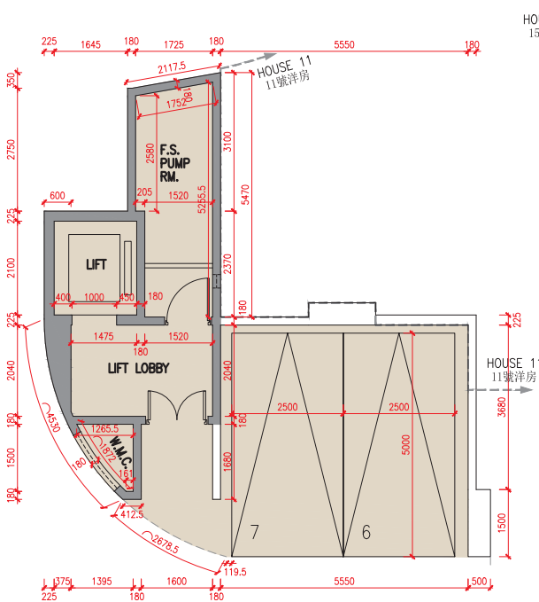
地庫平面圖 B/F Plan
