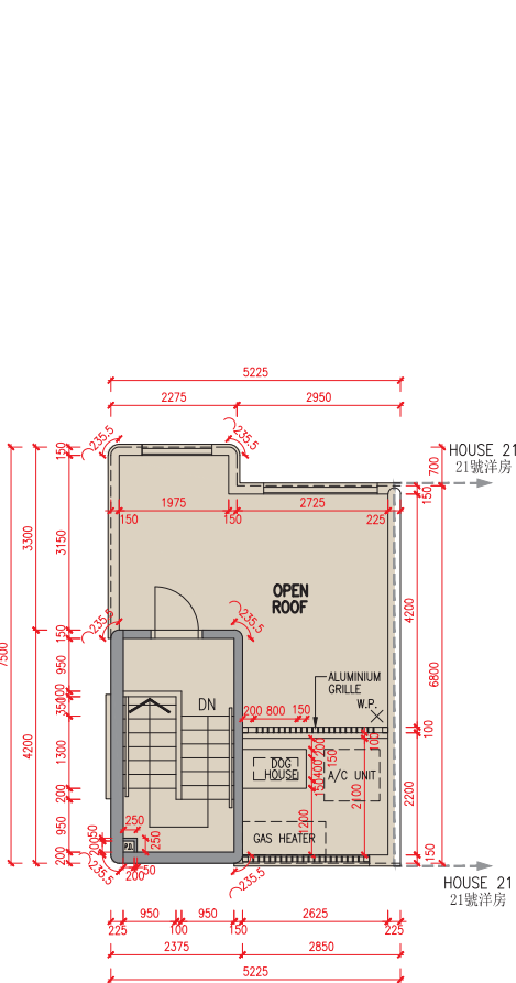
天台平面圖 Roof Plan
