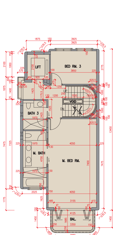
2樓平面圖 2/F Plan
