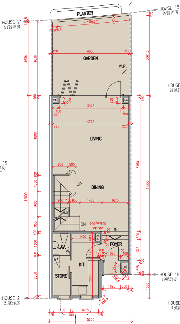
地下平面圖 G/F Plan
