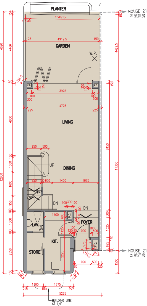
地下平面圖 G/F Plan
