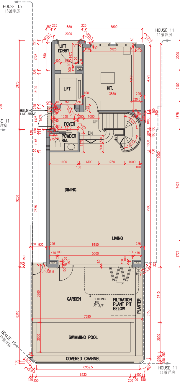
地下平面圖 G/F Plan
