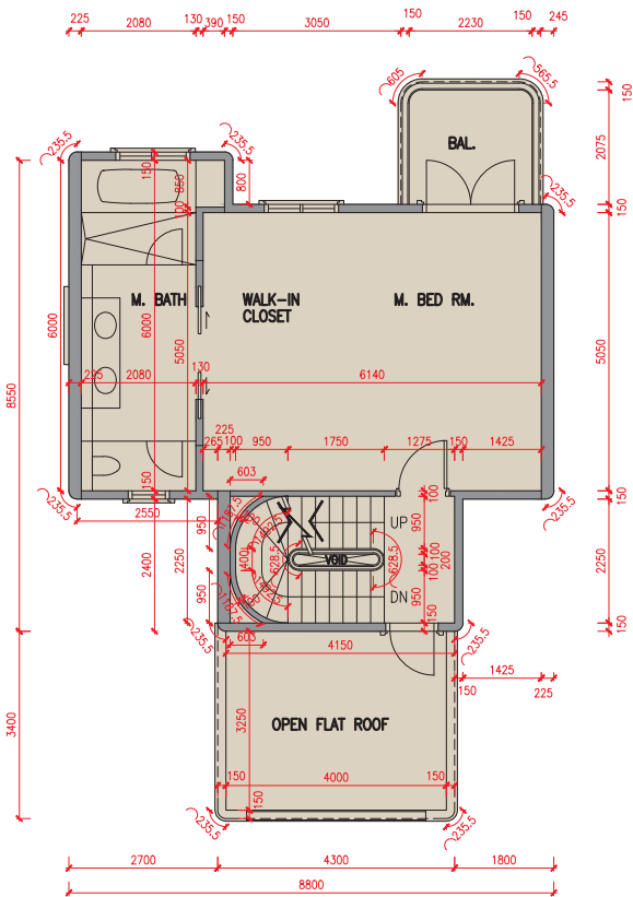
2樓平面圖 2/F Plan
