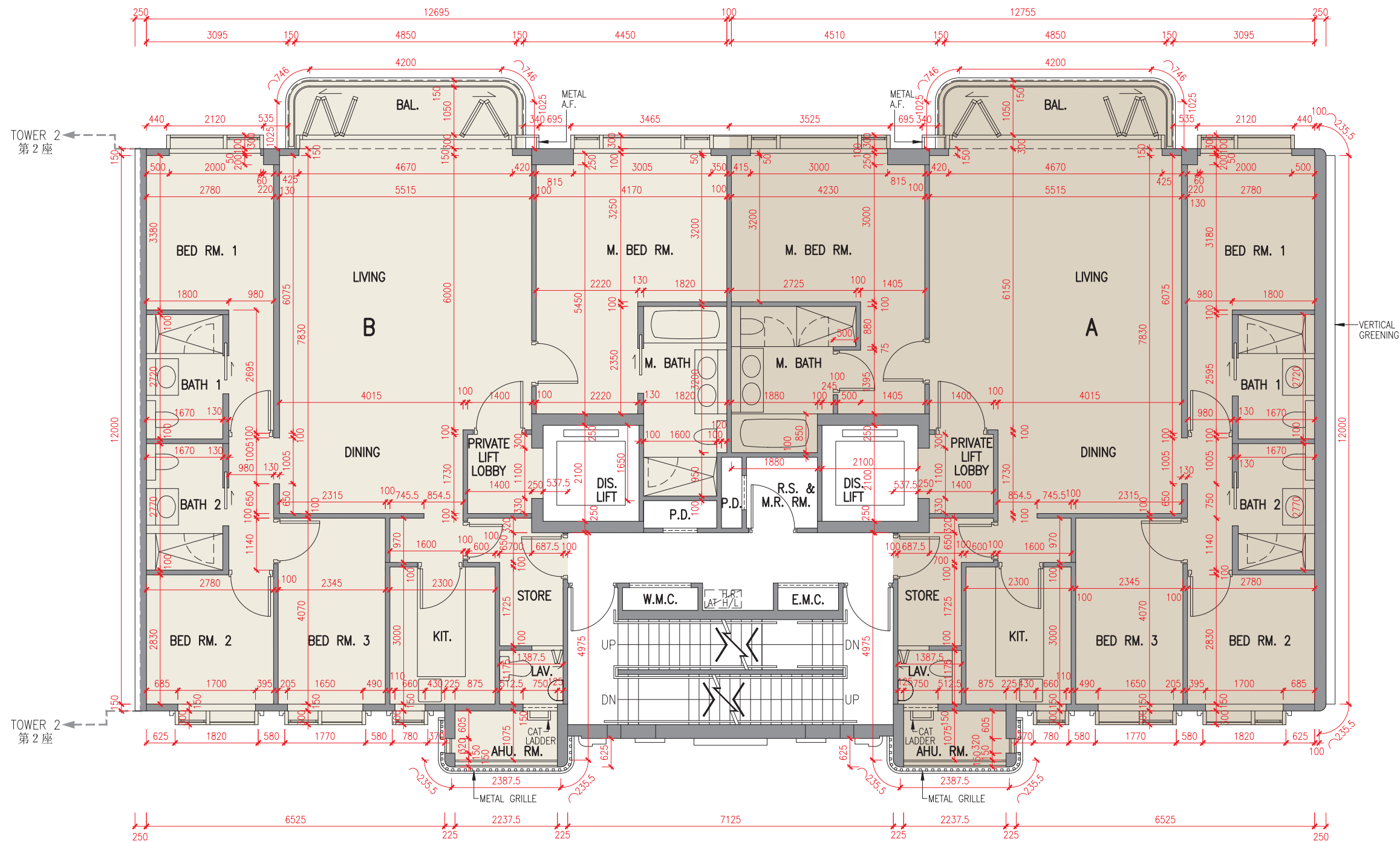
3樓平面圖 3/F Plan
