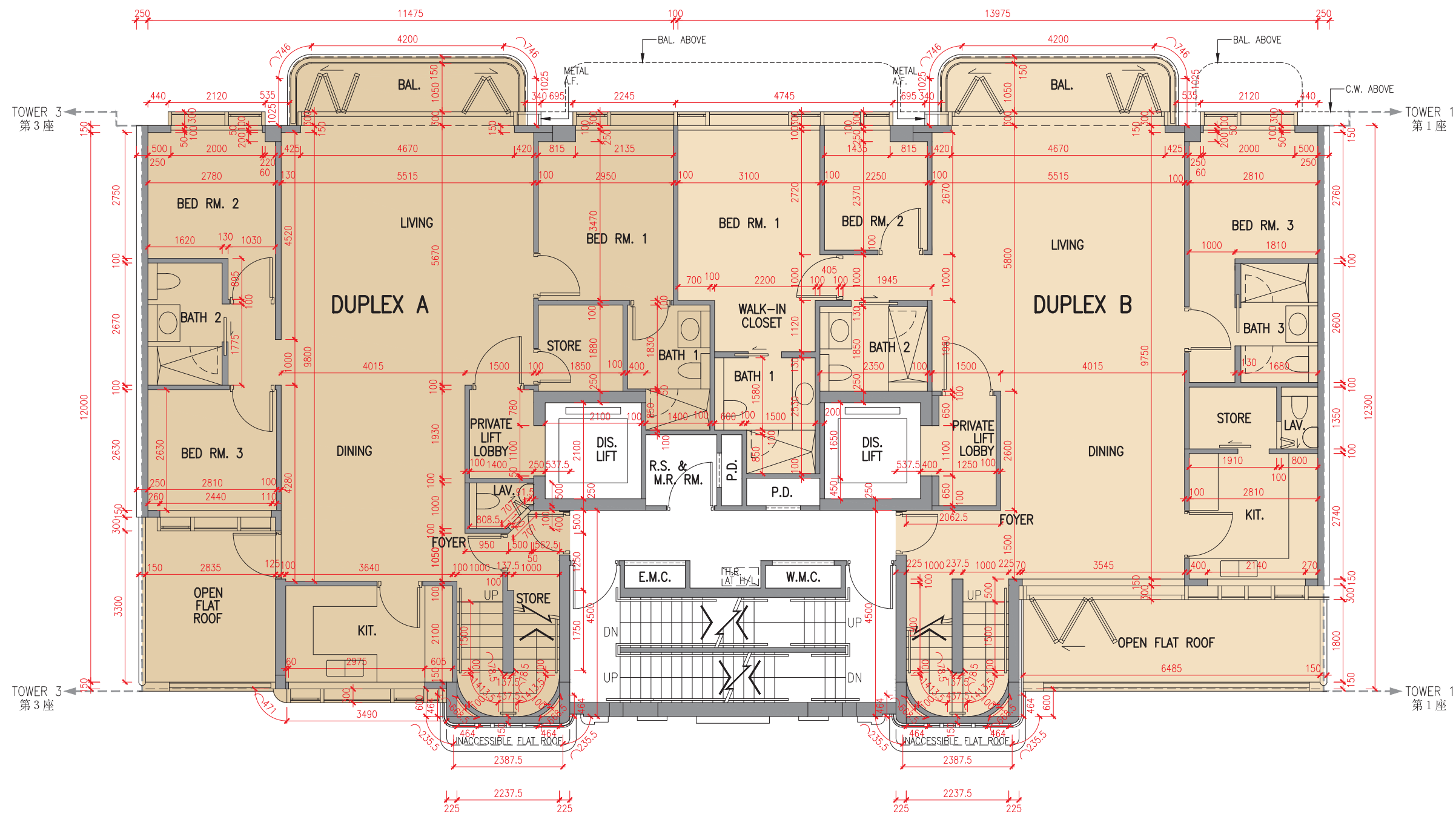
5樓平面圖 5/F Plan
