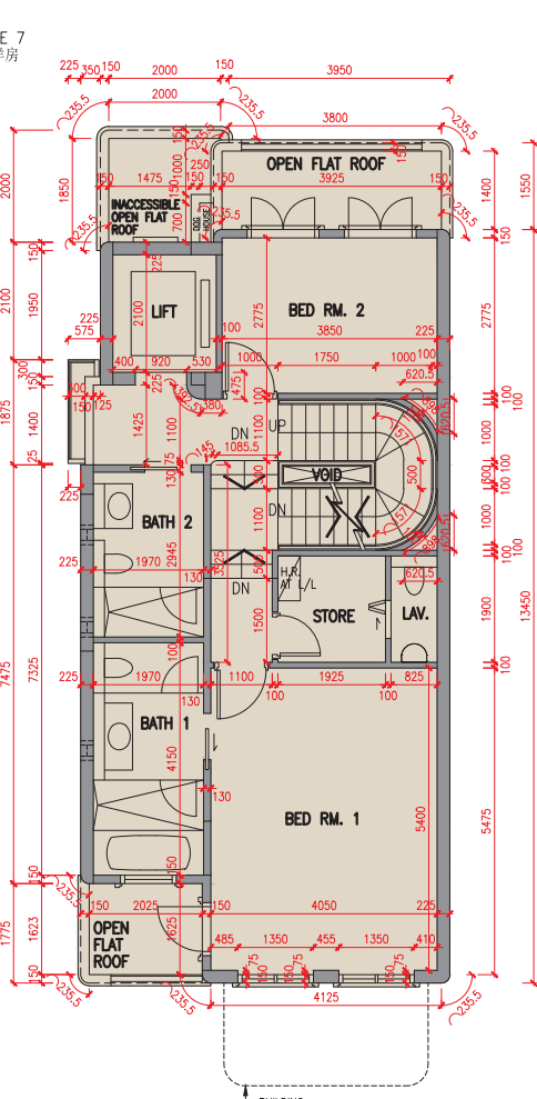
1樓平面圖 1/F Plan
