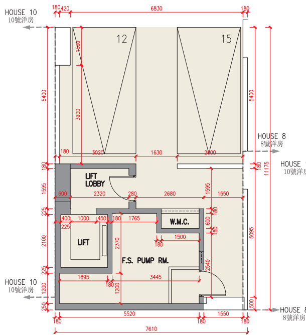
地庫平面圖 B/F Plan
