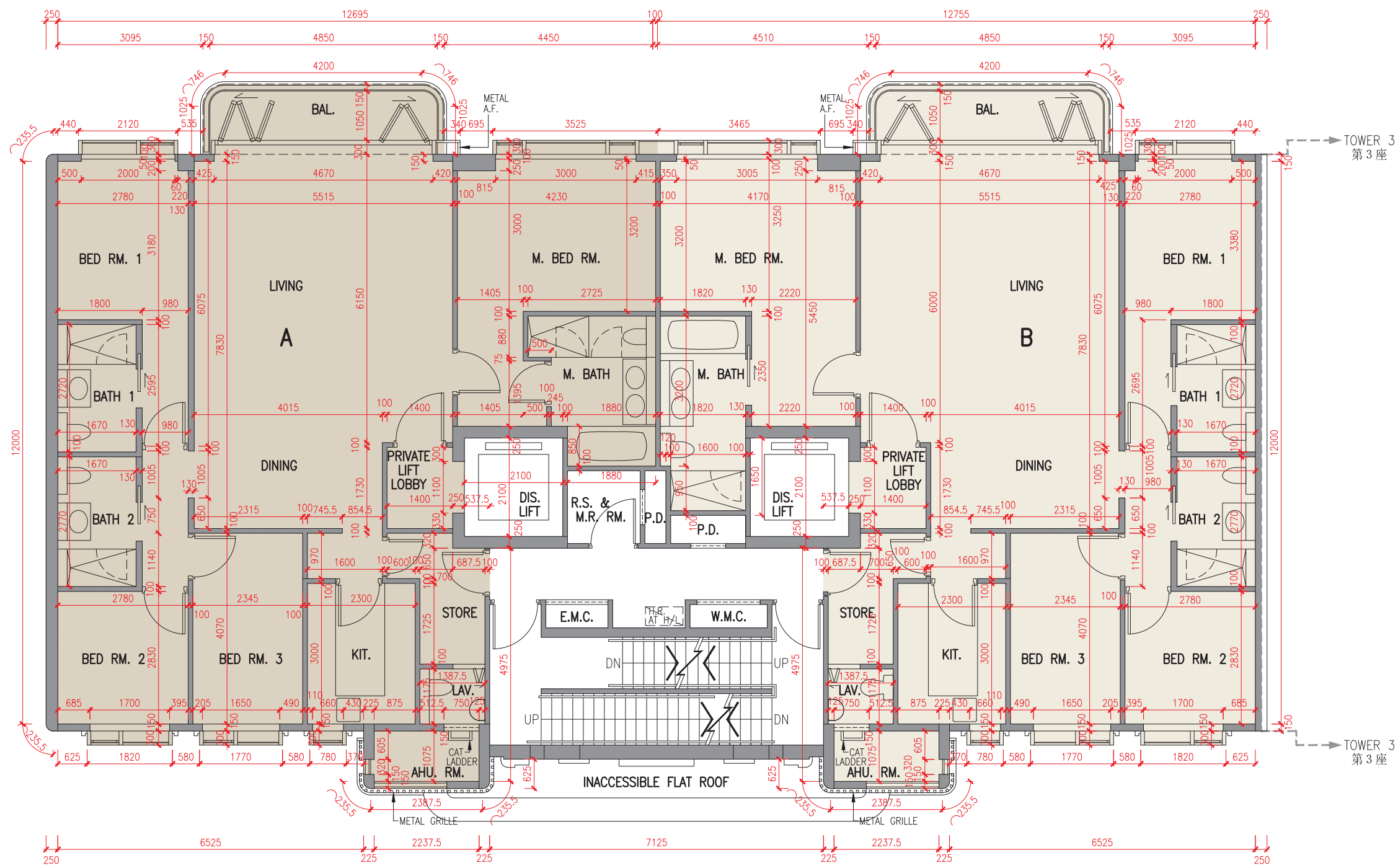
2樓平面圖 2/F Plan
