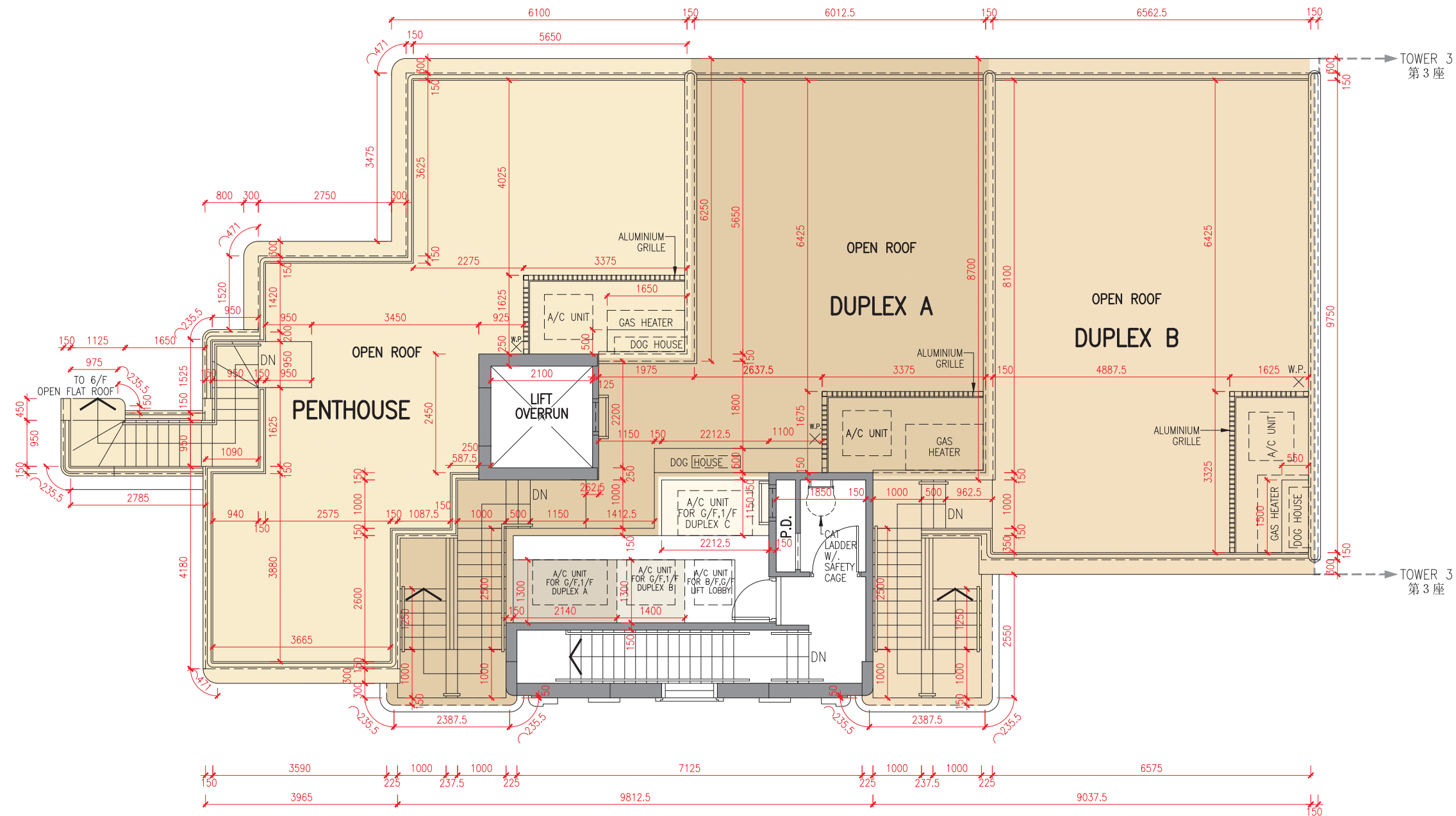
天台平面圖 Roof Plan
