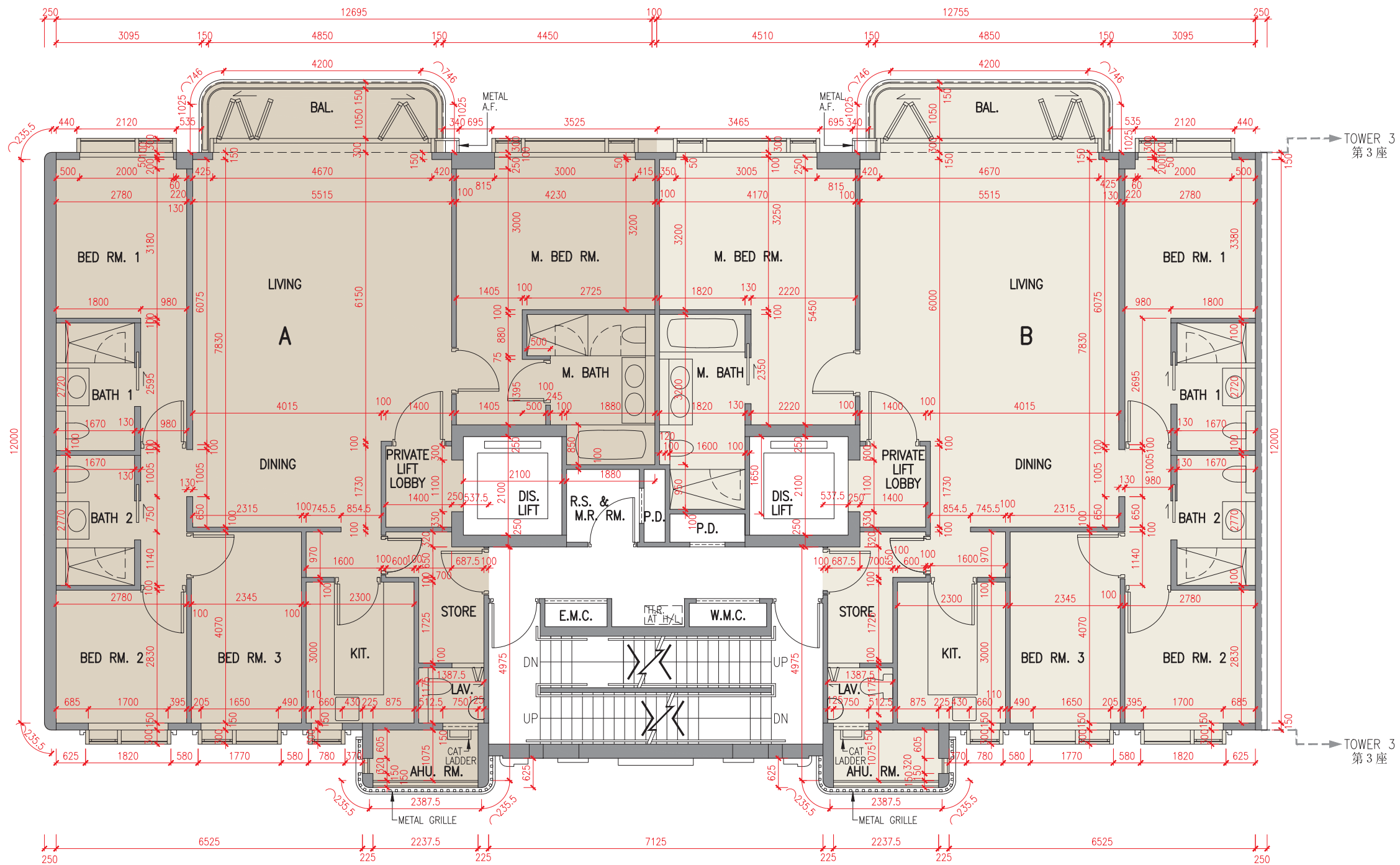
3樓平面圖 3/F Plan
