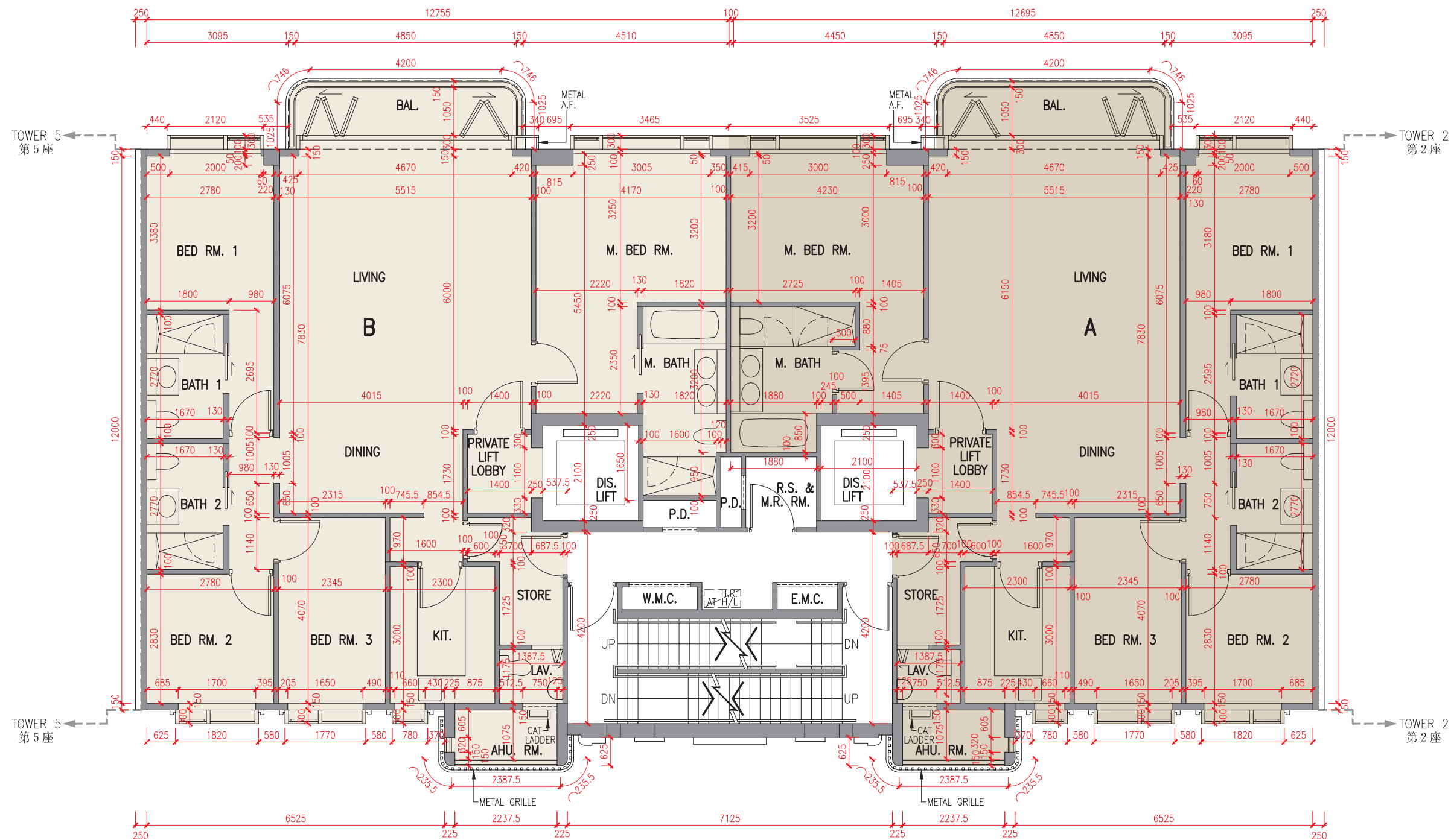
3樓平面圖 3/F Plan
