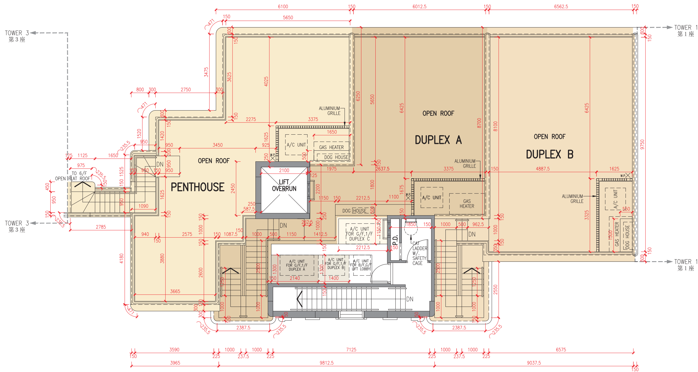
天台平面圖 Roof Plan
