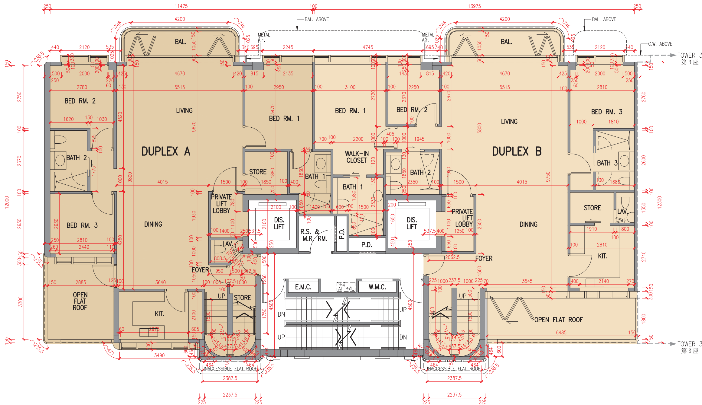
5樓平面圖 5/F Plan
