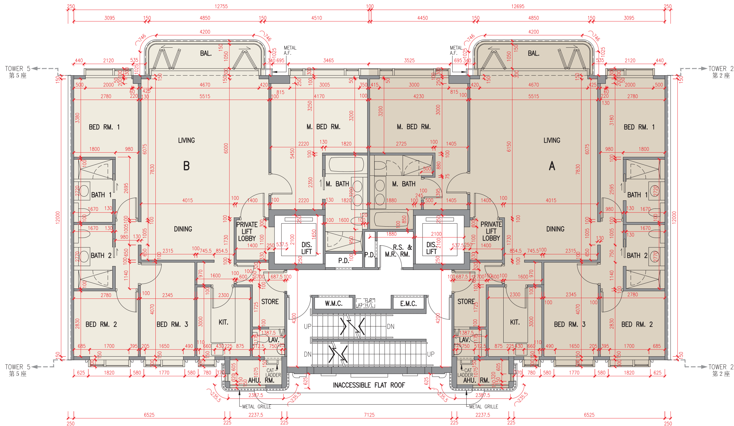
2樓平面圖 2/F Plan
