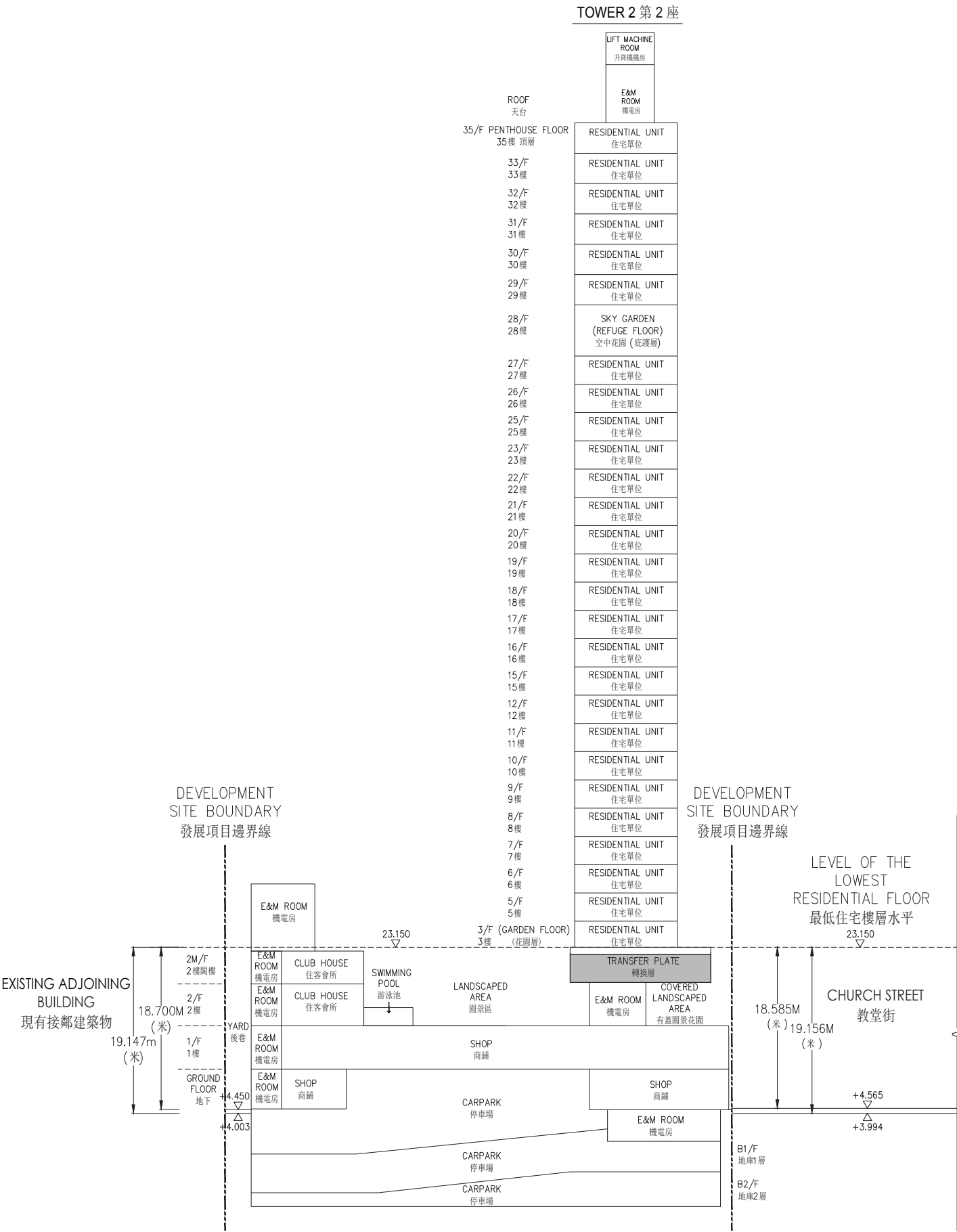
CROSS-SECTION PLAN SECTION B 橫截面圖 B 部份
