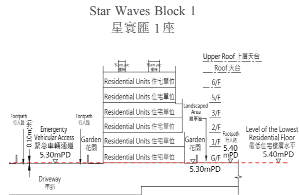
Cross Section Plan K-K 橫截面圖 K-K
