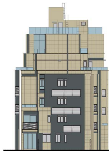
Elevation D 立面圖D
