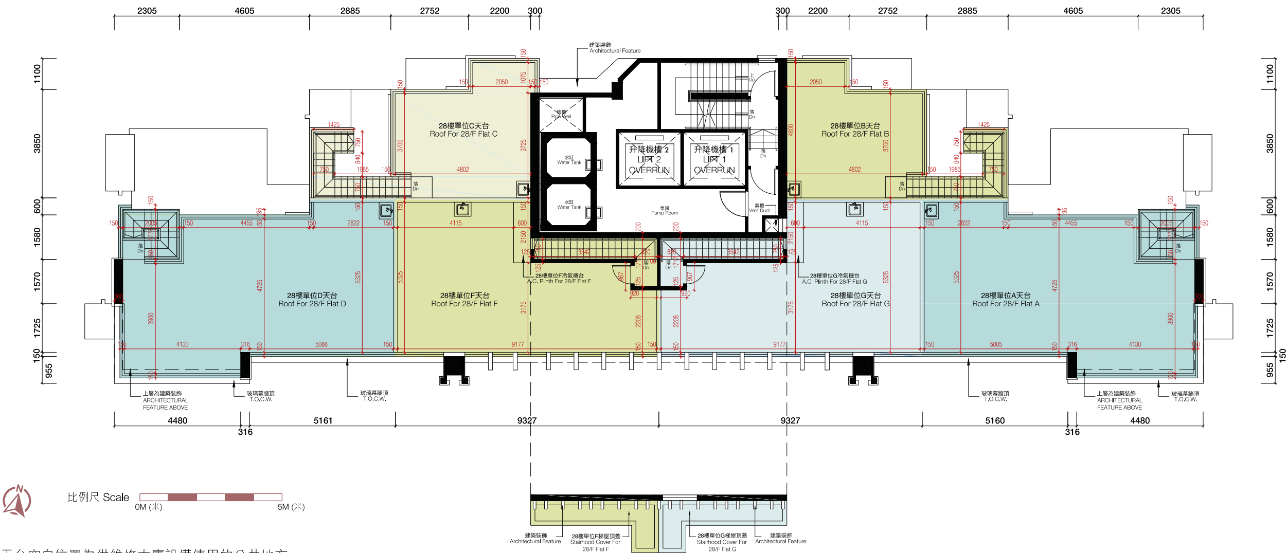
天台平面圖 Roof Floor Plan
