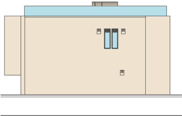
ELEVATION 4 立面圖 4
