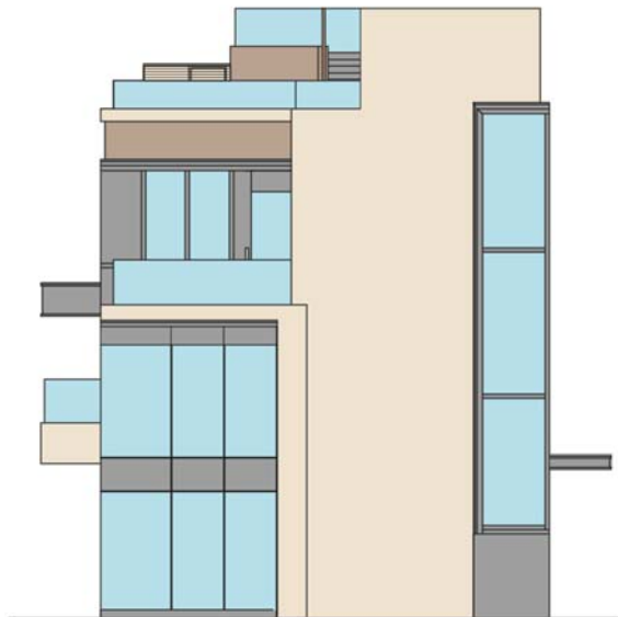
ELEVATION 4 立面圖 4
