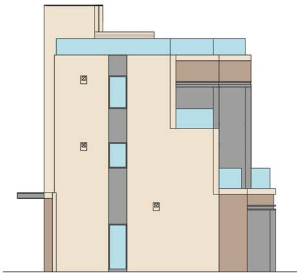
ELEVATION 2 立面圖 2
