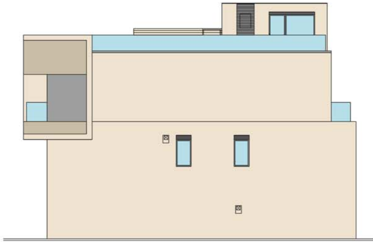
ELEVATION 4 立面圖 4
