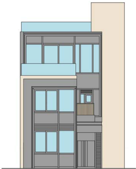
ELEVATION 3 立面圖 3
