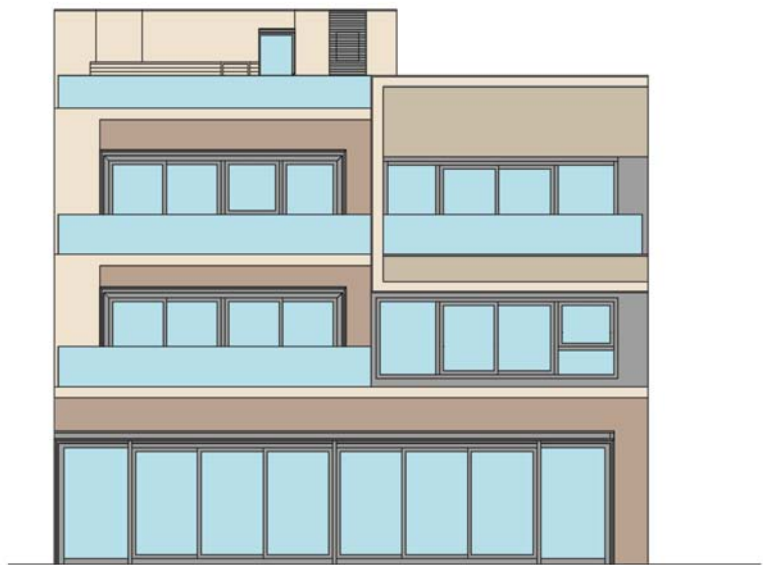
ELEVATION 1 立面圖 1
