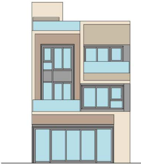
ELEVATION 1 立面圖 1
