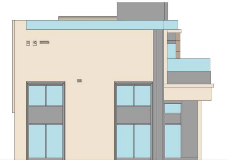
ELEVATION 2 立面圖 2
