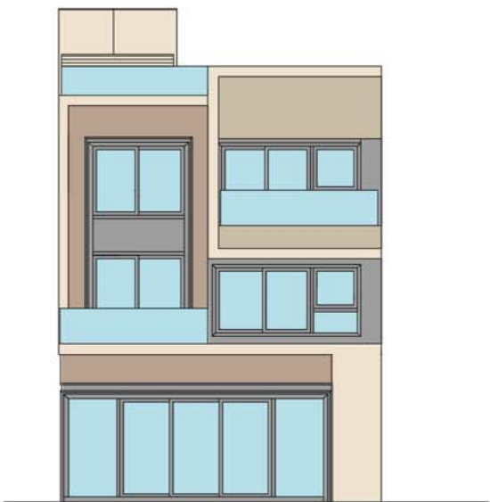
ELEVATION 1 立面圖 1
