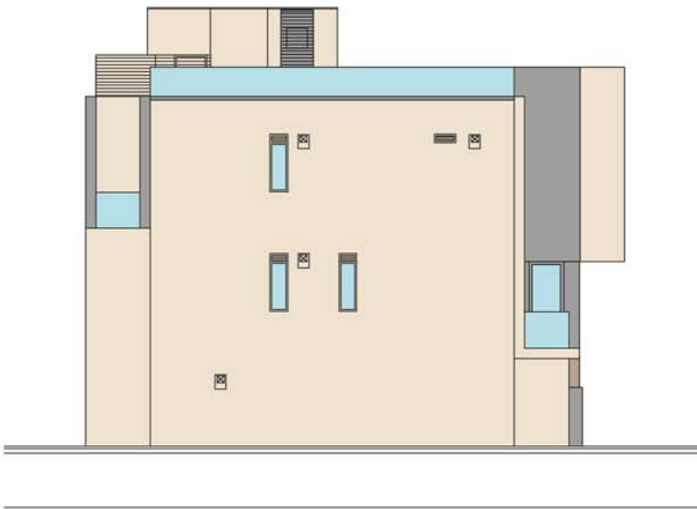
ELEVATION 2 立面圖 2
