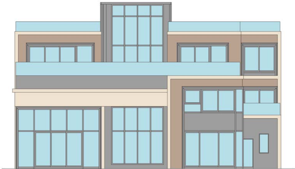
ELEVATION 1 立面圖 1
