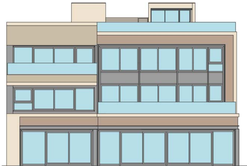
ELEVATION 1 立面圖 1
