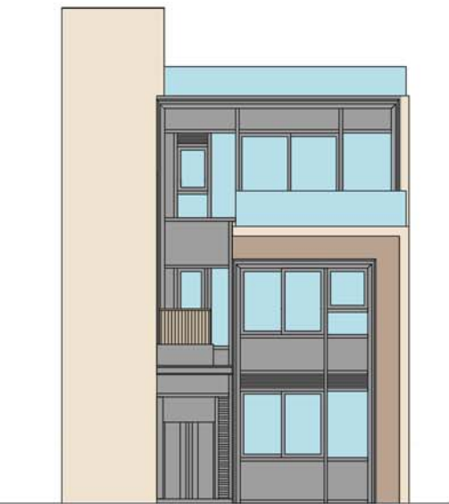
ELEVATION 3 立面圖 3
