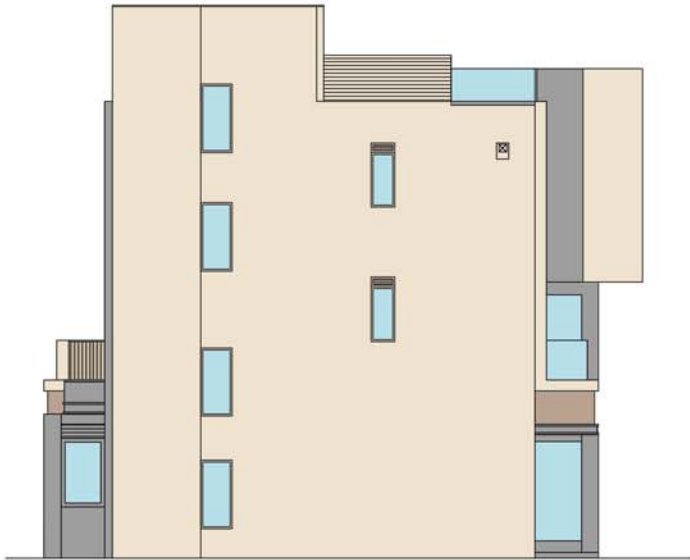
ELEVATION 2 立面圖 2
