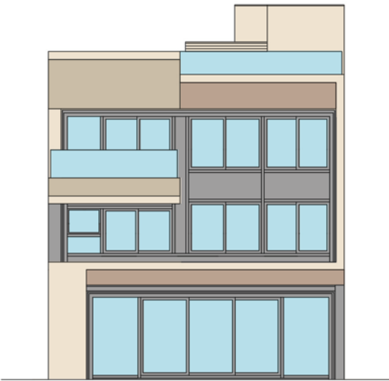
ELEVATION 1 立面圖 1
