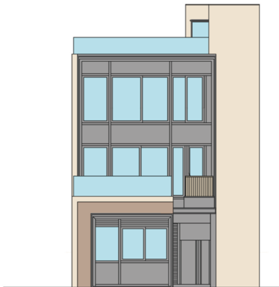
ELEVATION 3 立面圖 3
