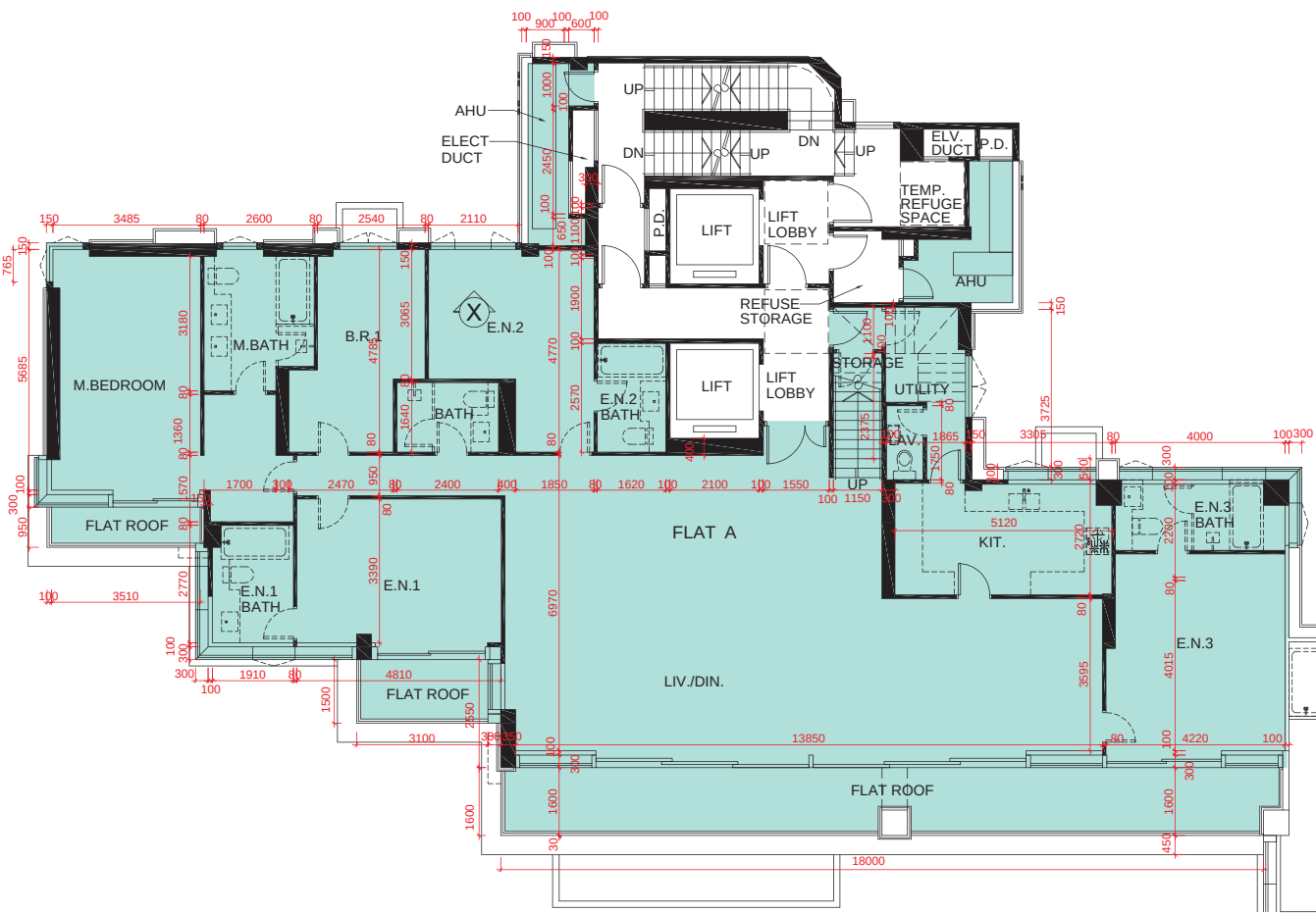
15/F PLAN 15樓平面圖
