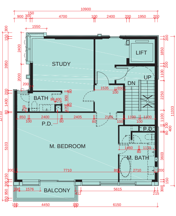
2/F PLAN 2樓平面圖
