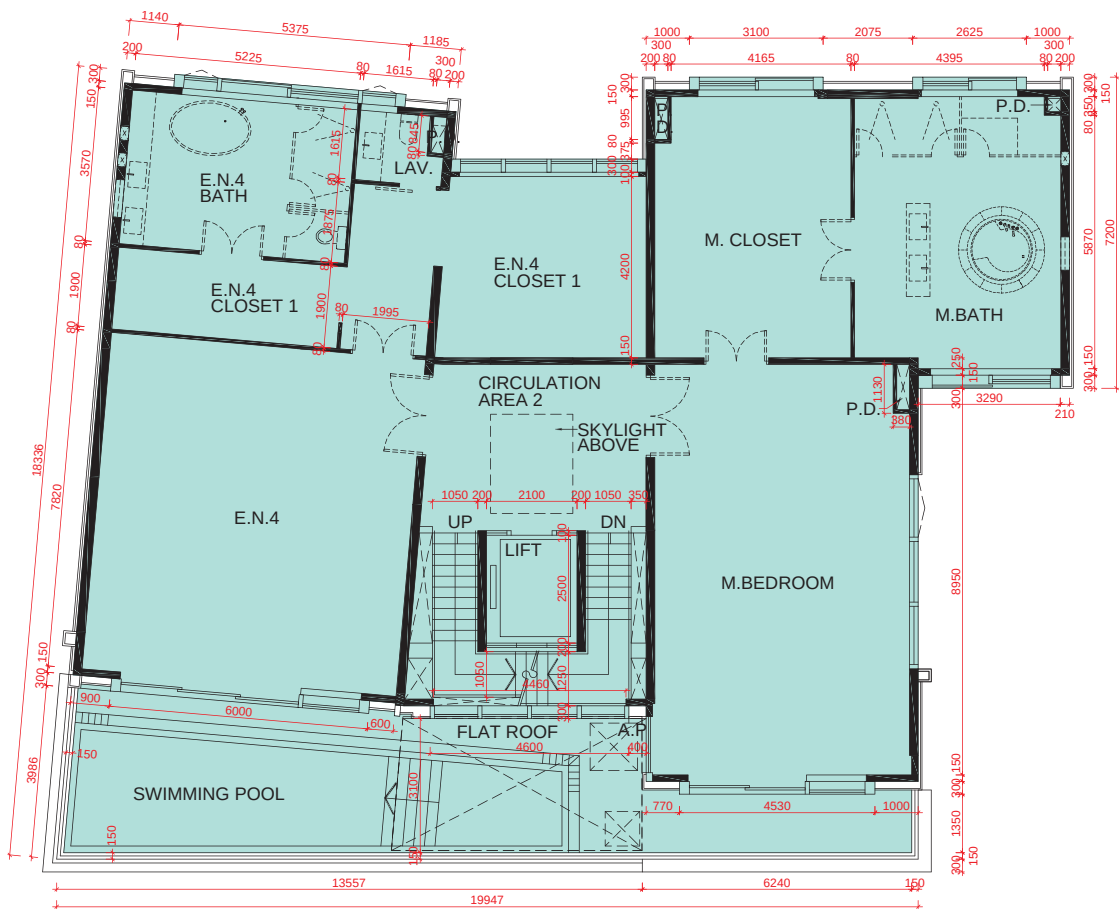
2/F PLAN 2樓平面圖
