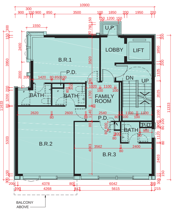
1/F PLAN 1樓平面圖
