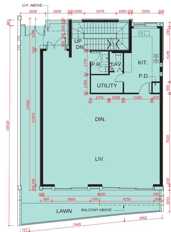
G/F PLAN 地面層平面圖
