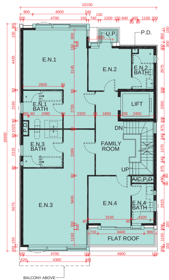
1/F PLAN 1樓平面圖
