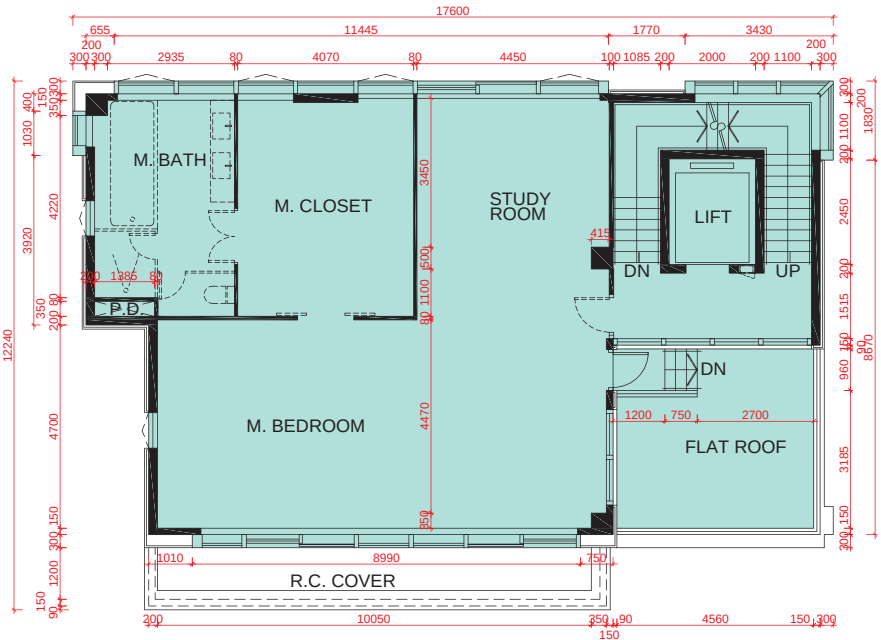
2/F PLAN 2樓平面圖
