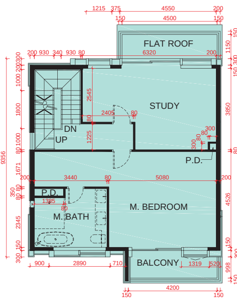
2/F PLAN 2樓平面圖
