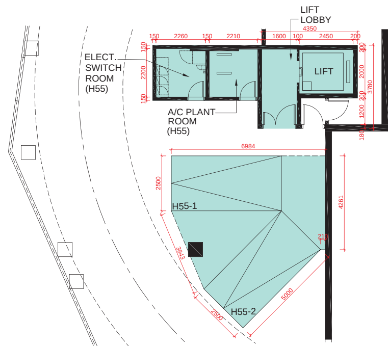
B/F PLAN 地庫層平面圖
