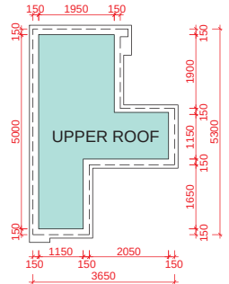
UPPER ROOF PLAN 上層天台平面圖
