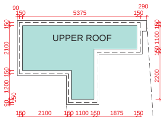
UPPER ROOF PLAN 上層天台平面圖
