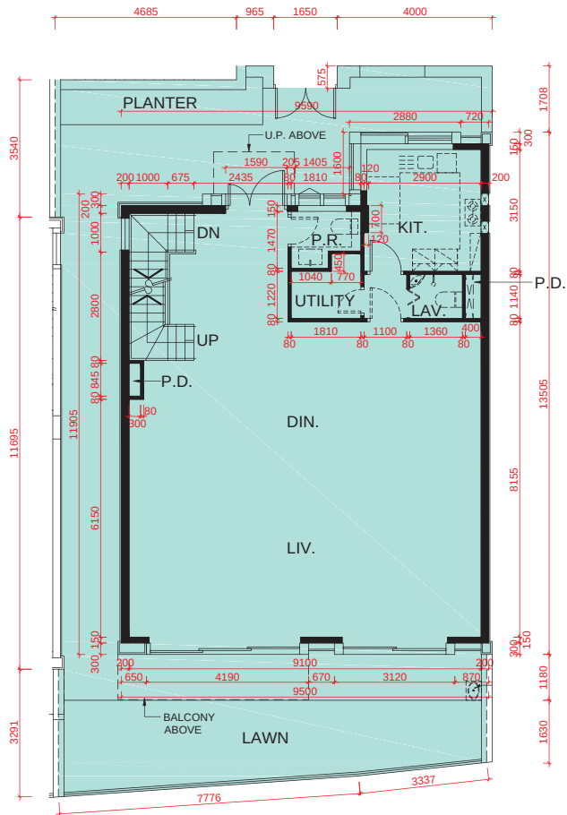
G/F PLAN 地面層平面圖
