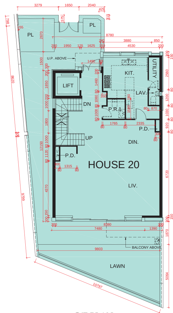
G/F PLAN 地面層平面圖
