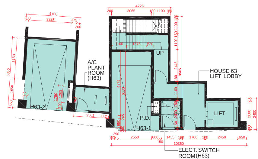
B/F PLAN 地庫層平面圖
