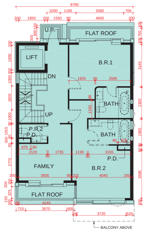
1/F PLAN 1樓平面圖
