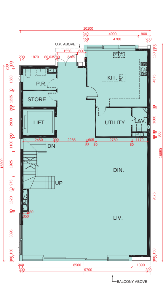
G/F PLAN 地面層平面圖
