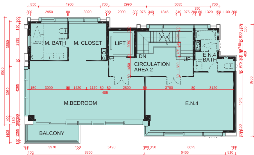
2/F PLAN 2樓平面圖
