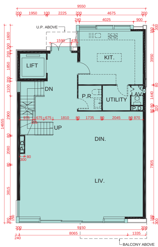
G/F PLAN 地面層平面圖
