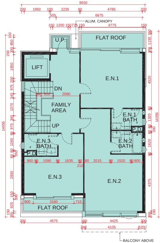
1/F PLAN 1樓平面圖
