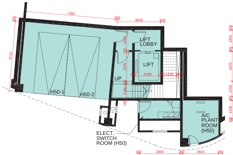
B/F PLAN 地庫層平面圖
