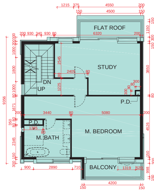
2/F PLAN 2樓平面圖
