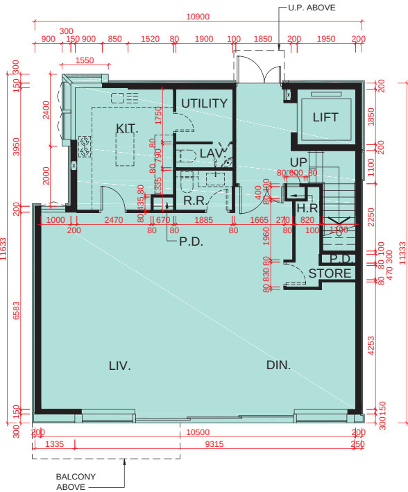
G/F PLAN 地面層平面圖
