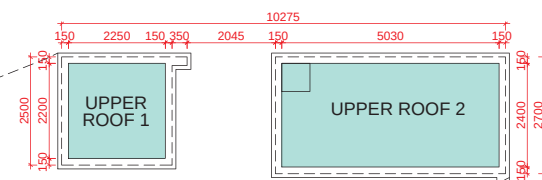
UPPER ROOF PLAN 上層天台平面圖
