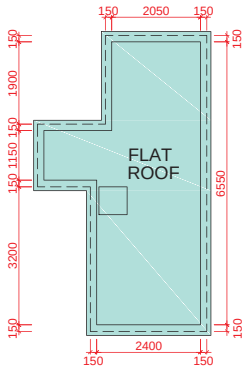
UPPER ROOF PLAN 上層天台平面圖
