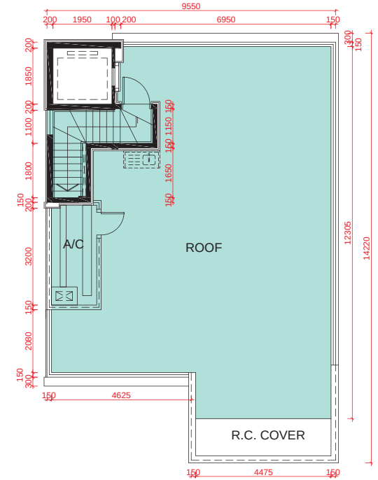
ROOF PLAN 天台平面圖
