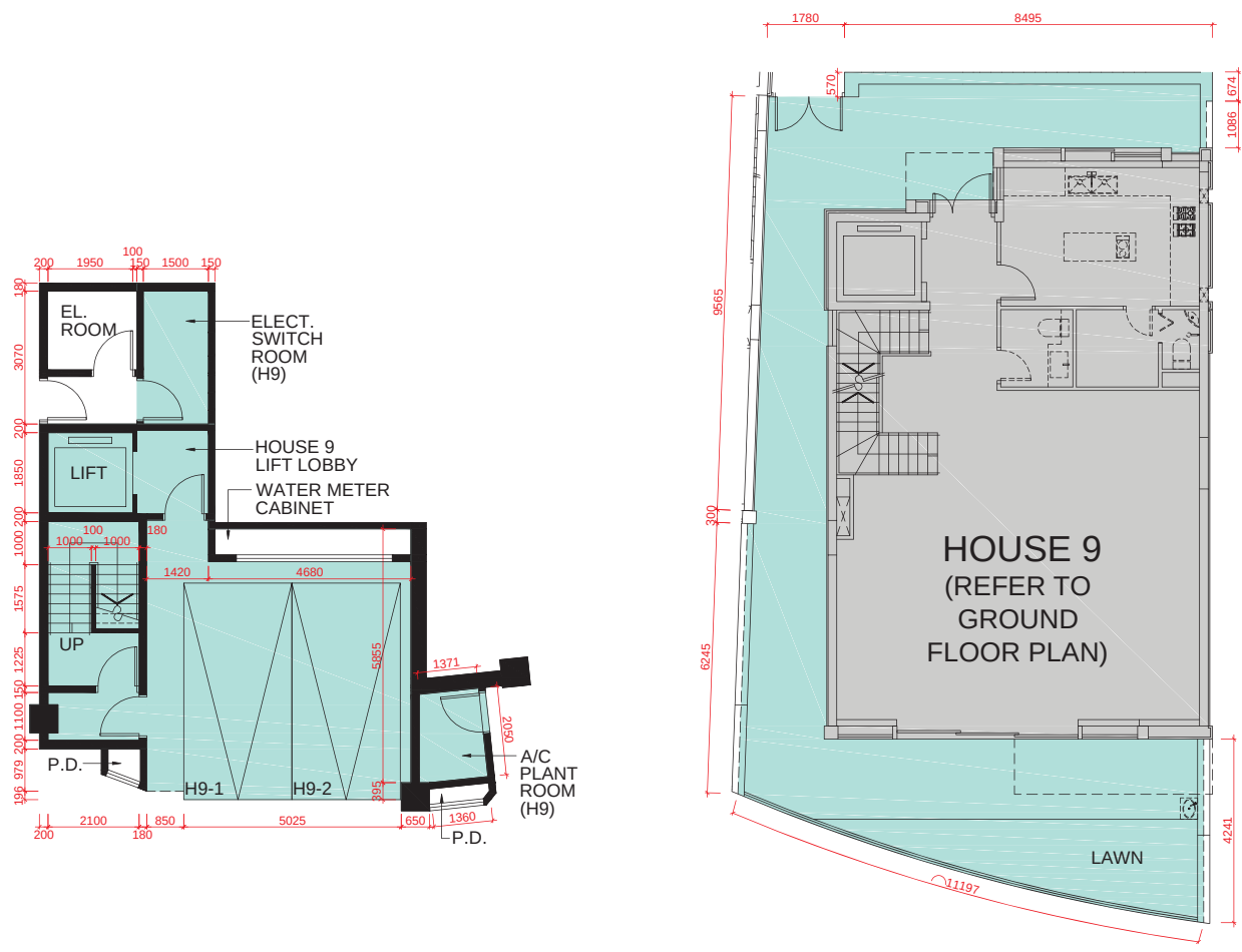
B/F PLAN 地庫層平面圖
