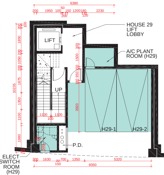
B/F PLAN 地庫層平面圖
