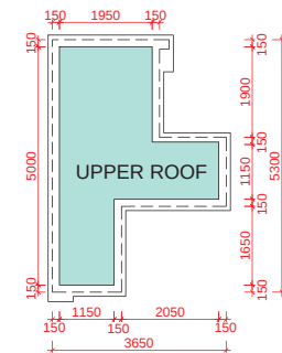
UPPER ROOF PLAN 上層天台平面圖
