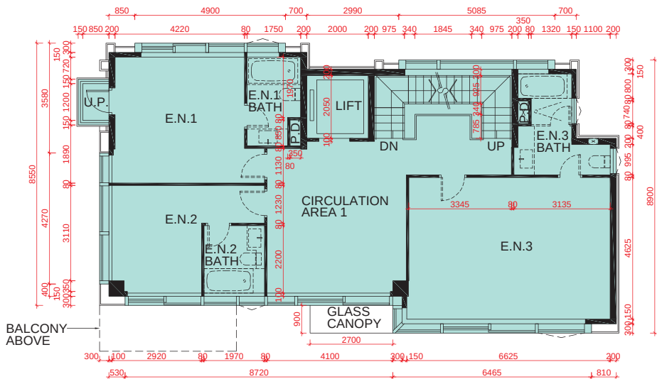
1/F PLAN 1樓平面圖
