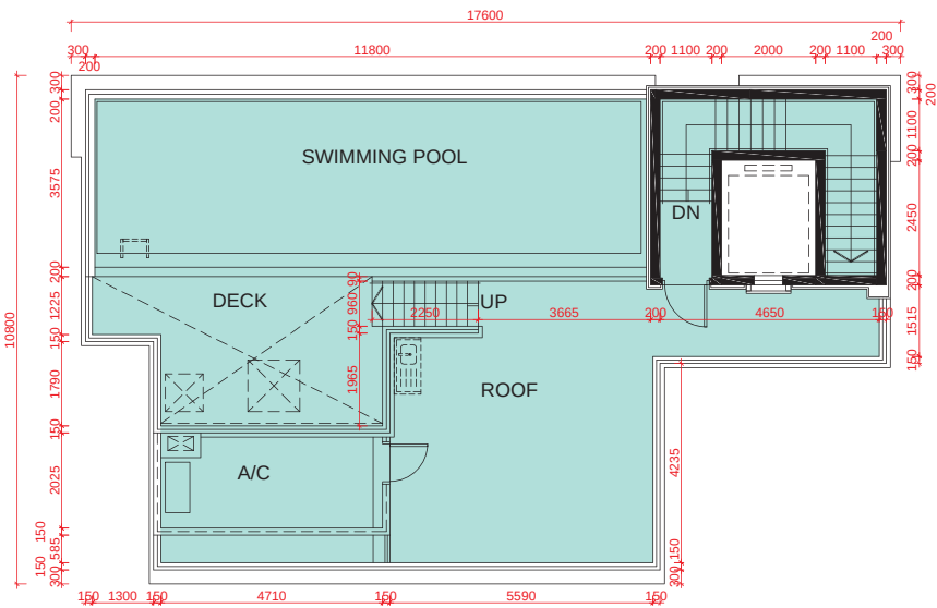
UPPER ROOF PLAN 上層天台平面圖
