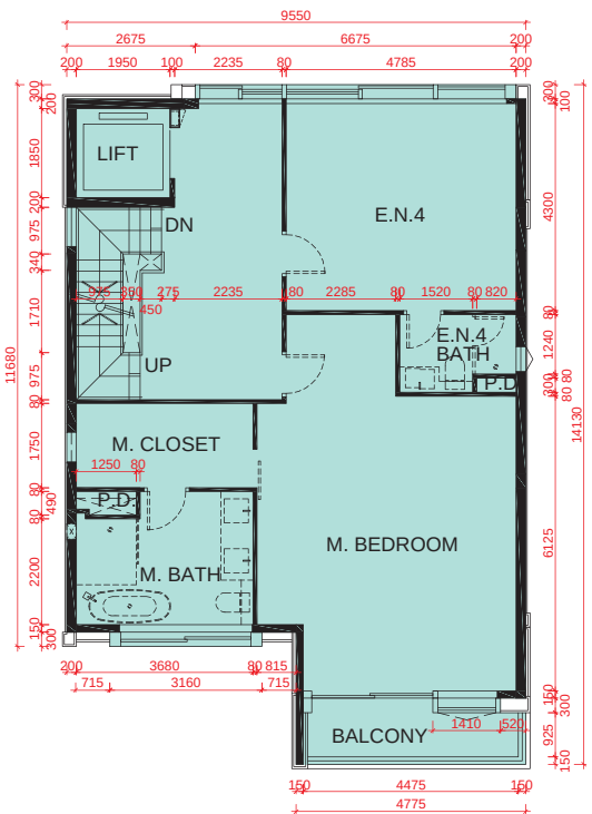
2/F PLAN 2樓平面圖
