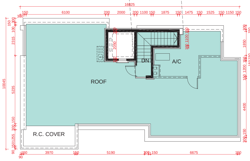
ROOF PLAN 天台平面圖
