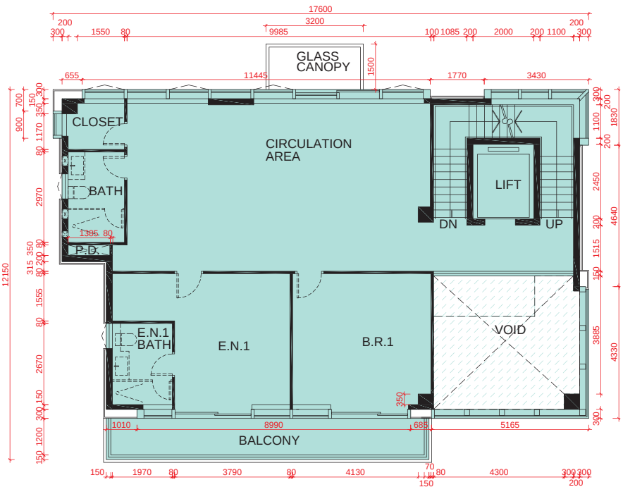
1/F PLAN 1樓平面圖
