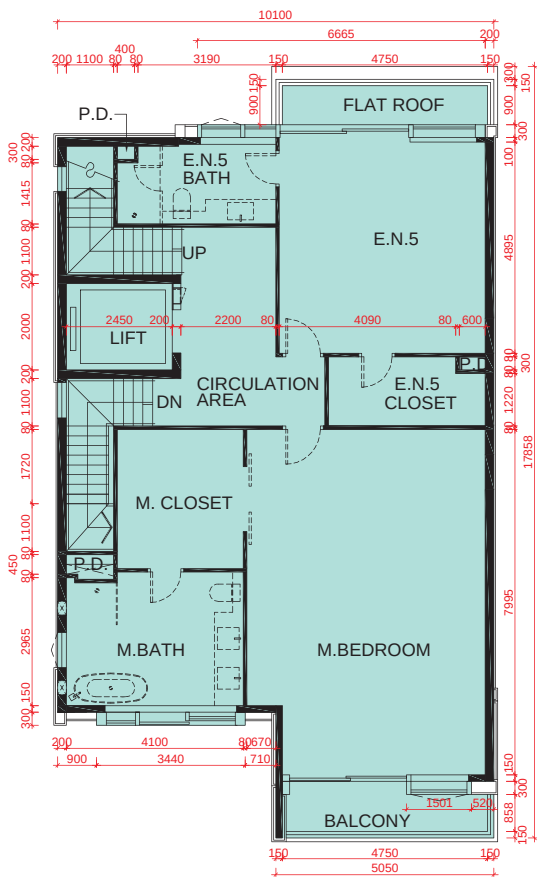
2/F PLAN 2樓平面圖
