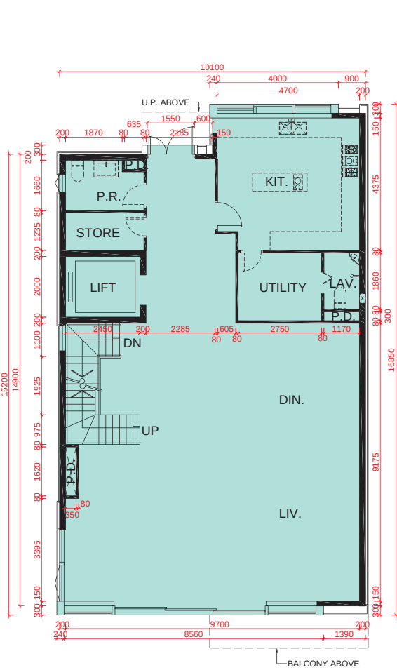
G/F PLAN 地面層平面圖
