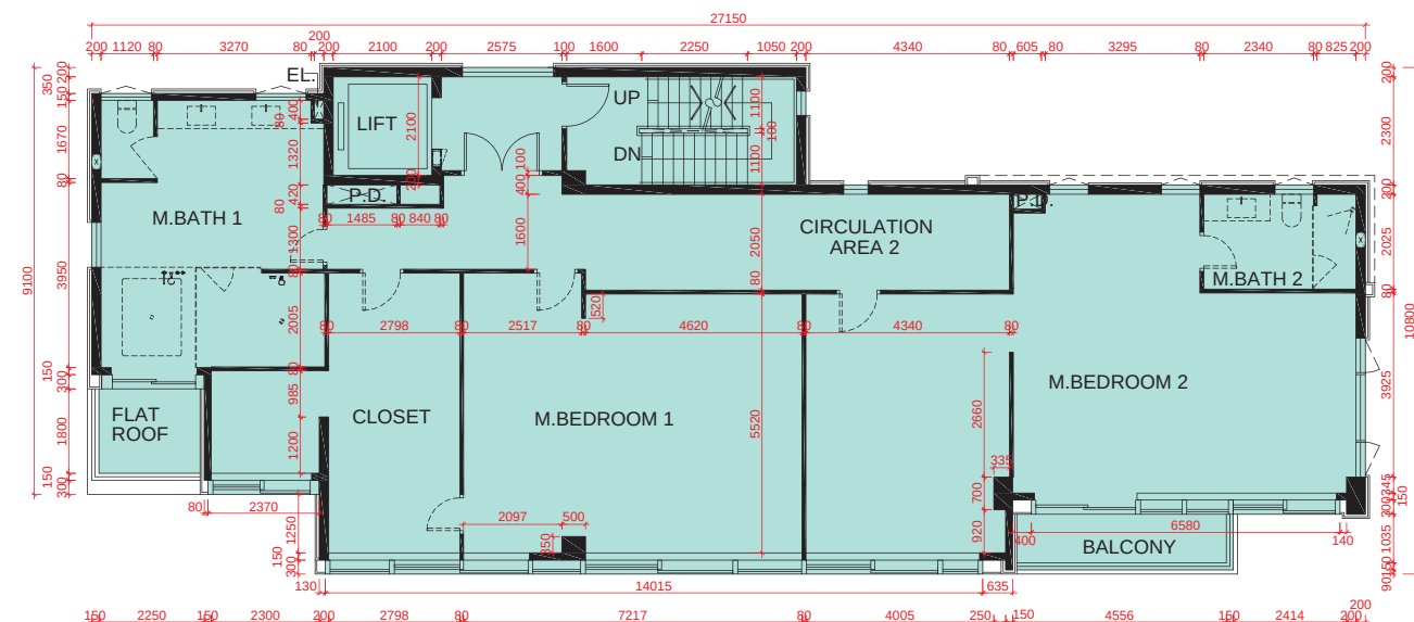
2/F PLAN 2樓平面圖
