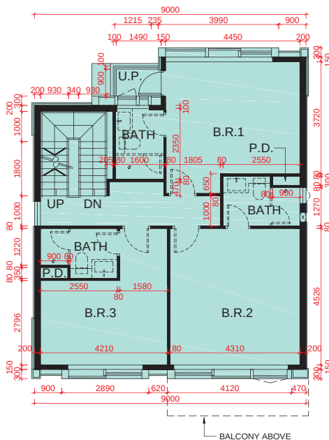
1/F PLAN 1樓平面圖
