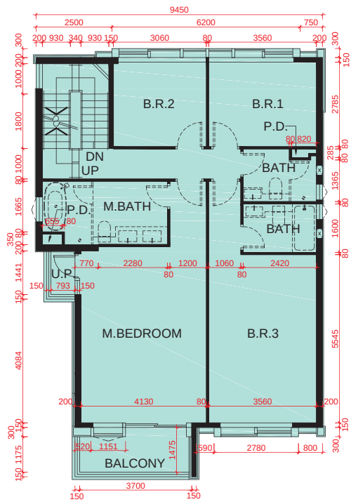
1/F PLAN 1樓平面圖
