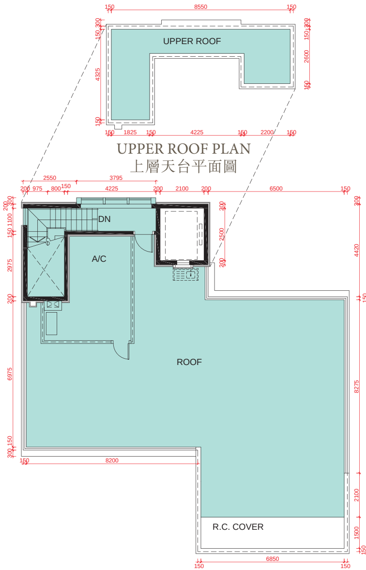
ROOF PLAN 天台平面圖
