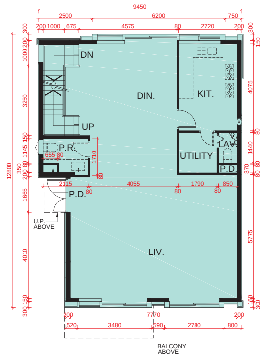
G/F PLAN 地面層平面圖
