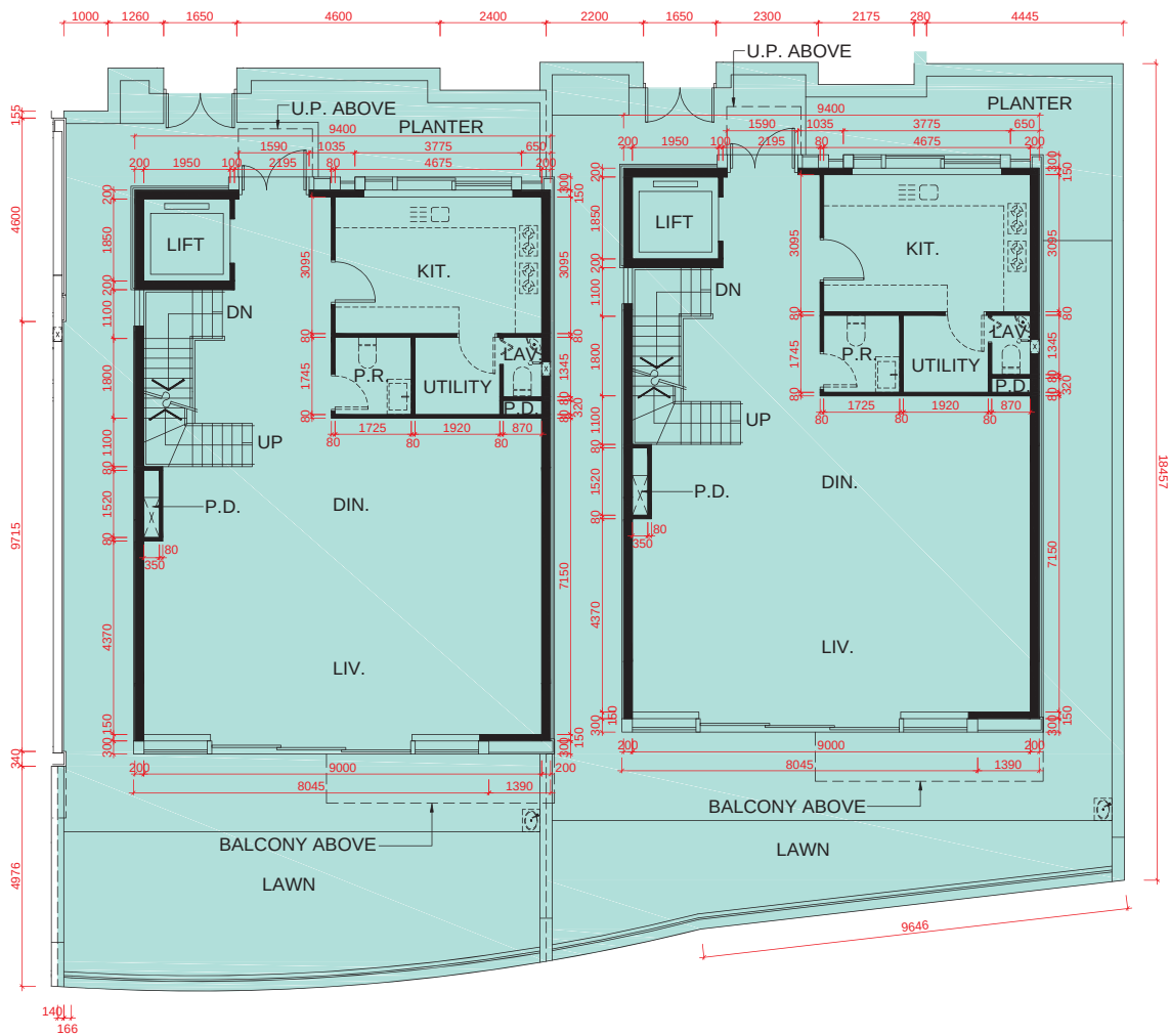
HOUSE 30 G/F PLAN 洋房30號地面層平面圖
