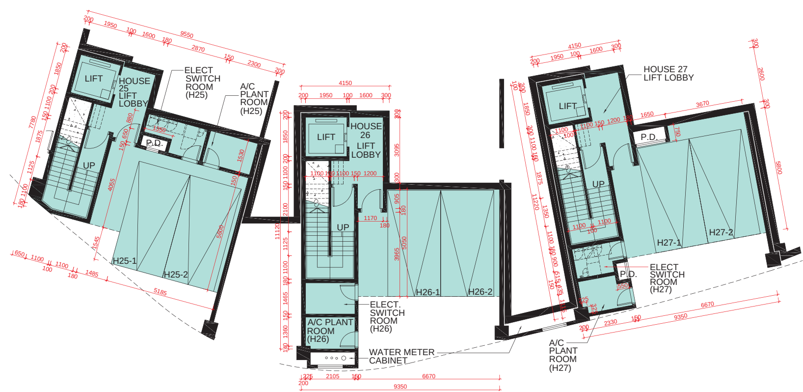
B/F PLAN 地庫層平面圖
