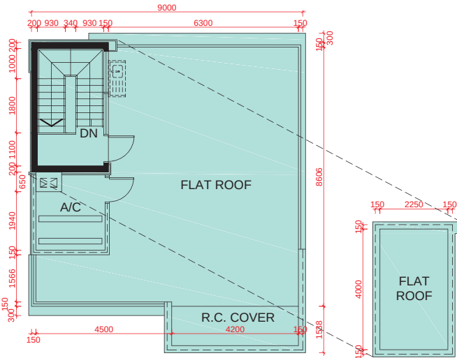
UPPER ROOF PLAN 上層天台平面圖
