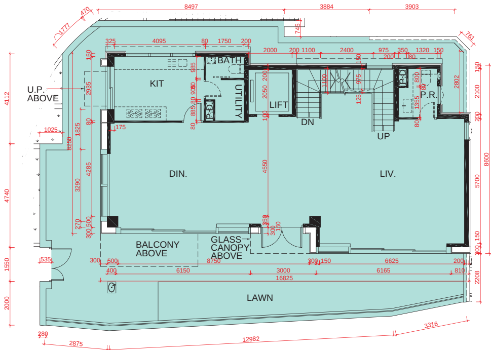
G/F PLAN 地面層平面圖
