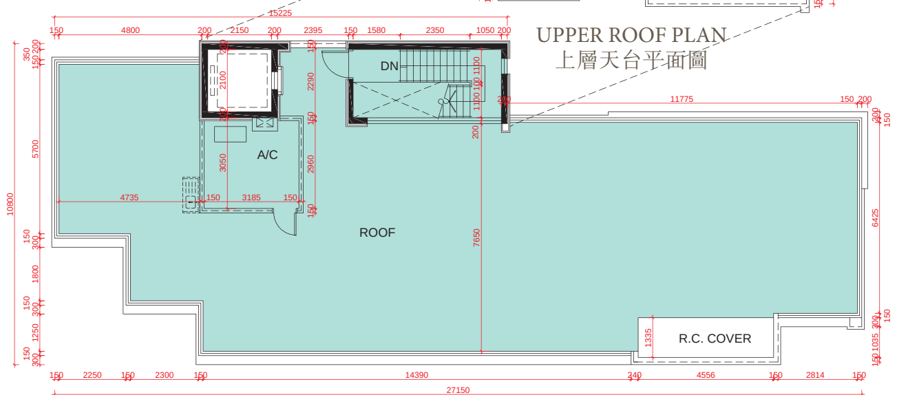
ROOF PLAN 天台平面圖
