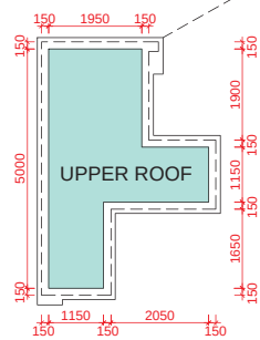
UPPER ROOF PLAN 上層天台平面圖
