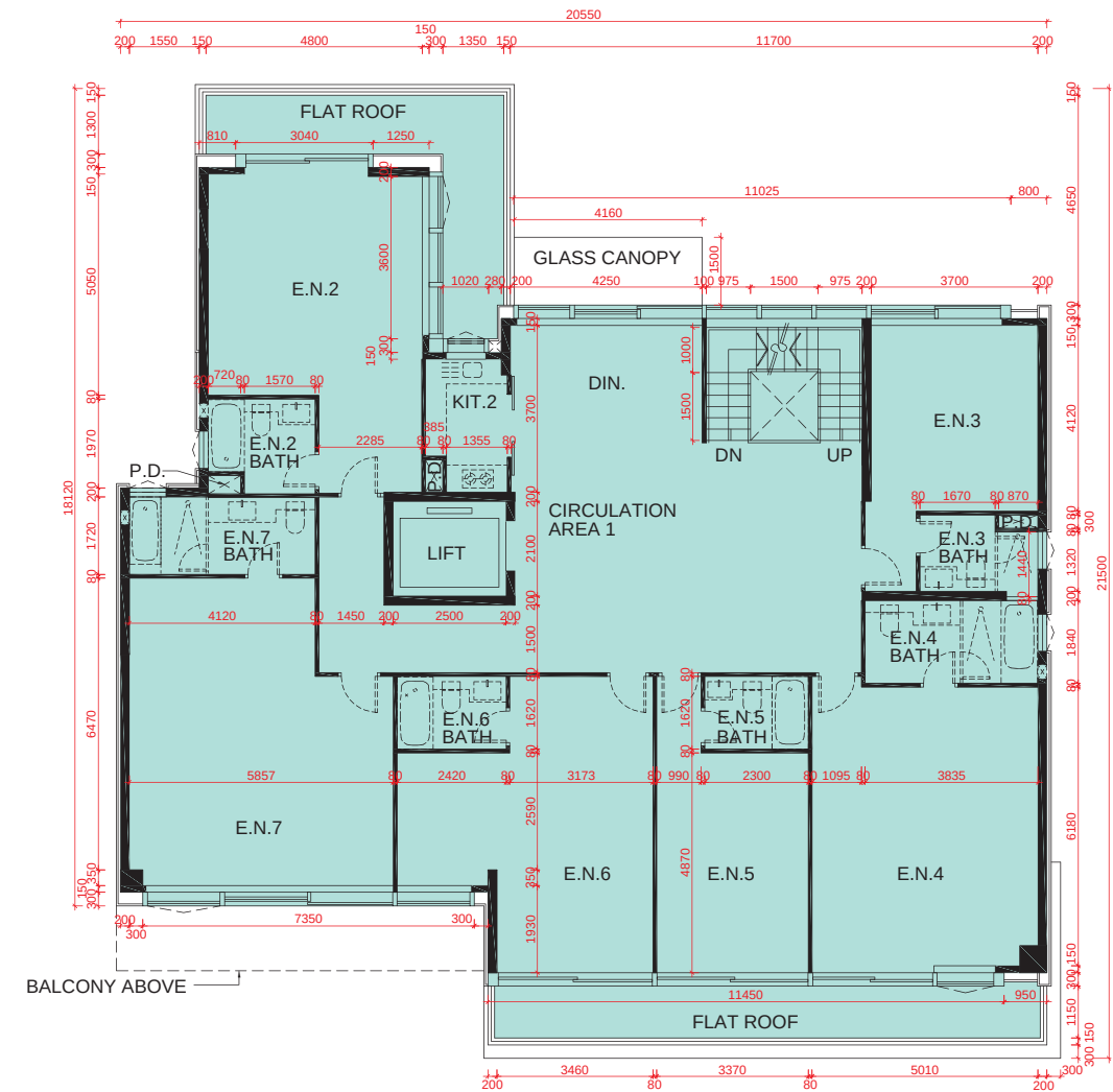
1/F PLAN 1樓平面圖
