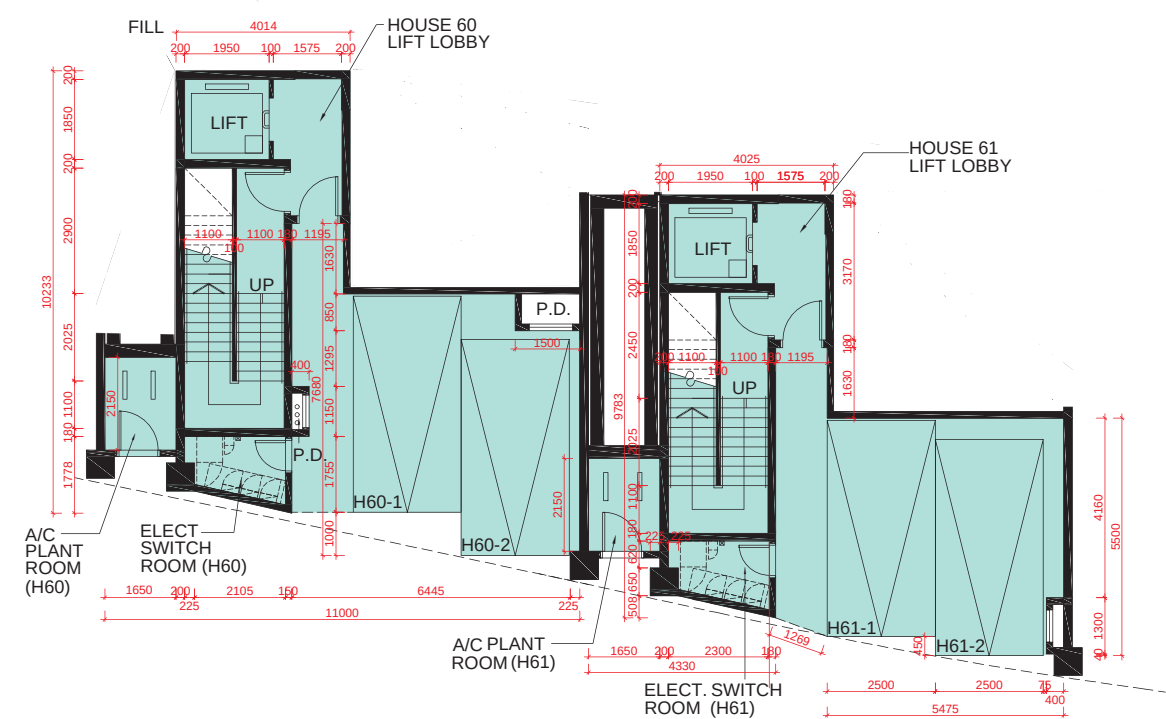
B/F PLAN 地庫層平面圖
