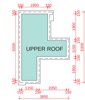
UPPER ROOF PLAN 上層天台平面圖
