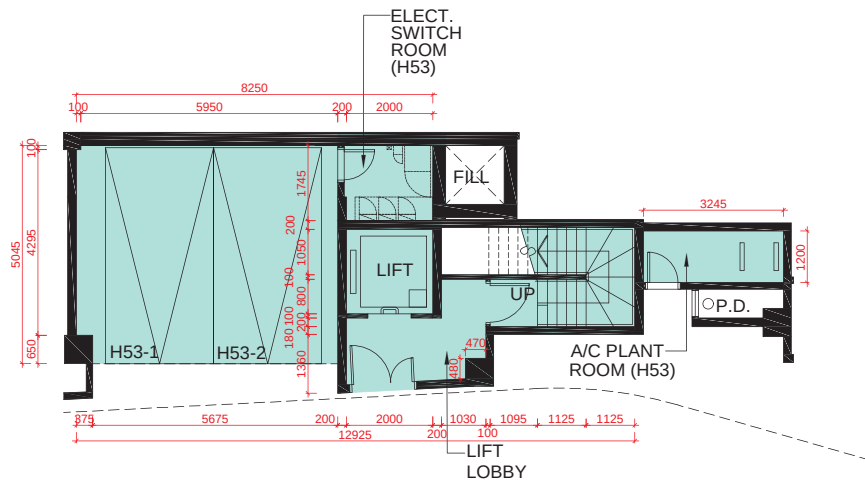
B/F PLAN 地庫層平面圖
