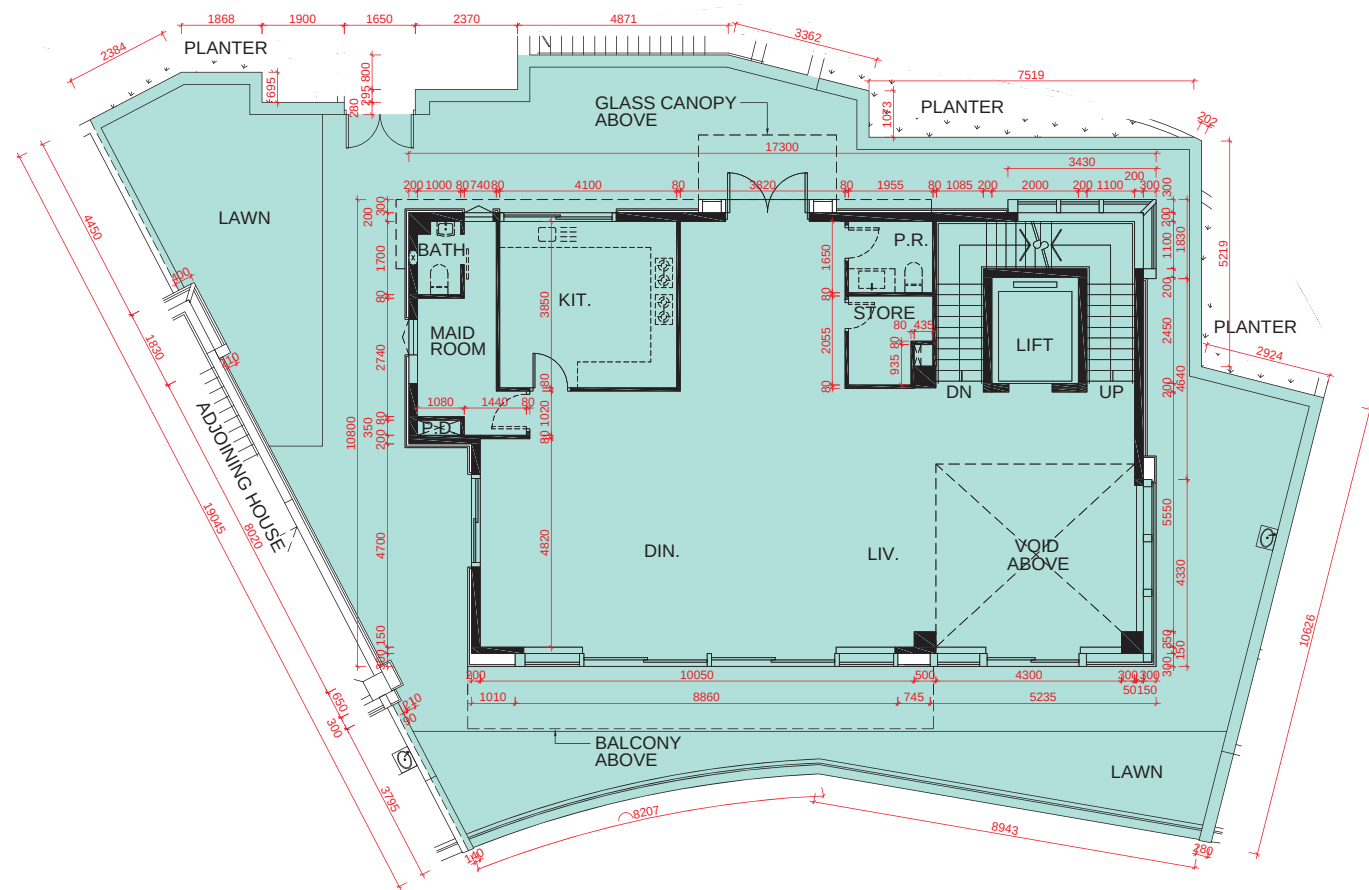
G/F PLAN 地面層平面圖
