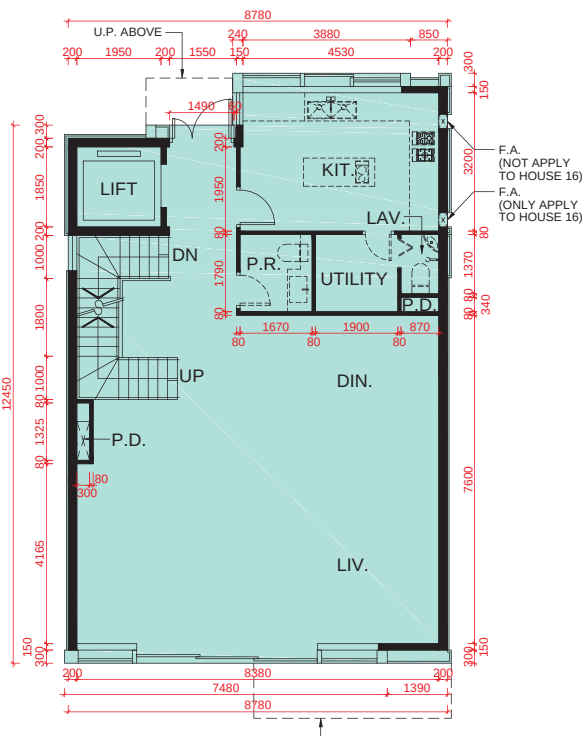
G/F PLAN 地面層平面圖
