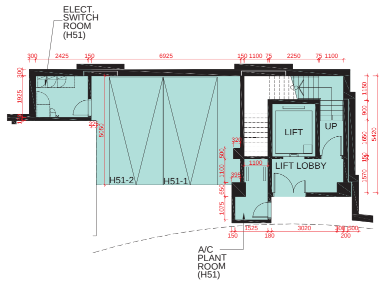
B/F PLAN 地庫層平面圖
