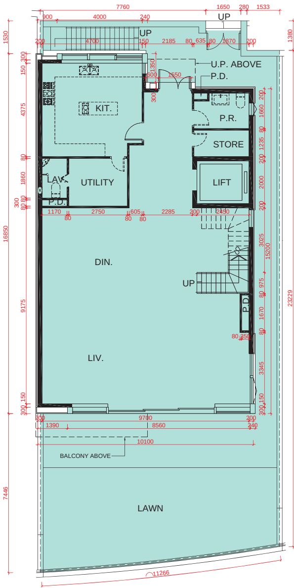
G/F PLAN 地面層平面圖
