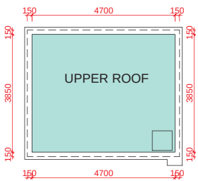
UPPER ROOF PLAN 上層天台平面圖
