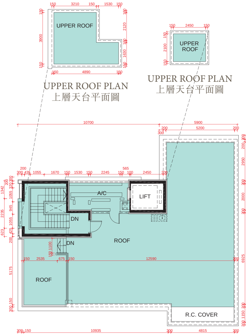
ROOF PLAN 天台平面圖
