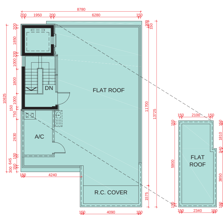
ROOF PLAN 天台平面圖
