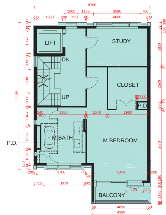
2/F PLAN 2樓平面圖
