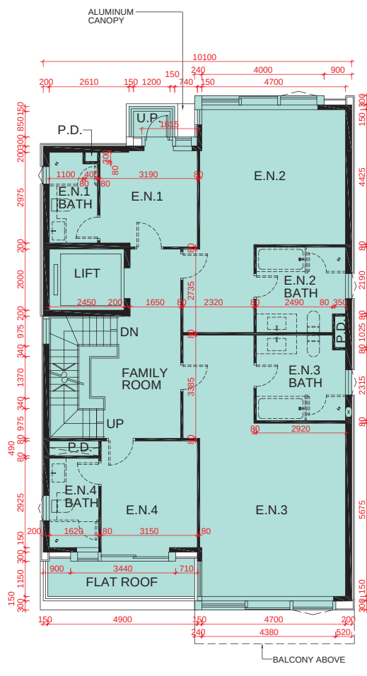
1/F PLAN 1樓平面圖
