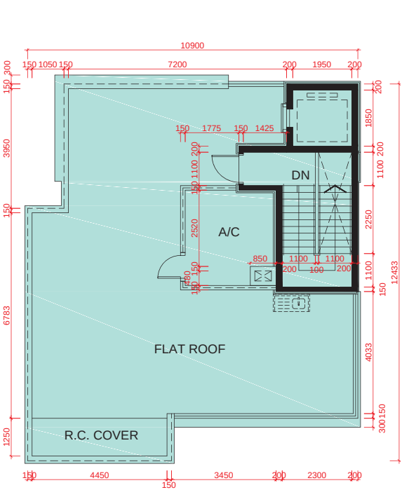
ROOF PLAN 天台平面圖
