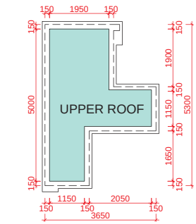
UPPER ROOF PLAN 上層天台平面圖
