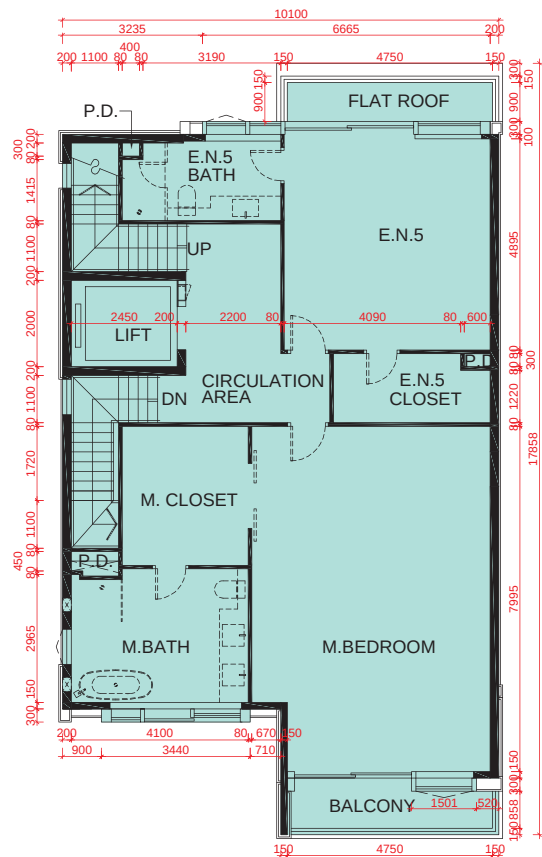
2/F PLAN 2樓平面圖
