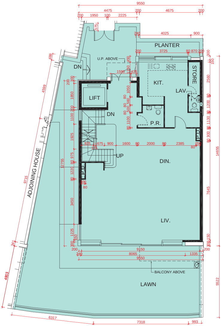
G/F PLAN 地面層平面圖
