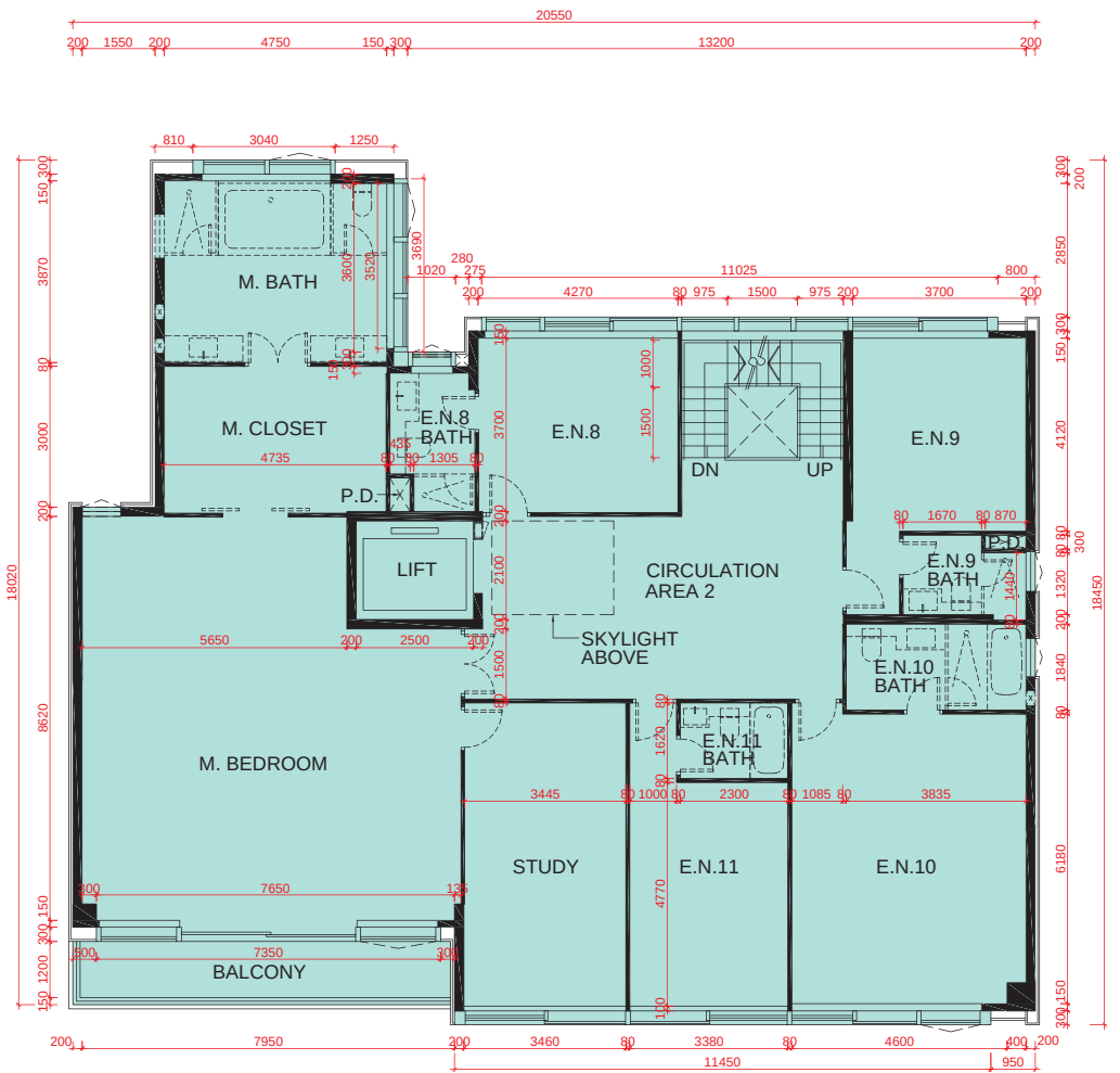
2/F PLAN 2樓平面圖
