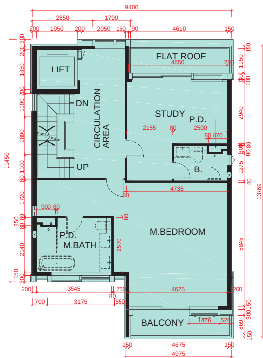
2/F PLAN 2樓平面圖
