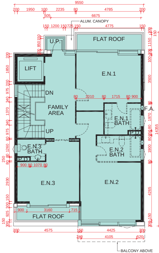
1/F PLAN 1樓平面圖
