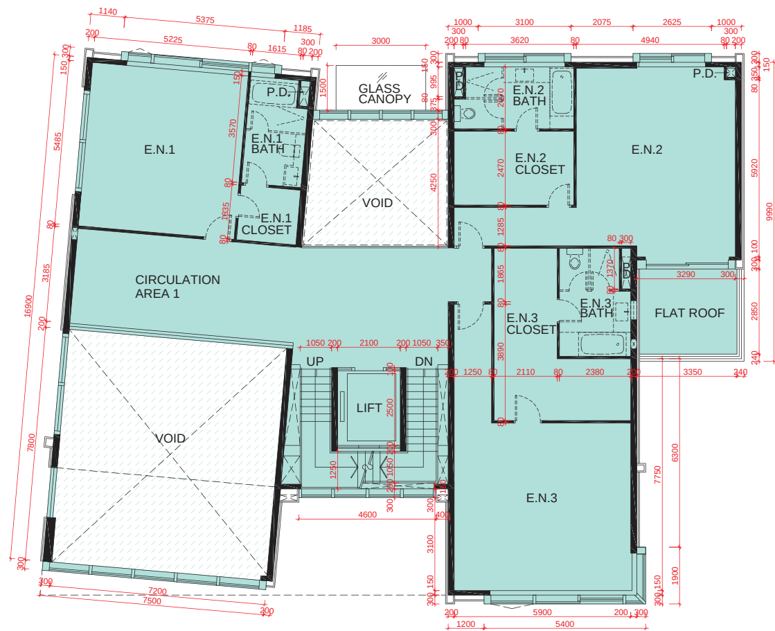
1/F PLAN 1樓平面圖
