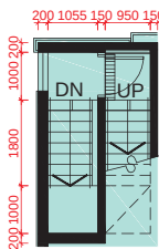
STAIRHOOD PLAN 梯屋平面圖
