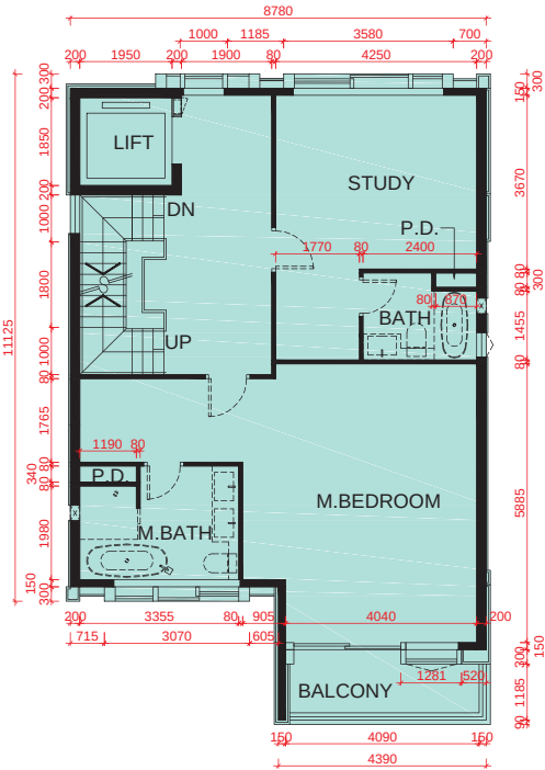
2/F PLAN 2樓平面圖
