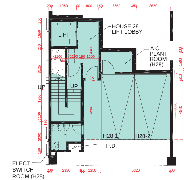
B/F PLAN 地庫層平面圖
