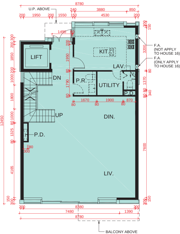
G/F PLAN 地面層平面圖
