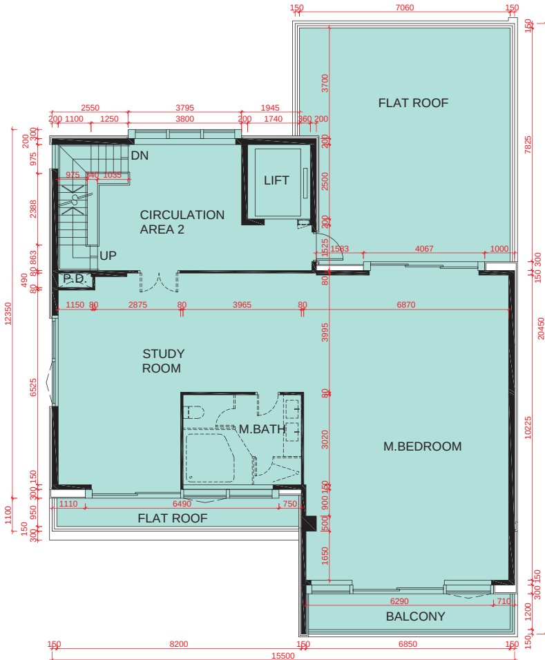
2/F PLAN 2樓平面圖
