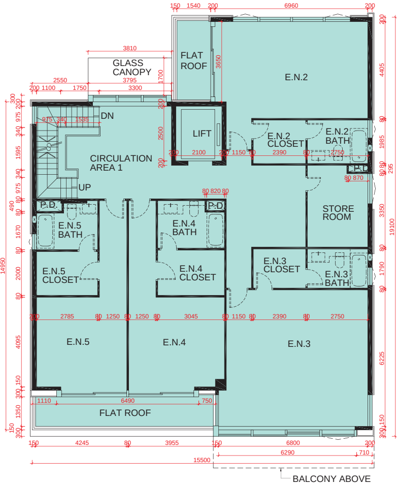
1/F PLAN 1樓平面圖
