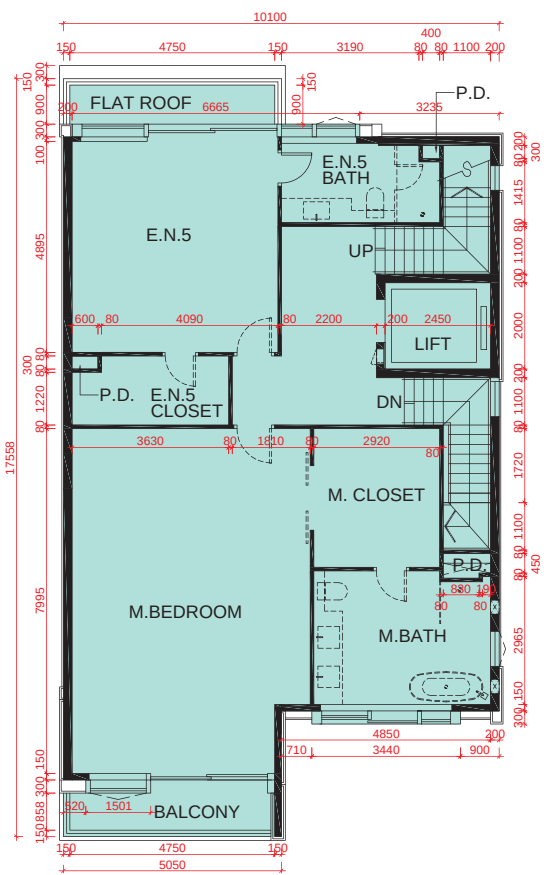
2/F PLAN 2樓平面圖
