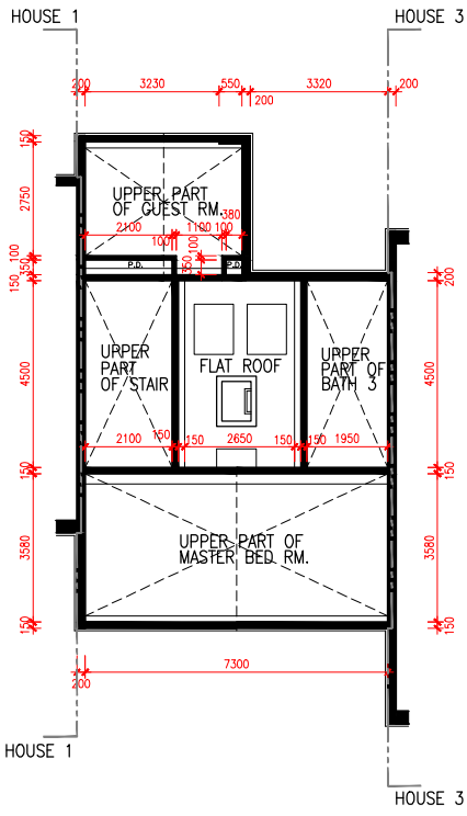
R/F PLAN
