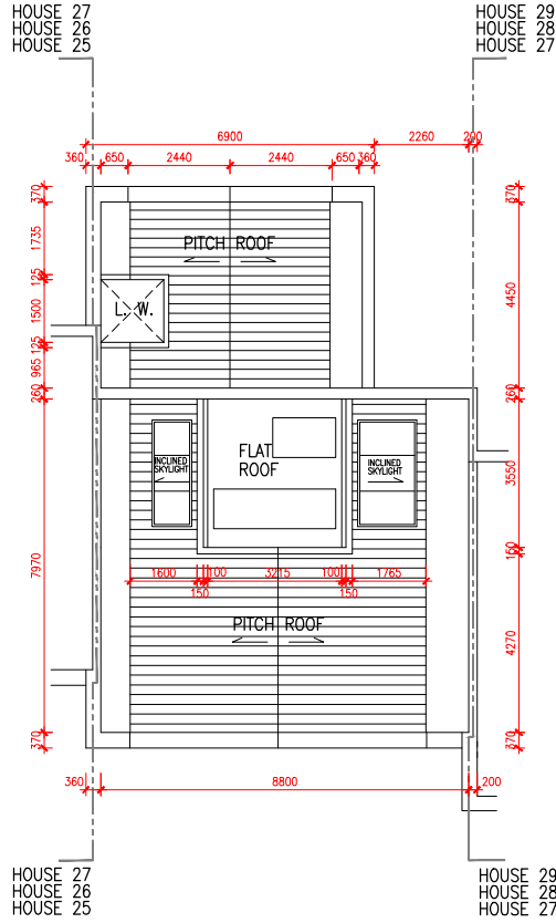
UR/F PLAN 上層天台平面圖
