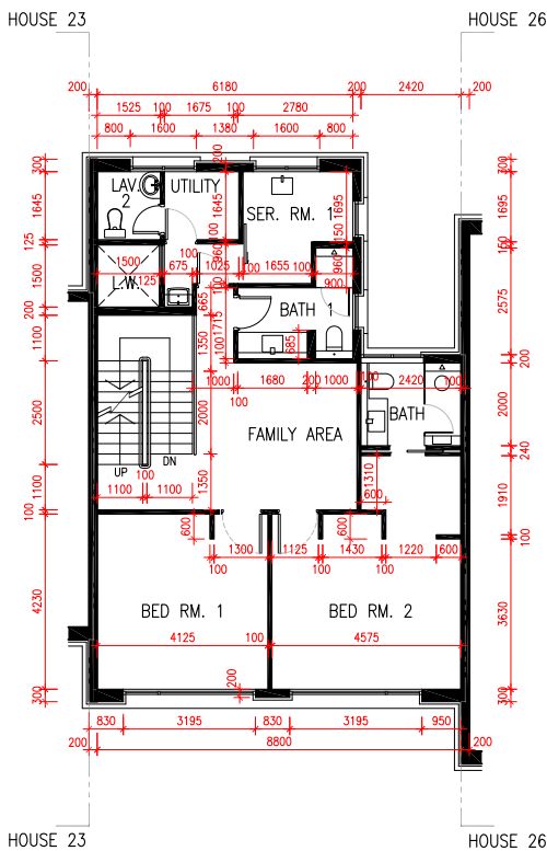
1/F AS-IS PLAN 1樓現狀平面圖
