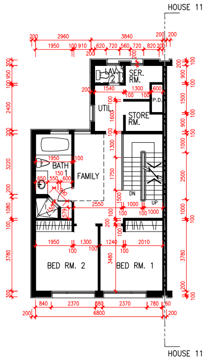
1/F PLAN 1樓平面圖
