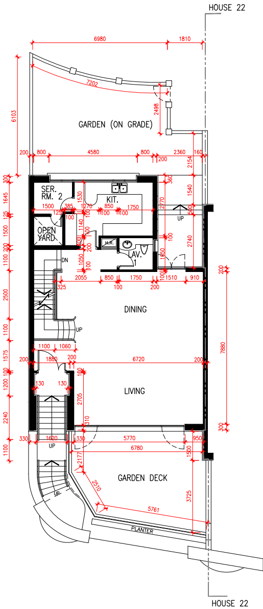
G/F PLAN 地下層平面圖
