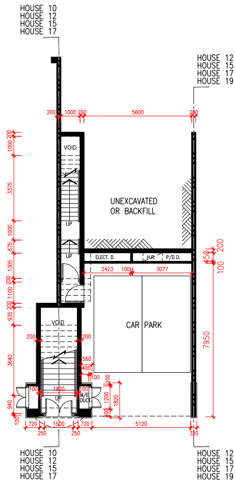
LG/F PLAN 低層地下平面圖
