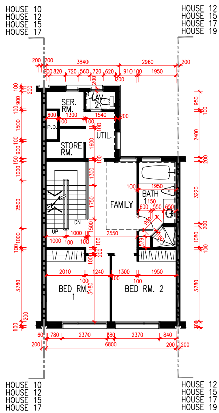
1/F PLAN 1樓平面圖
