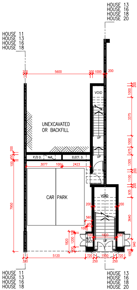
LG/F PLAN 低層地下平面圖
