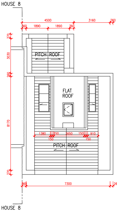
UR/F PLAN
