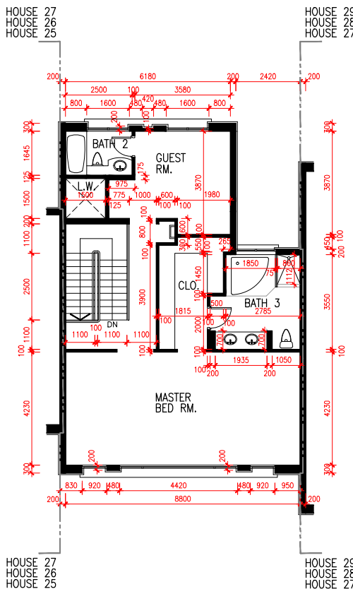
2/F PLAN 2樓平面圖
