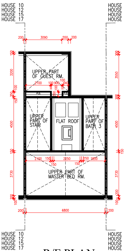
R/F PLAN 天台平面圖
