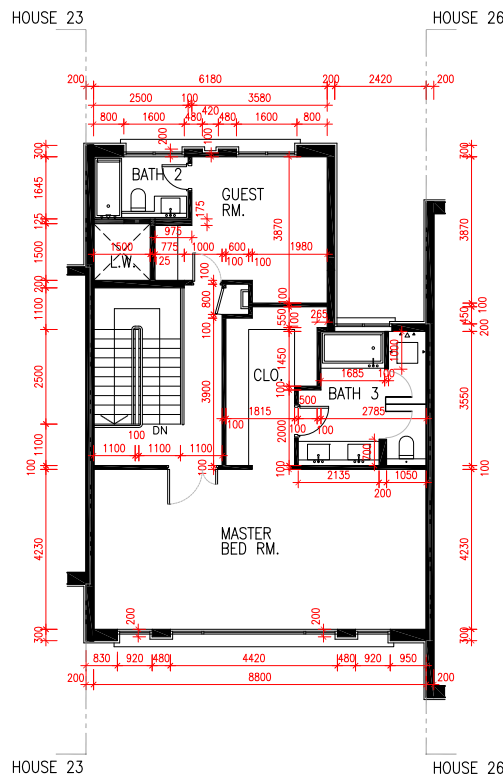
2/F AS-IS PLAN 2樓現狀平面圖
