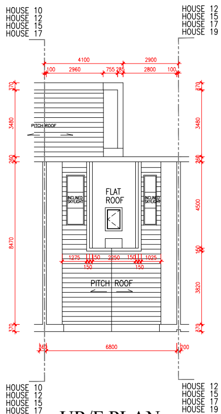
UR/F PLAN 上層天台平面圖
