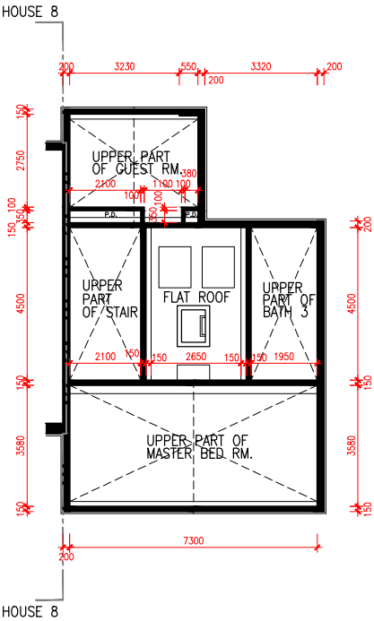
R/F PLAN
