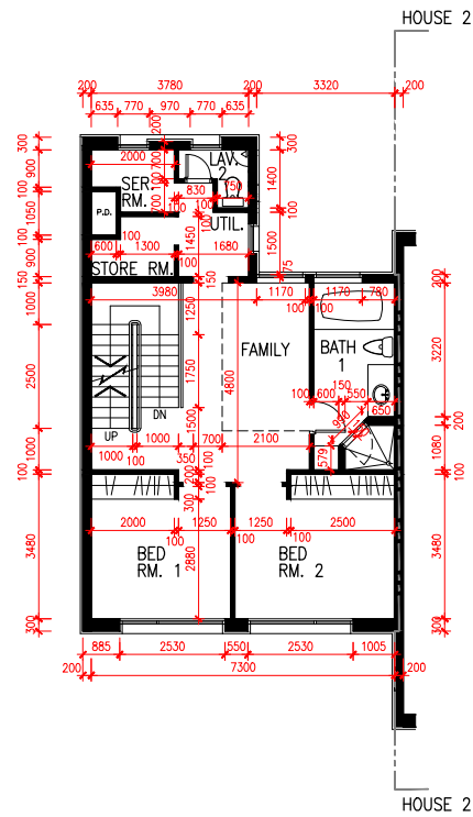
1/F PLAN 1樓平面圖
