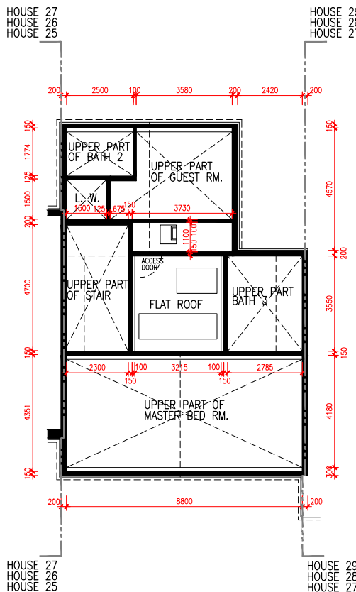
R/F PLAN 天台平面圖
