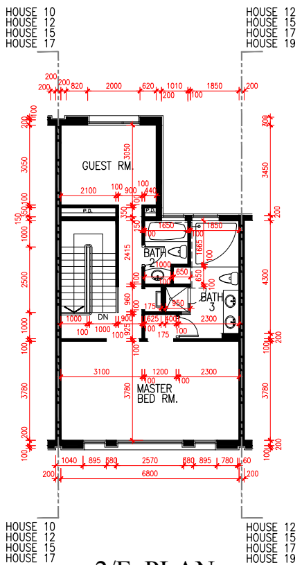
2/F PLAN 2樓平面圖
