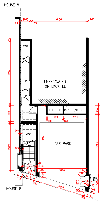
LG/F PLAN 低層地下平面圖
