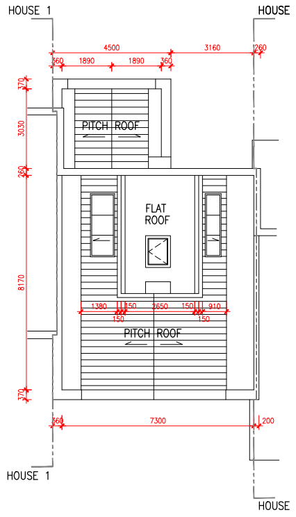
UR/F PLAN
