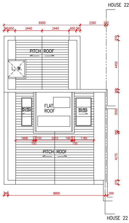
UR/F PLAN 上層天台平面圖
