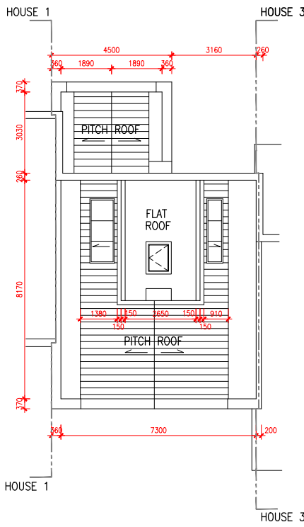
UR/F PLAN
