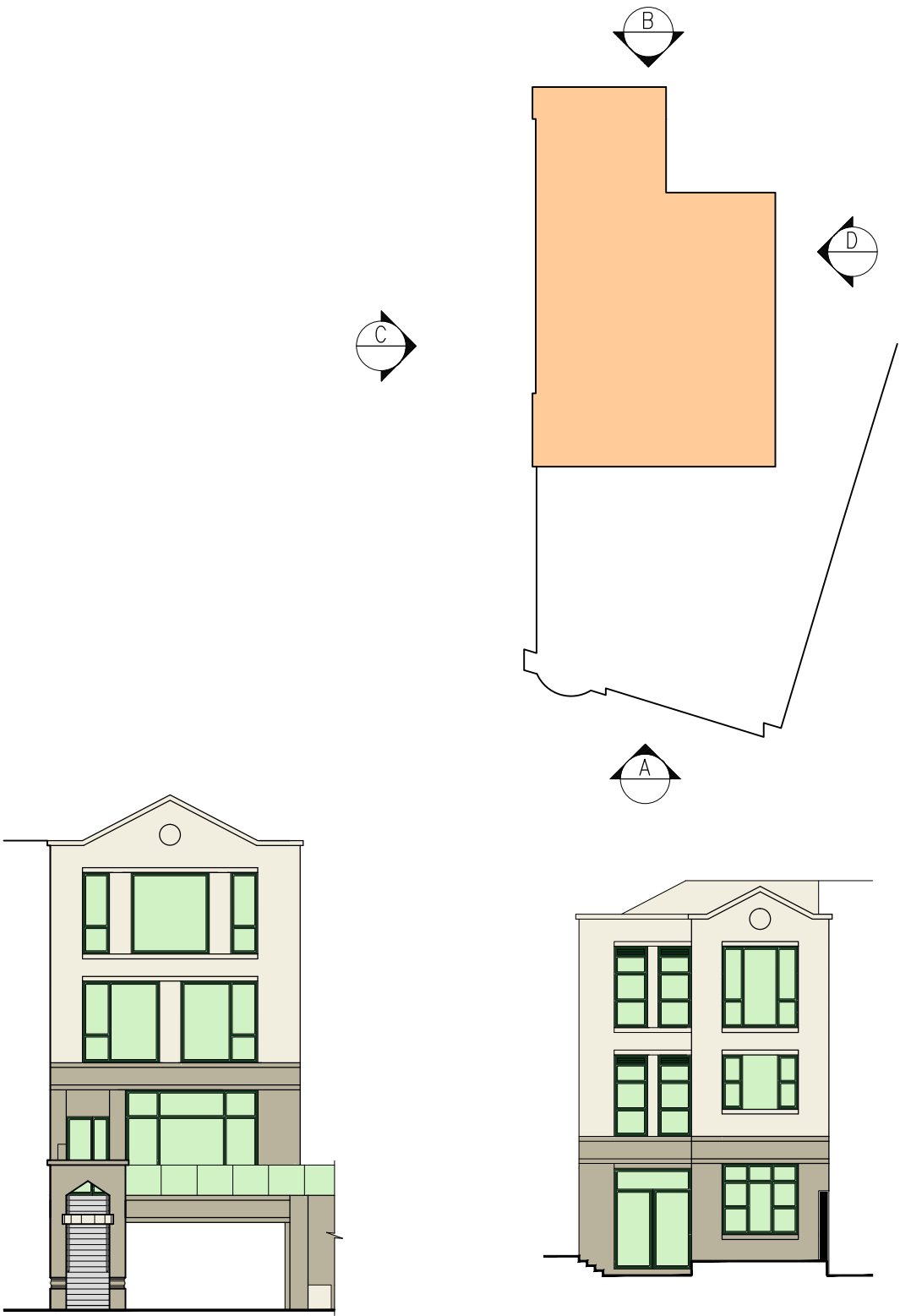
ELEVATION A 立面圖 A
