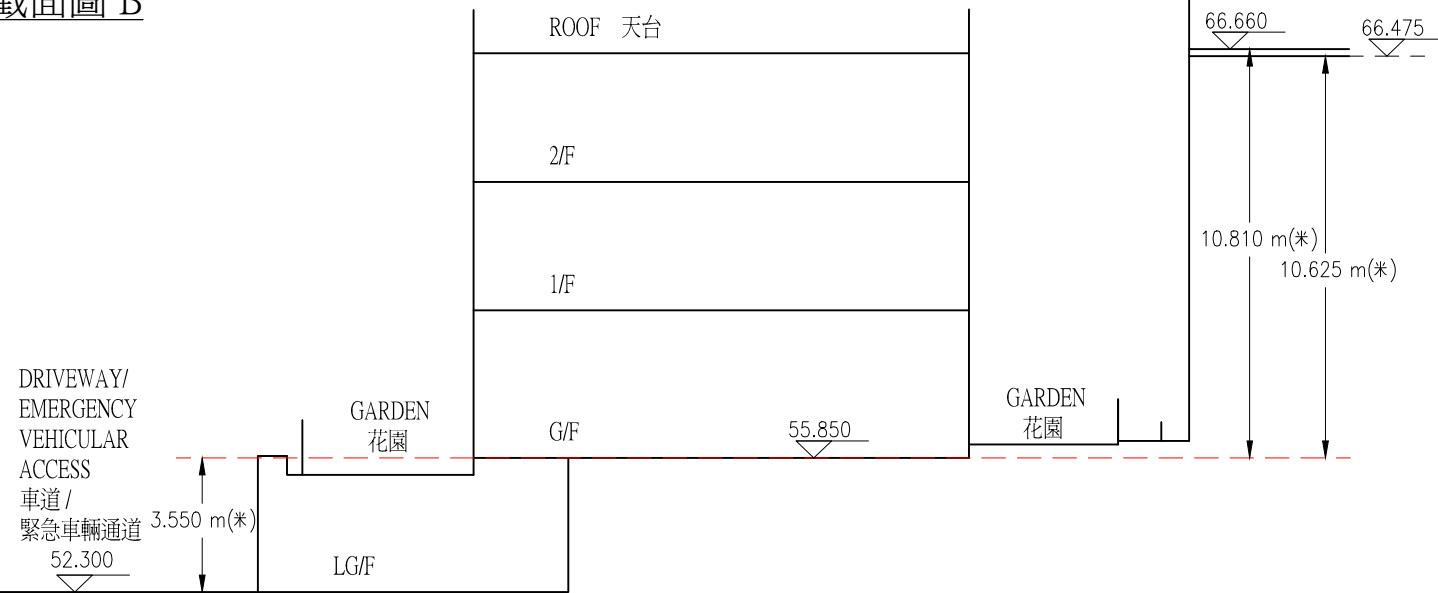
CROSS - SECTION PLAN B 橫截面圖 B
