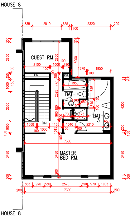
2/F PLAN 2樓平面圖
