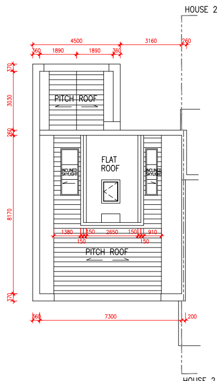
UR/F PLAN
