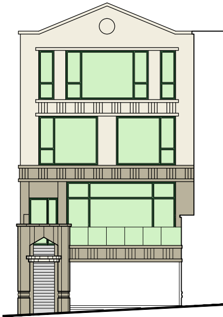
ELEVATION A 立面圖 A
