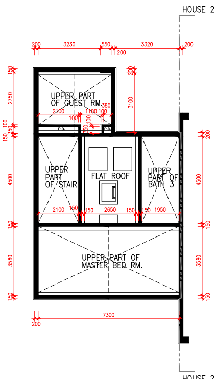
R/F PLAN
