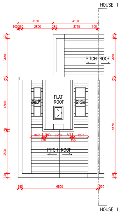
UR/F PLAN
