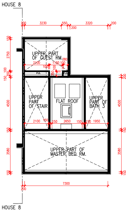
R/F PLAN 天台平面圖
