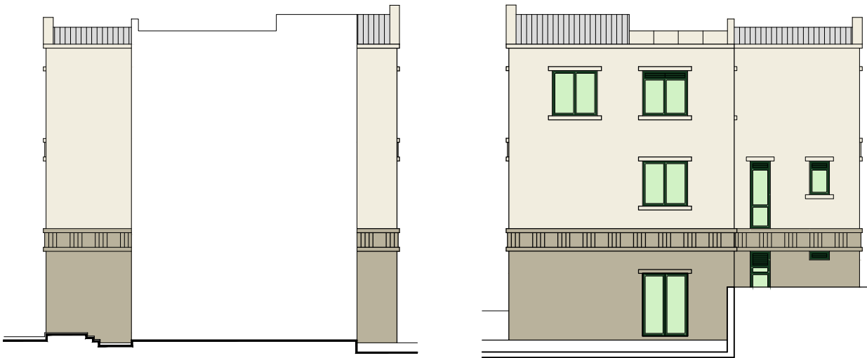
ELEVATION C 立面圖 C
