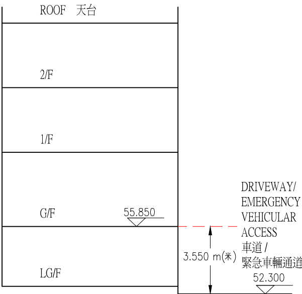
CROSS - SECTION PLAN B 橫截面圖 B
