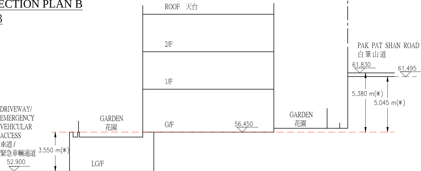
橫截面圖 B
