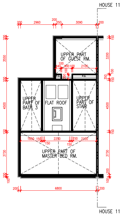
R/F PLAN
