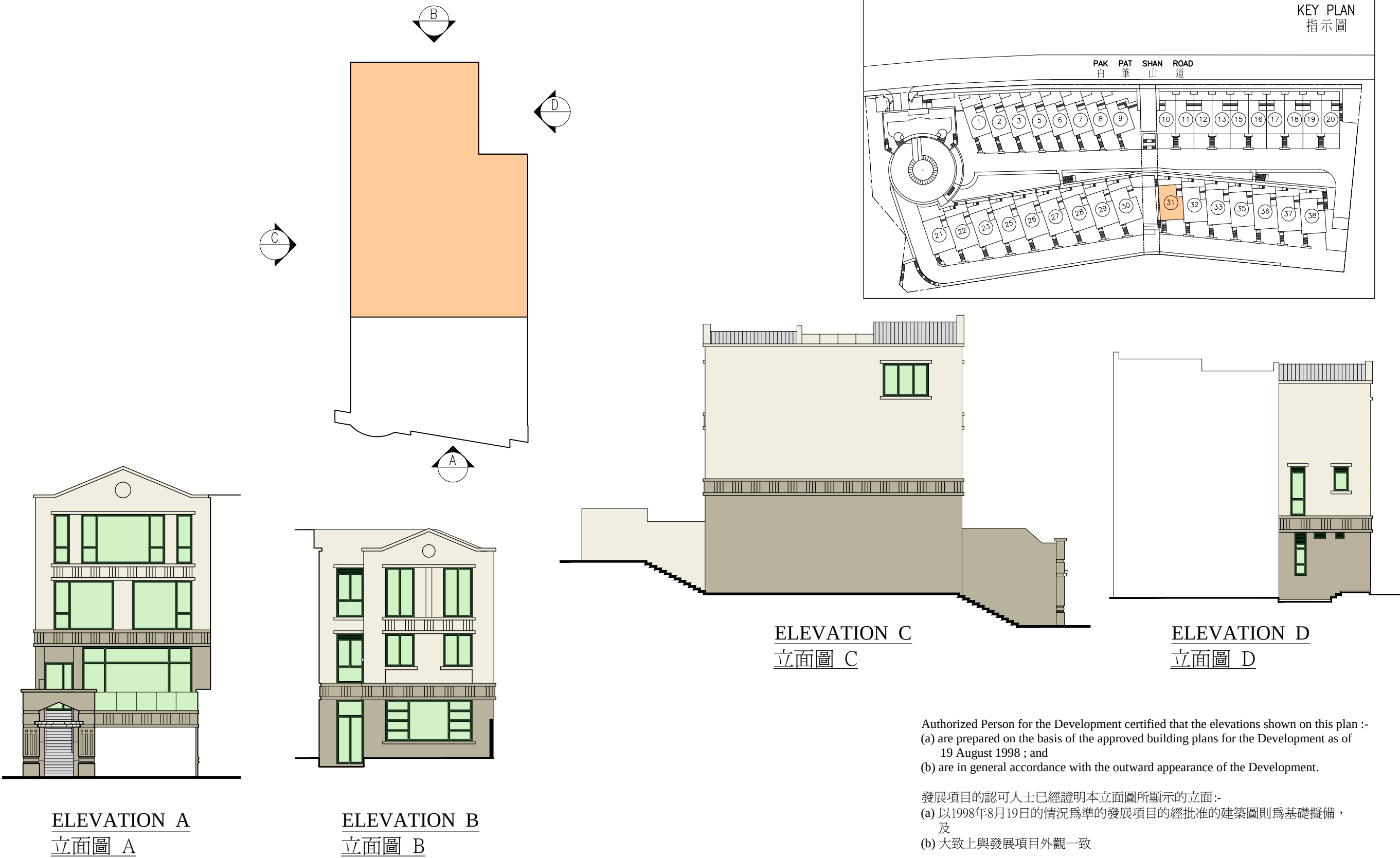
HOUSE 31 ELEVATION PLAN 31號洋房 立面圖
