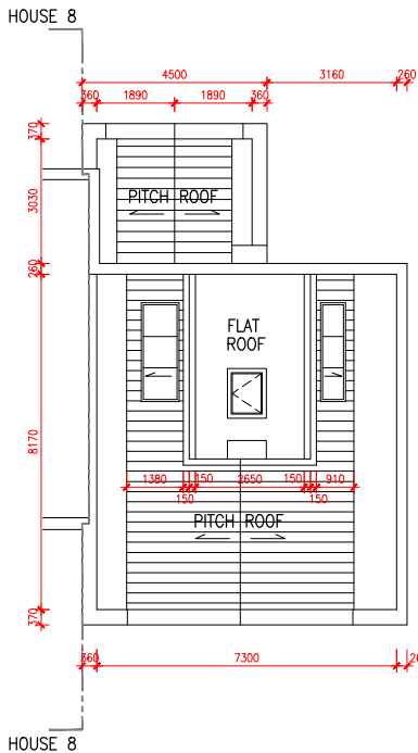
UR/F PLAN 上層天台平面圖
