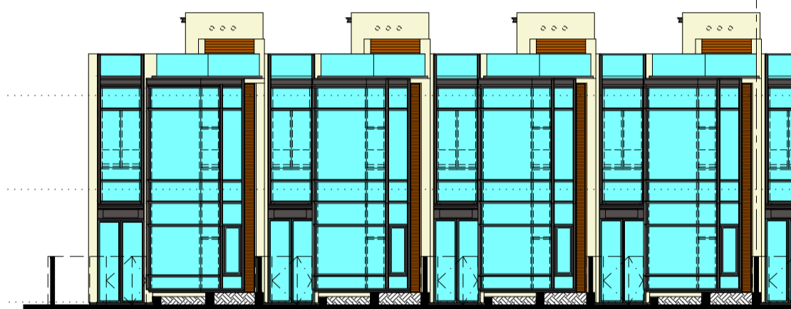
Elevation Plan D1 立面圖 D1
