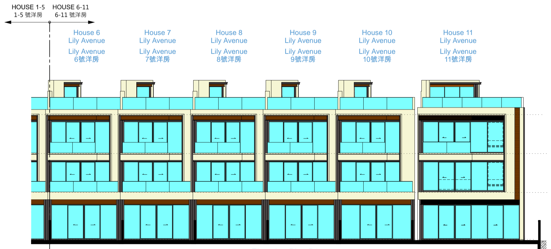
Elevation Plan B2 立面圖 B2
