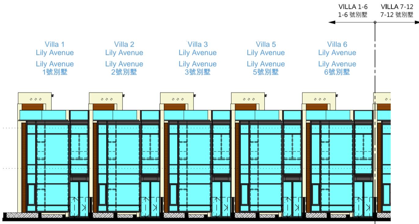
Elevation Plan C1 立面圖 C1
