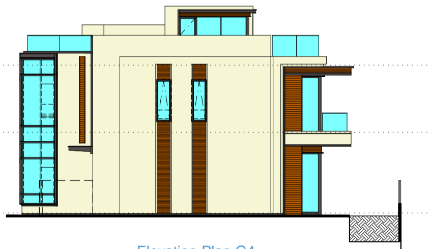
Elevation Plan G4 立面圖 G4
