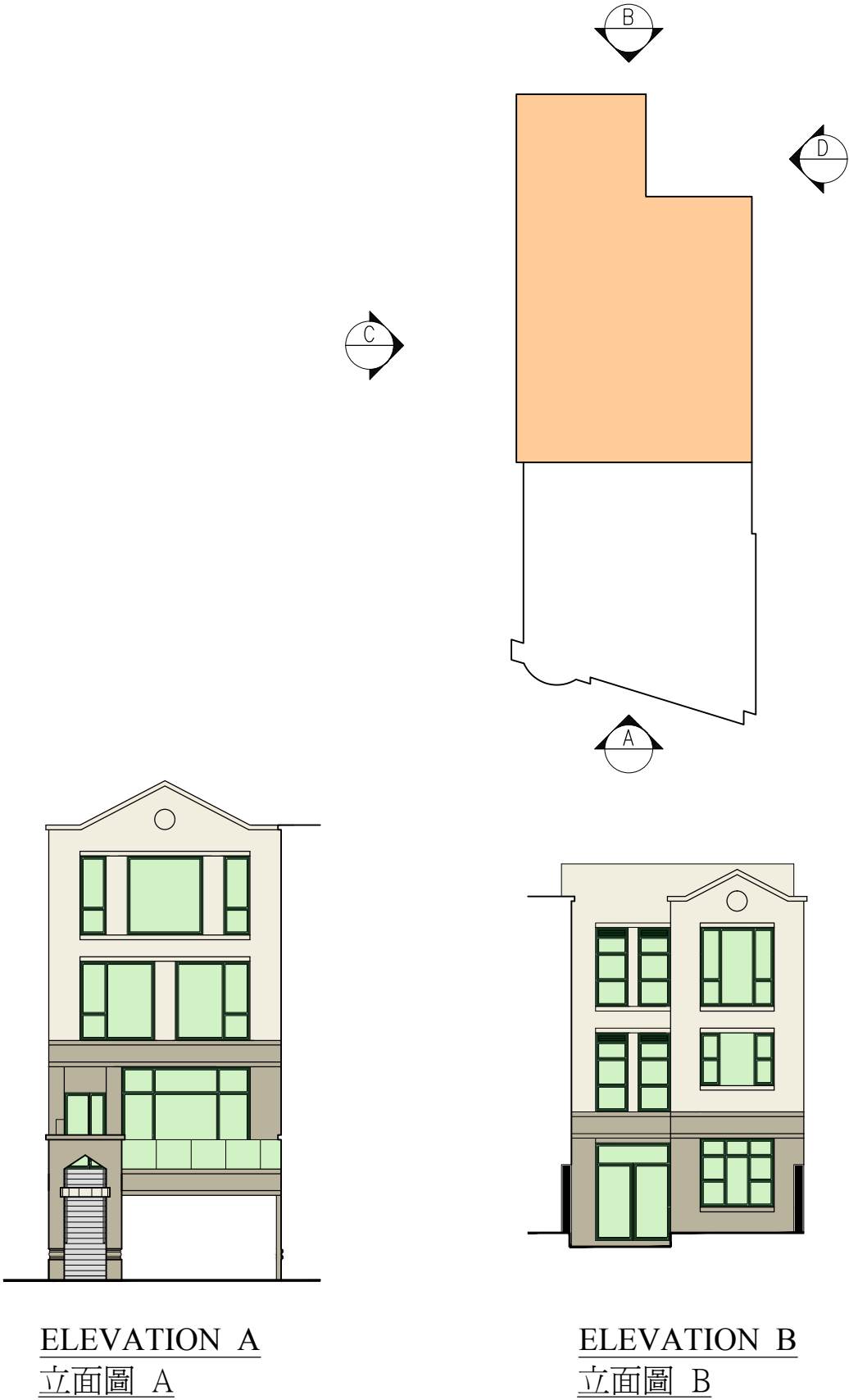
HOUSE 1 ELEVATION PLAN 1號洋房 立面圖
