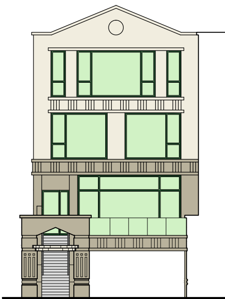
ELEVATION A 立面圖 A
