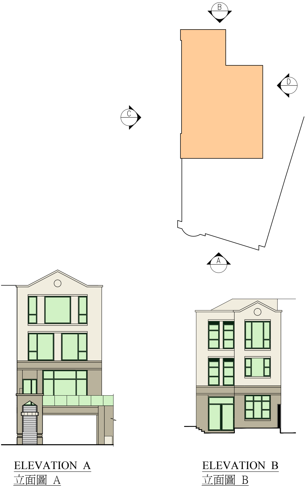
HOUSE 9 ELEVATION PLAN 9號洋房 立面圖
