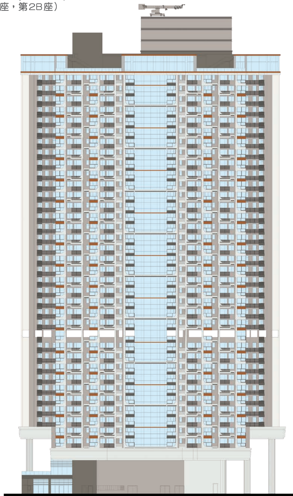
Elevation Plan 3 - Tower 2 (Tower 2A, Tower 2B) 立面圖3 - 第2座(第2A座, 第2B座)
